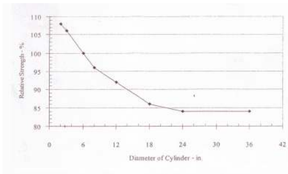
รูปที่ 4.2 ค่าเปรียบเทียบกำลังอัดรูปทรงกระบอกมาตรฐาน
