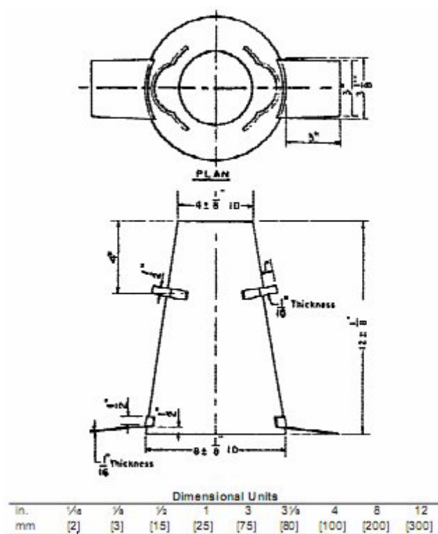
รูปที่ ๑ รูปร่างและมิติของกรวยทดสอบค่ายุบตัว
