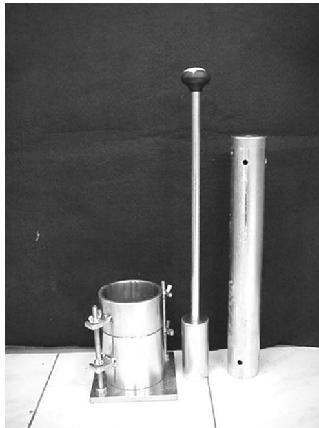
รูปที่ ๓ แบบเหล็ก และ ค้อน
