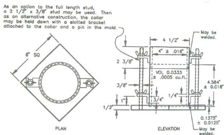
รูปที่ ๑ แบบเหล็ก ๔ นิ้ว
