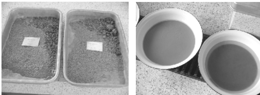
รูปที่ ๔ ตัวอย่างส่วนที่ค้ำตะแกรงเบอร์ ๒๐๐รูปที่ ๕ ตัวอย่างส่วนที่ผ่านตะแกรงเบอร์ ๒๐๐ สำหรับการร่อนผ่านตะแกรงสำหรับการทดสอบขนาดผลโดยไฮโดรมิเตอร์
