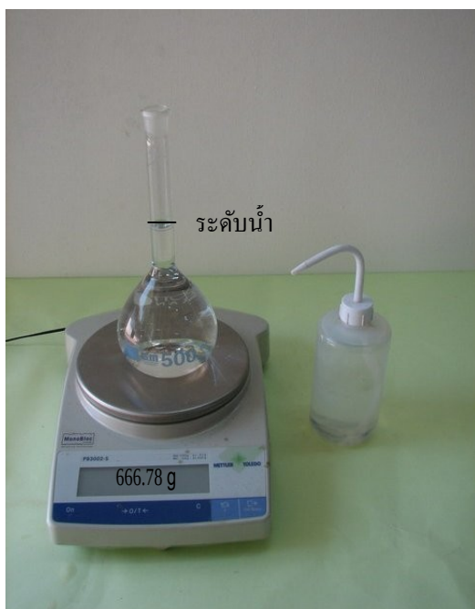
รูปผนวกที่ ๑ ชั่งน้ำหนักขวด Pycnometer และน้ำ
