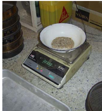
๑.๔ ชั่งน้ำหนักตัวอย่างที่ค้ำตะแกรง
