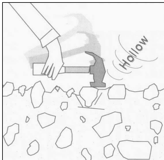
รูปที่ ผ3-3 การตรวจสอบเบื้องต้นหลังจากการสกัดคอนกรีตที่เสียหายออก (ที่มา: Concrete Repair and Maintenance Illustrated) (ข้อ ผ3.3)
