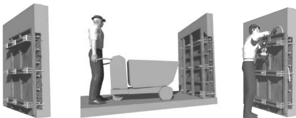
รูปที่ 52 วิธีการซ่อมแซมโดยวิธีการเทด้วยคอนกรีตธรรมดา (ที่มา: ACI-RAP 4)
