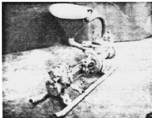
รูปที่ ผ4-5 เครื่องสูบบแบบ Simplex Pump (ที่มา: EM 1110-1-3500)
