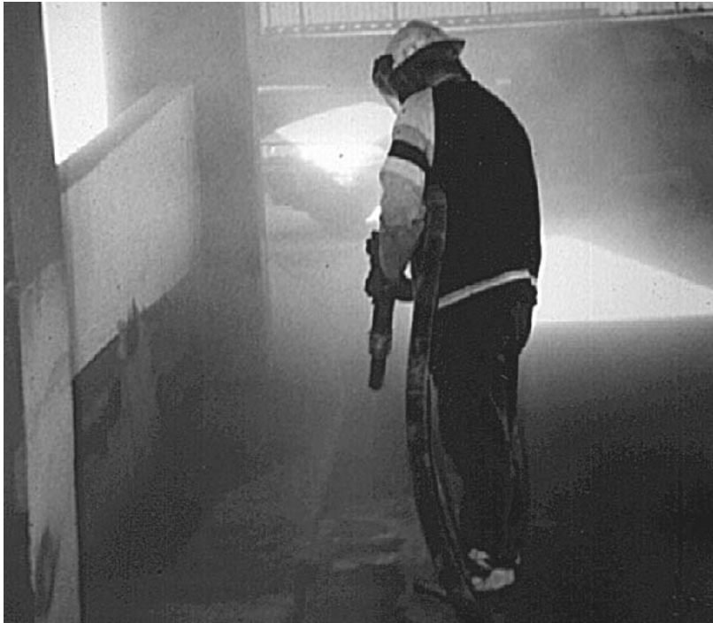
รูปที่ 10 Abrasive Sand Blasting (ที่มา: ICRI 03732)
