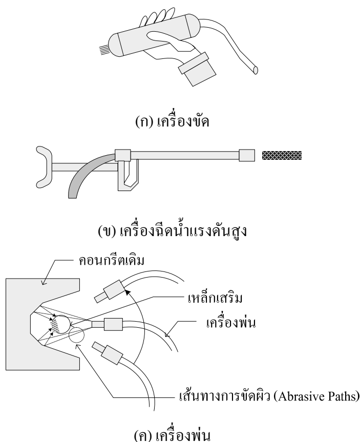
รูปที่ 17 เครื่องมือที่นิยมใช้ในการทำความสะอาดเหล็กเสริม
