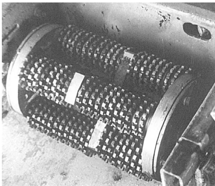
รูปที่ 14 Scrifier (ที่มา: ICRI 03732)
