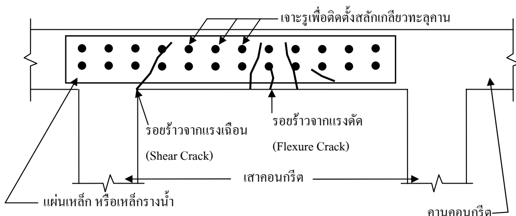
รูปที่ ผ2-4 การติดตั้งแผ่นเหล็กปะกับภายนอกเพื่อเพิ่มกำลังรับน้ำหนักของคาน คสล. (ที่มา: ACI 546)
