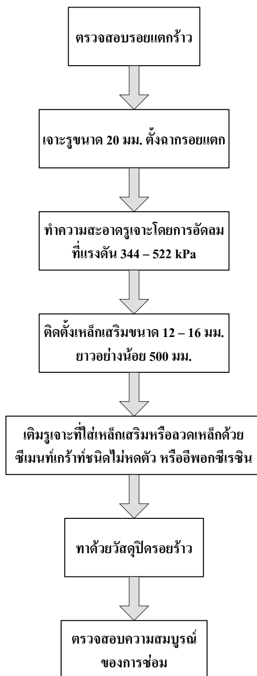
รูปที่ 57 วิธีการซ่อมแซมโดยใส่เหล็กเสริมเพิ่มเติม (ข้อ 7.10, 7.10.3.5)
