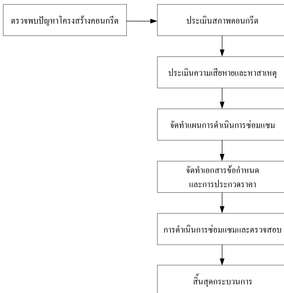
รูปที่ ผ5-1 กระบวนการซ่อมแซมโครงสร้างคอนกรีต (ข้อ ผ5)
