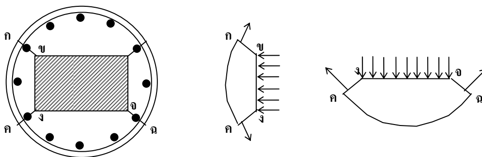
รูปที่ ผ2-5 การเสริมกำลังแบบใส่ปลอก
