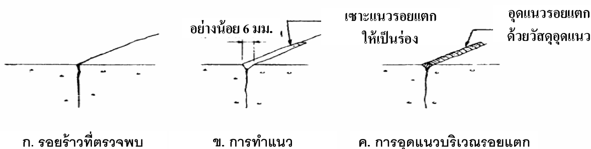
รูปที่ 46 วิธีการซ่อมแซมแบบทำแนวและอุดแนวบริเวณรอยแตก (Routing และ Sealing) (ที่มา: EM 1110-2-2002) (ข้อ 7.4)
