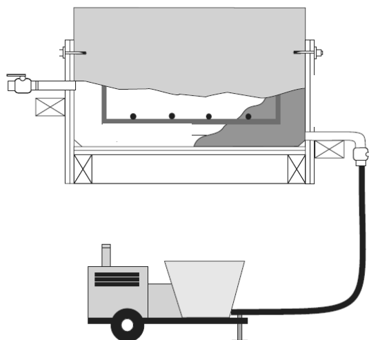
รูปที่ 27 การซ่อมแซมโดยตักแบบแล้วใช้เครื่องสูบลูกกรวดเข้าไป (ที่มา: ICRI 03731) (ข้อ 5.6.2)
