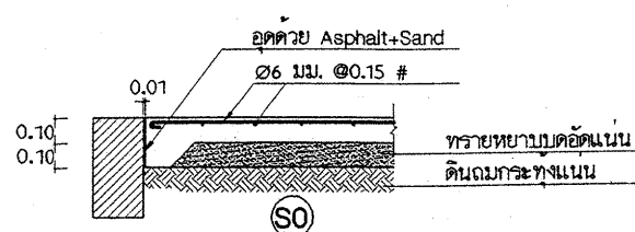
แบบขยาย SO
