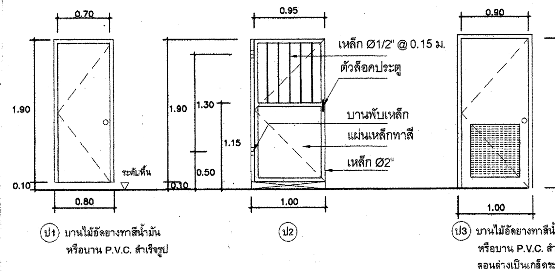
แบบขยายประตู
