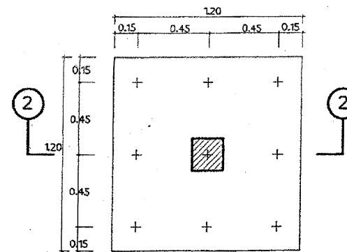
F2 1:25
