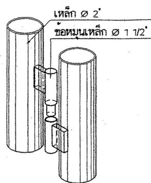
แบบขยายข้อประตุมุม
