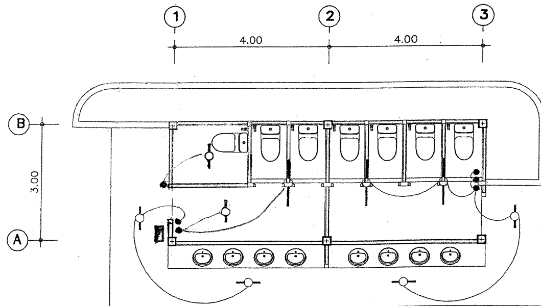
แปลนไฟฟ้า
