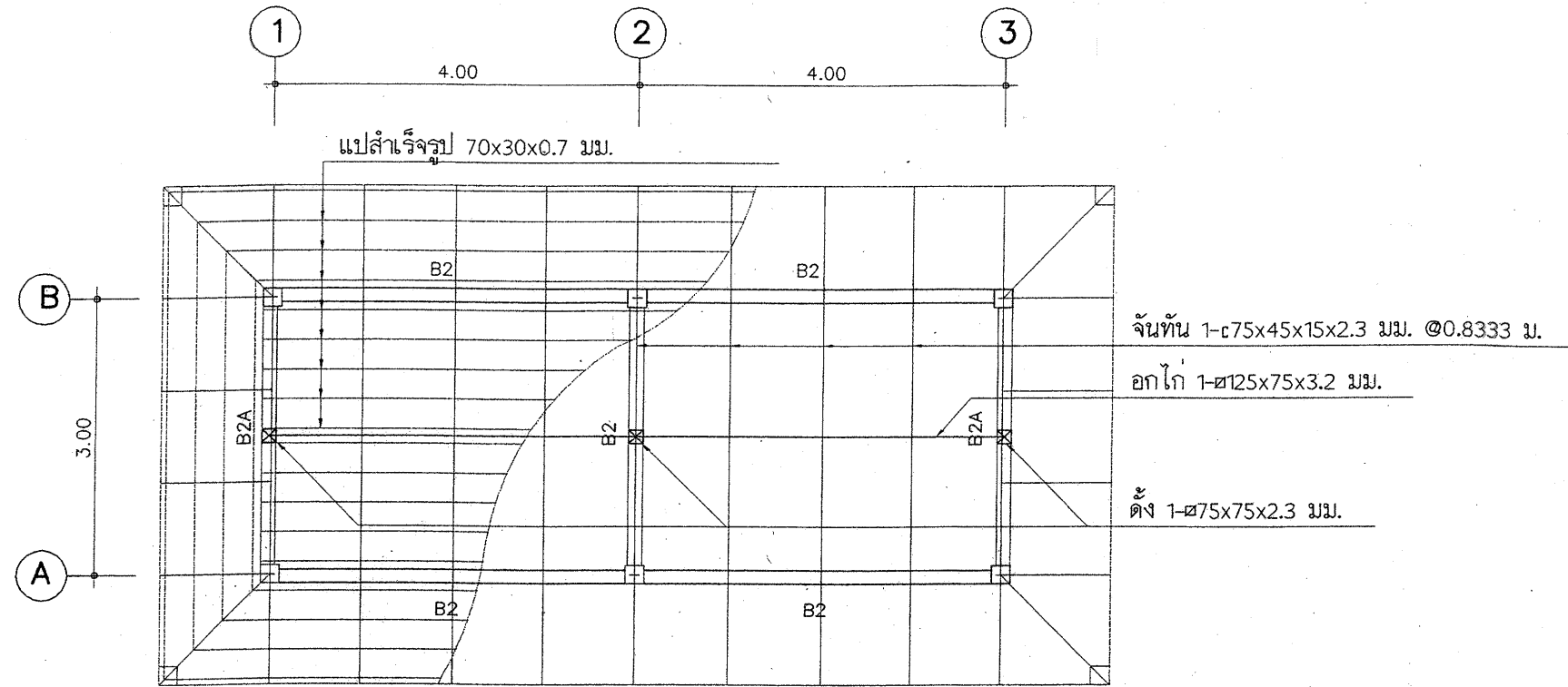
แปลนคาน และโครงสร้างหลังคา
