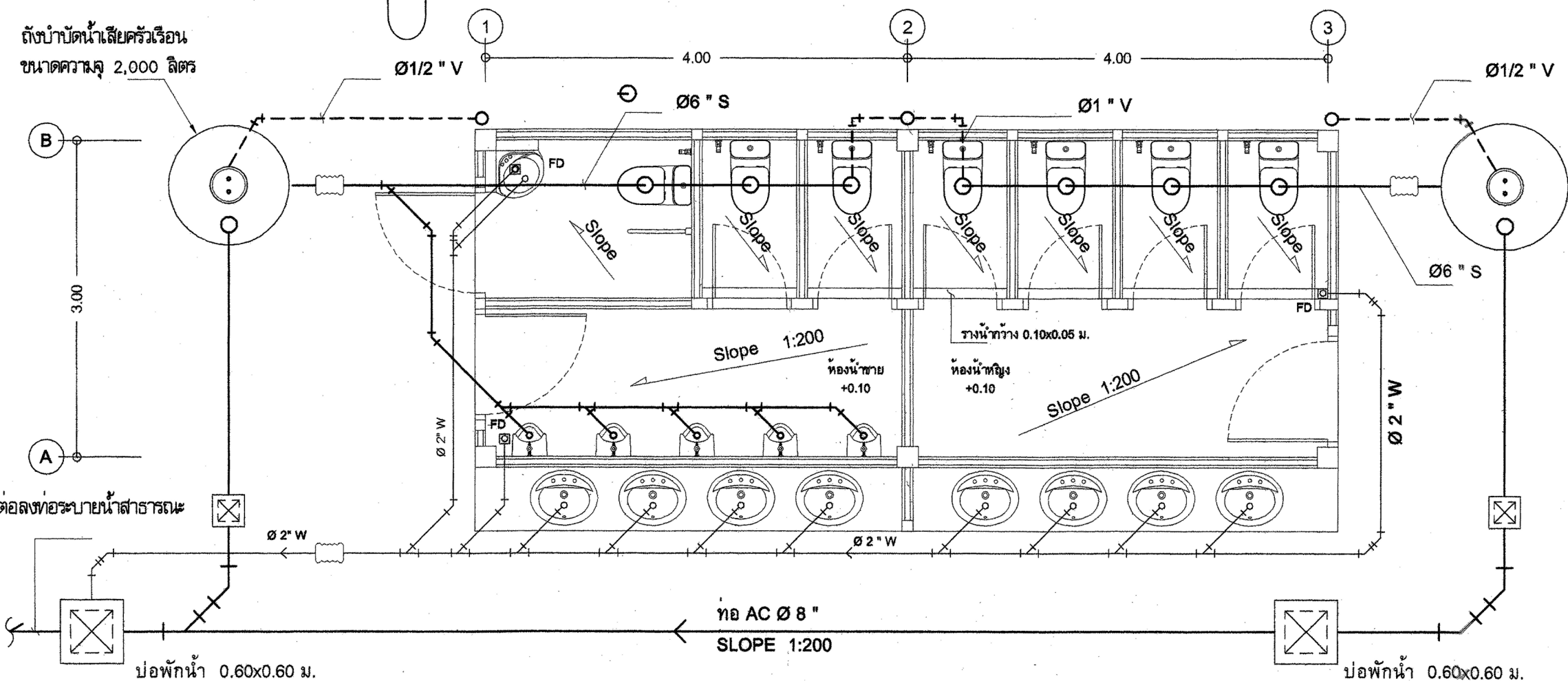
แปลนท่อน้ำทิ้ง มาตราส่วน 1:50
