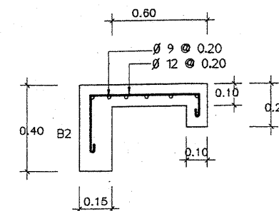
แบบขยายคานเดือร
