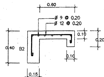
แบบขยายคานเดือร
