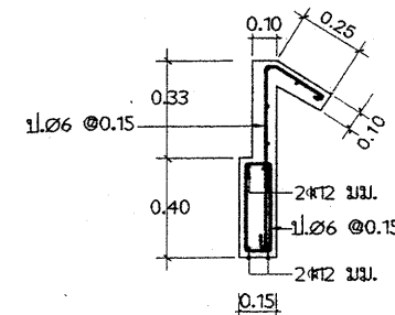
B2A 1:25
