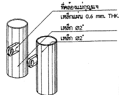
แบบขยายตัวล็อคประตู
