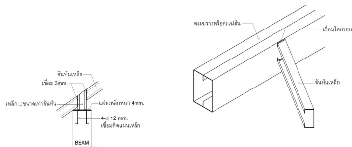
การยึดจันทันกับคาน ค.ส.ล.
