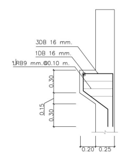
แบบขยายโครงถัก T-1 มาตราส่วน 1:25 แบบขยายการเสริมเหล็กหูช้าง มาตราส่วน 1:25
