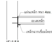
การยึดอะเสกับเสา ค.ส.ล.
