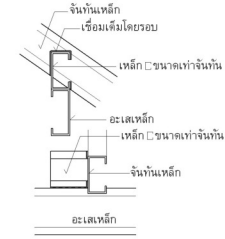
การเชื่อมจันทันกับอะเส
