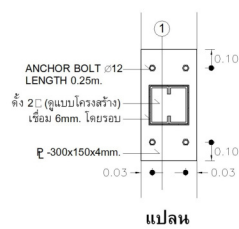
แบบขยายการติดตั้งบนคาน ค.ส.ล.
