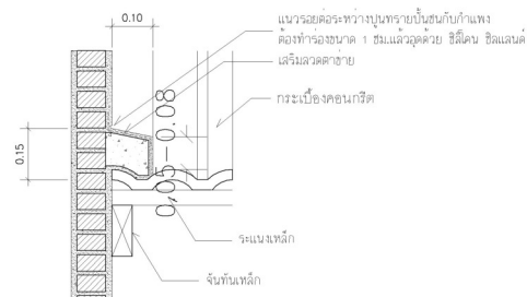
แบบขยายการทำปูนปั้นชนผนัง 1 : 10
