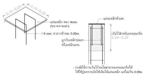
แบบขยายแผ่นเหล็กวางบนหัวเสา
