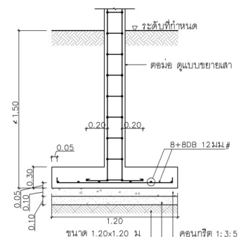
F2 1: 25
