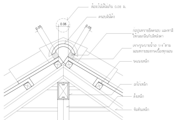
แบบขยายครอปสัน 1 : 10
