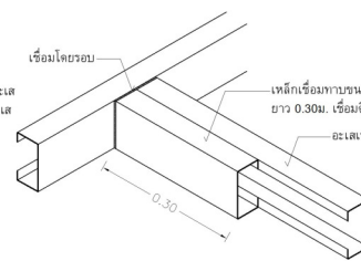
แบบขยายโครงสร้างทั่วไป
