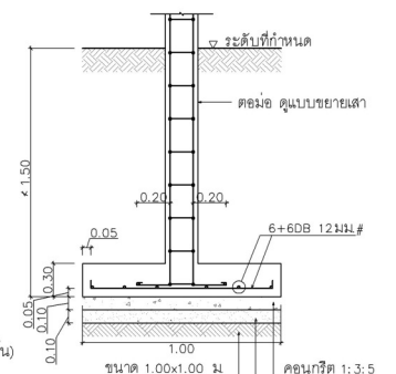
F1 1: 25
