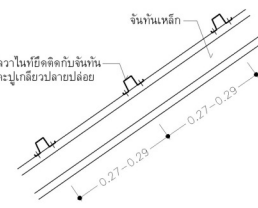
การติดตั้งแป
