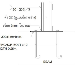
รูปตัด 1.
