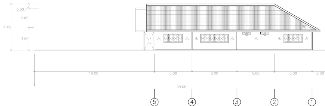
รูปด้าน B มาตราส่วน 1:150
