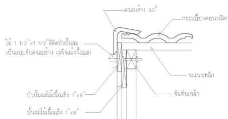
แบบขยายการติดตั้งครอปข้าง 90° 1 : 10
