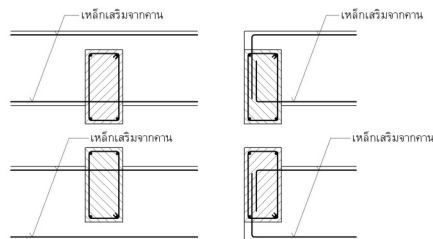
การเสริมเหล็กคานต่างระดับ
