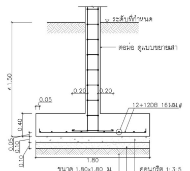
F4 1: 25
