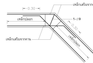
ผังขยายเหล็กในคานหักมุม
