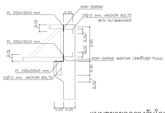
แบบขยายจุดรองรับโครงถัก T-1 มาตราส่วน 1:25
