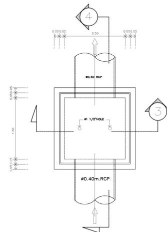
แปลนบ่อดักขยะ SCALE 1:10
