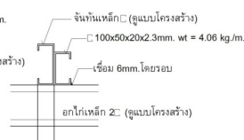
รูปตัด 2.
