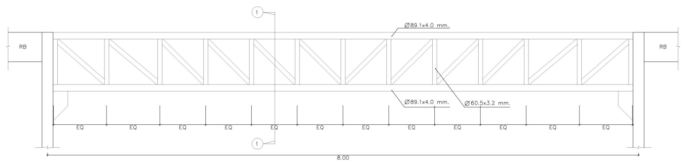
แบบขยายโครงถัก T-1 มาตราส่วน 1:25 แบบขยายการเสริมเหล็กหูช้าง มาตราส่วน 1:25
