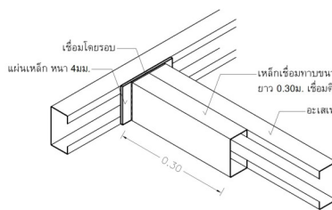
การเชื่อมอะเสเหล็ก
