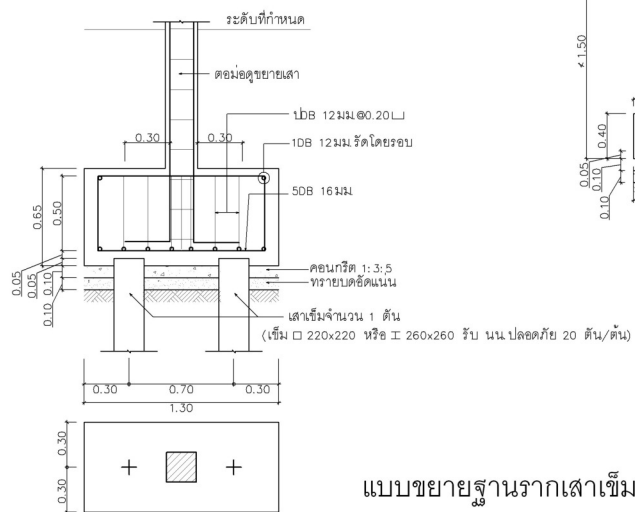
F2 1: 25
