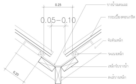
แบบขยายรางน้ำหลังคา 1 : 10
