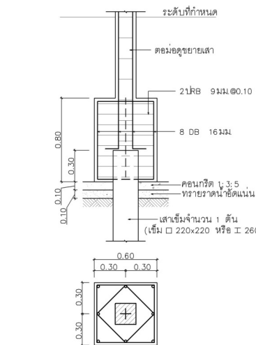
F1 1: 25
