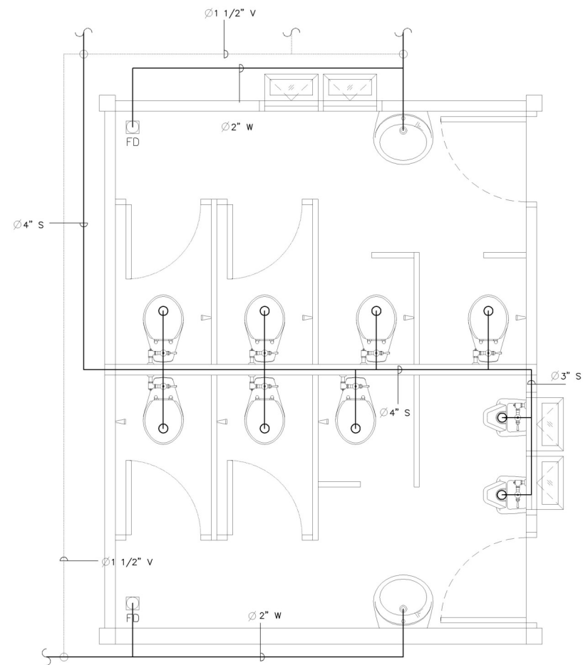
ห้องน้ำ 1 (น้ำเสีย)
