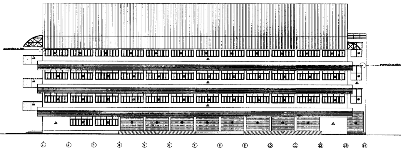
หน้าบ้าน (A) 1:100
