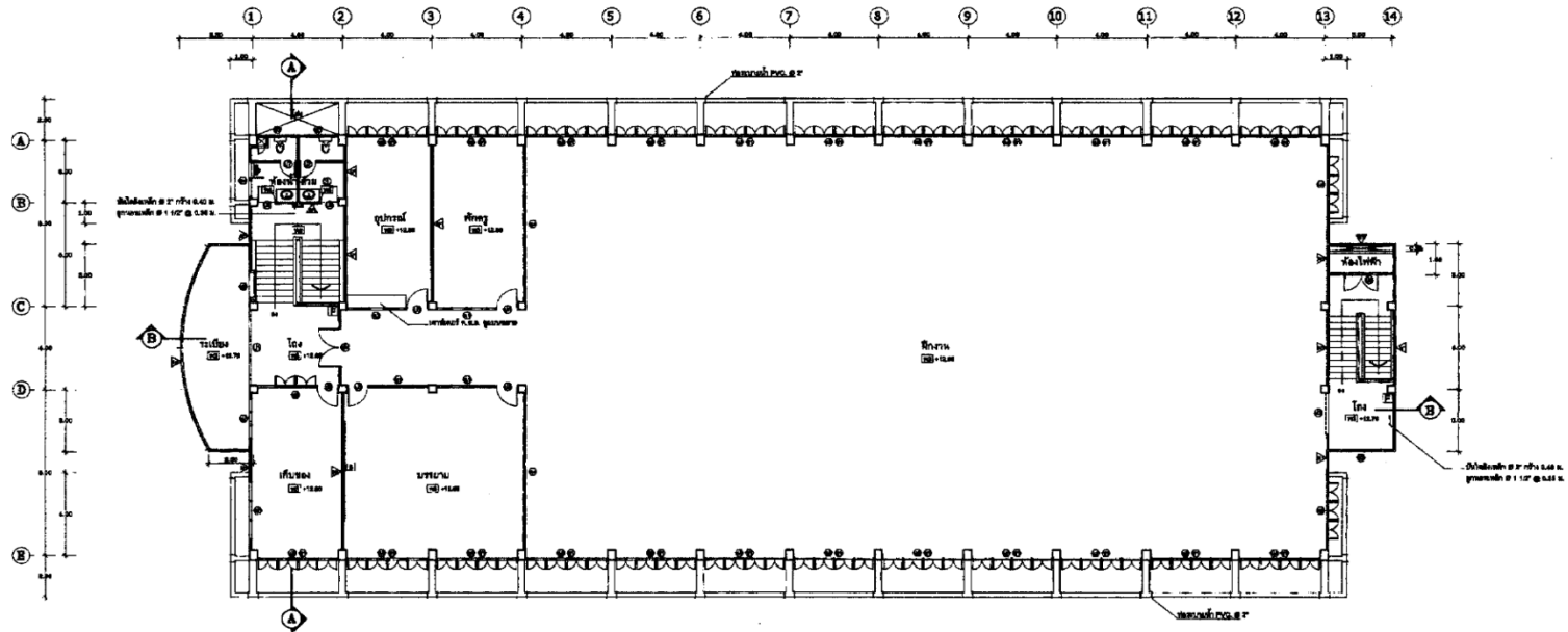
แปลนพื้นที่ 4 1:100
