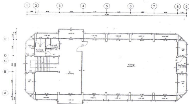
แปลนพื้นชั้นบน 1:100
