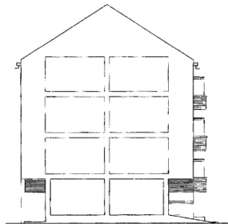
รูปด้าน 2 SCALE 1 : 100
