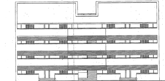
รูปด้าน ① SCALE 1 : 100
