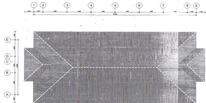
แปลนหลังคา 1:100
