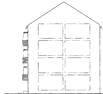
รูปด้าน 4 SCALE 1 : 100
