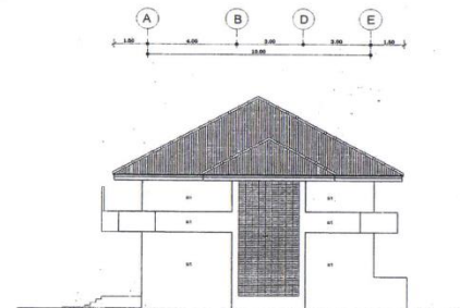
รูปด้าน ④ 1:100
