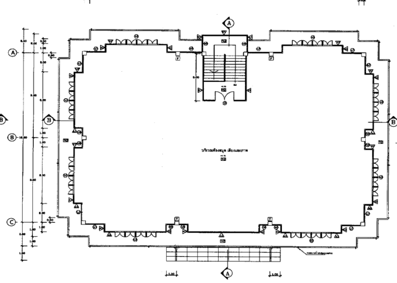
แปลนพื้นที่ชั้นบน 1:100
