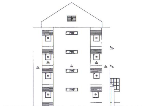
รูปด้าน ④ 1:100
