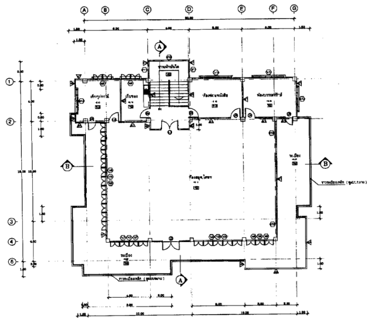
แปลนพื้นที่ 3 1:100
