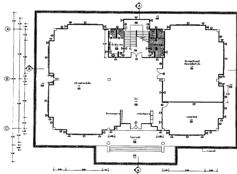
แปลนพื้นที่ชั้นล่าง 1:100
