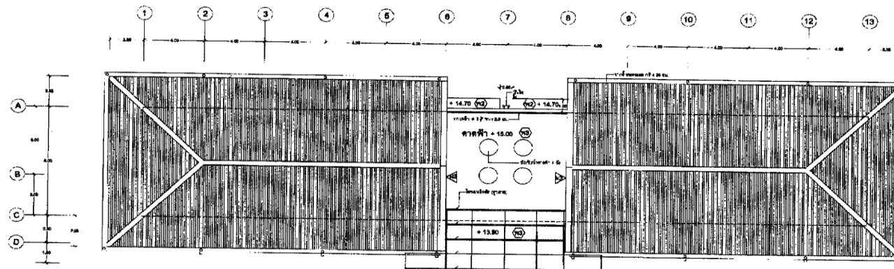
ผังชั้นหลังคา 1:100
