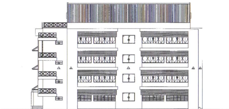
รูปด้าน ③ 1:100
