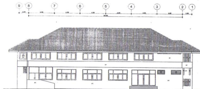
รูปด้าน ③ 1:100
