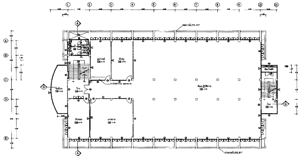
แปลนพื้นที่ 2 1:100
