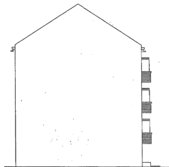
รูปด้าน ② SCALE 1 : 100
