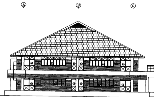
រូបគំនូរ (D) 1:100
