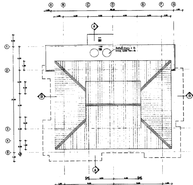
แปลนพื้นที่ 4 1:100
