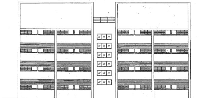
รูปด้าน ③ SCALE 1 : 100
