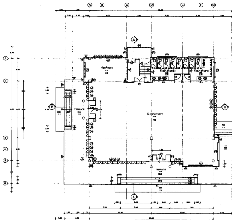
แปลนพื้นที่ล่าง 1:100
