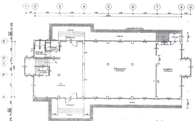
แปลนพื้นชั้นล่าง 1:100
