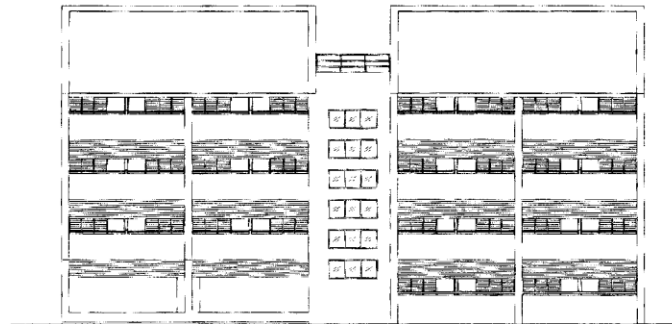
รูปด้าน 3 SCALE 1 : 100
