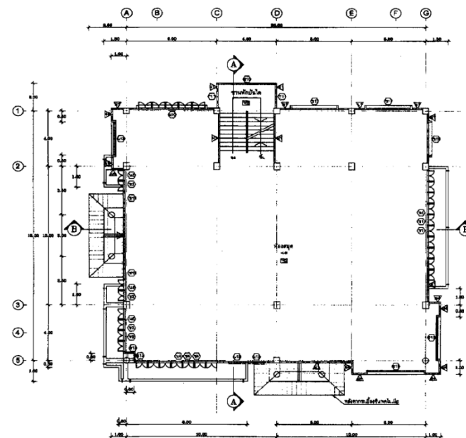
แปลนพื้นที่บน 1:100
