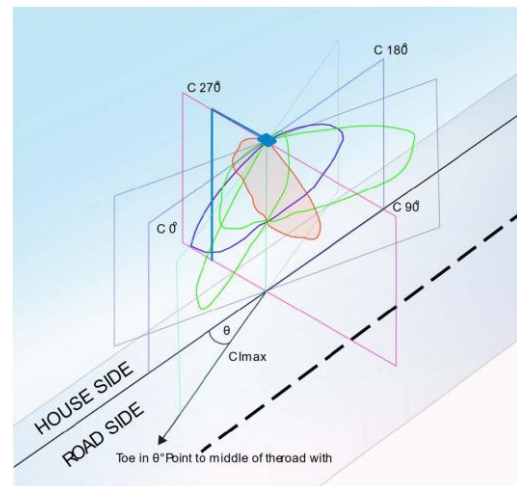
รูปที่ 16 การพิจารณาการกระจายความเข้มการส่องสว่างของโคมไฟในระบบพิกัด C- \gamma ตามมาตรฐาน CIE
