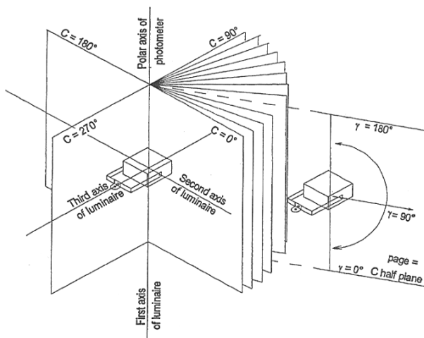
รูปที่ 16 การพิจารณาการกระจายความเข้มการส่องสว่างของโคมไฟในระบบพิกัด C- \gamma ตามมาตรฐาน CIE
