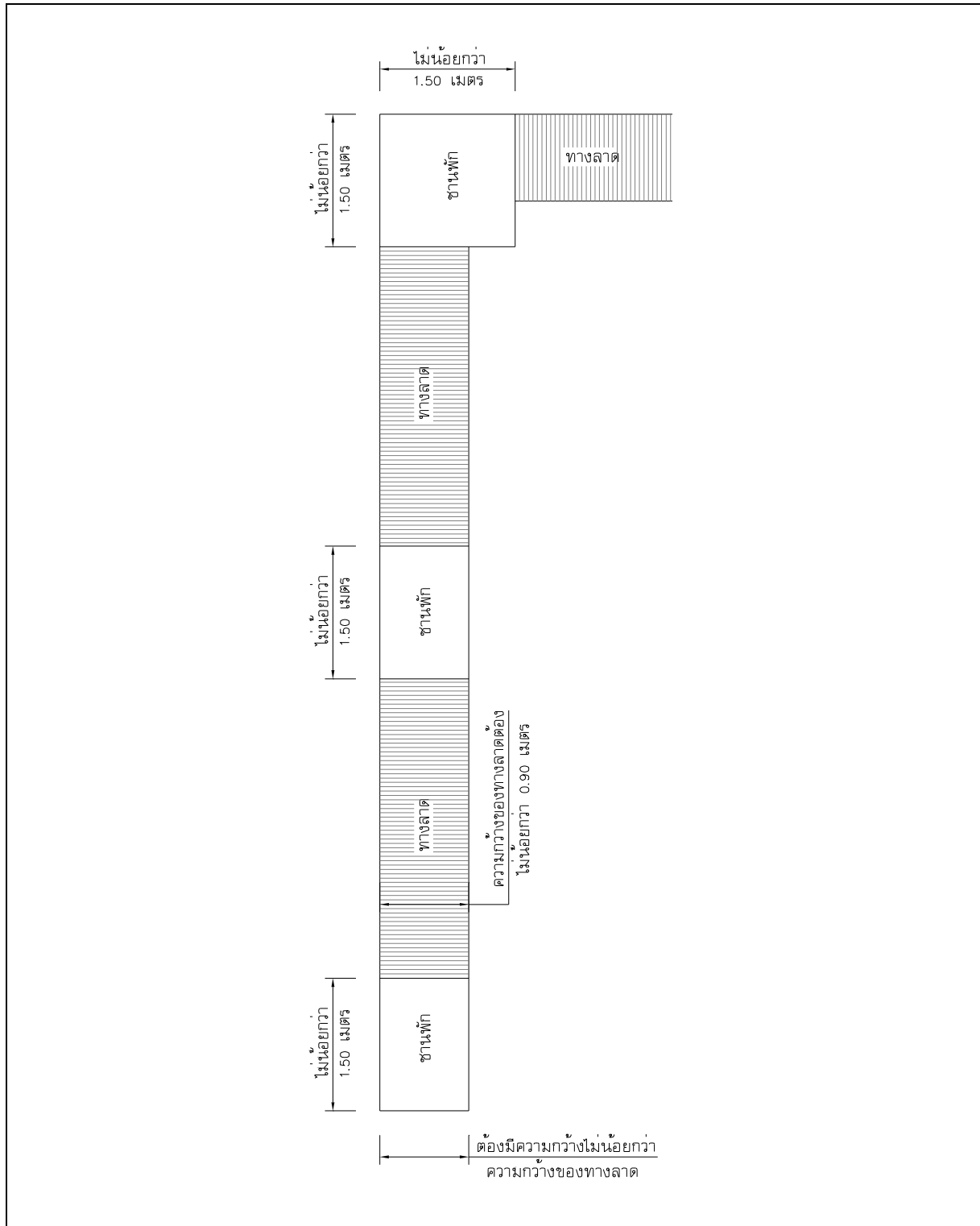
รูปที่ 10 ชานพักของทางลาด (ข้อ 3.1.7.3)
