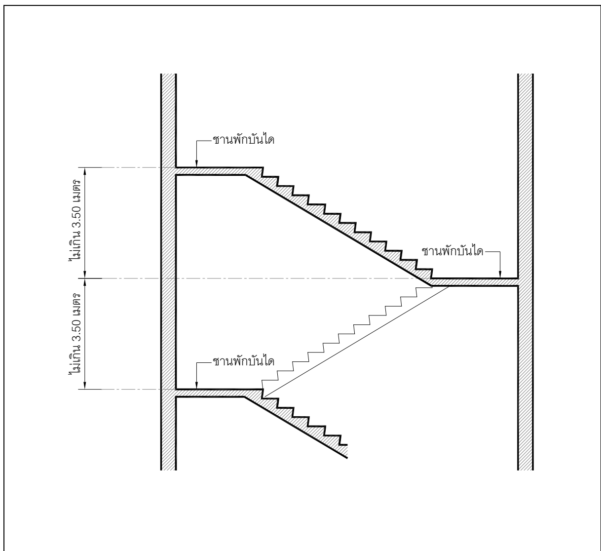
รูปที่ 9 ช่วงบันไดในแนวดิ่ง
