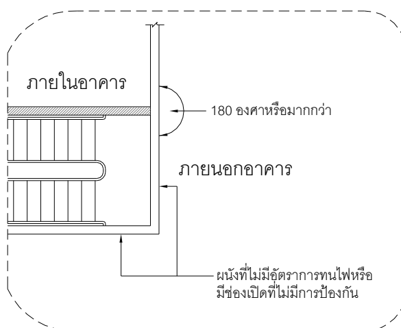
รูปที่ 17 ผนังปิดล้อมบันได (ข้อ 3.3.3.5)
