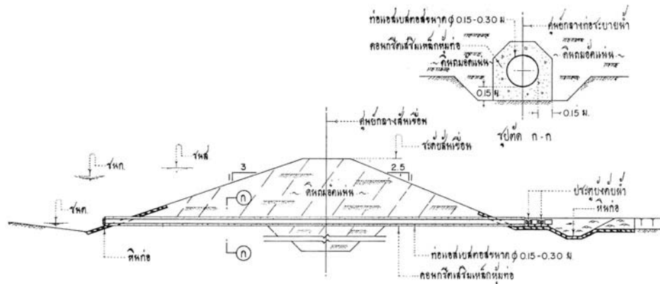
รูปที่ 8-8 รูปแบบทั่วไปของท่อบายน้ำขนาดเส้นผ่าศูนย์กลาง 15-30 เซนติเมตร
