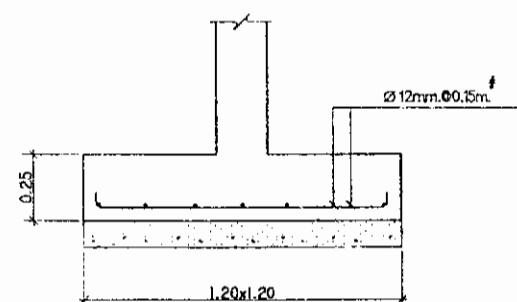
แบบขยายฐานราก F1
