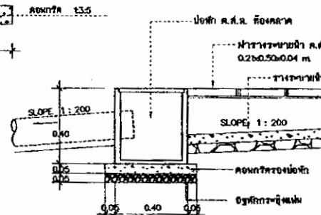
รูปตัดท่อระบายน้ำชนิดเปิดฟ้า
