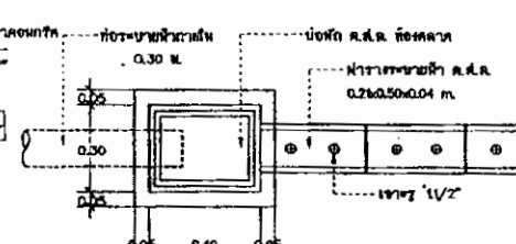
แปลนท่อระบายน้ำชนิดเปิดฟ้า
