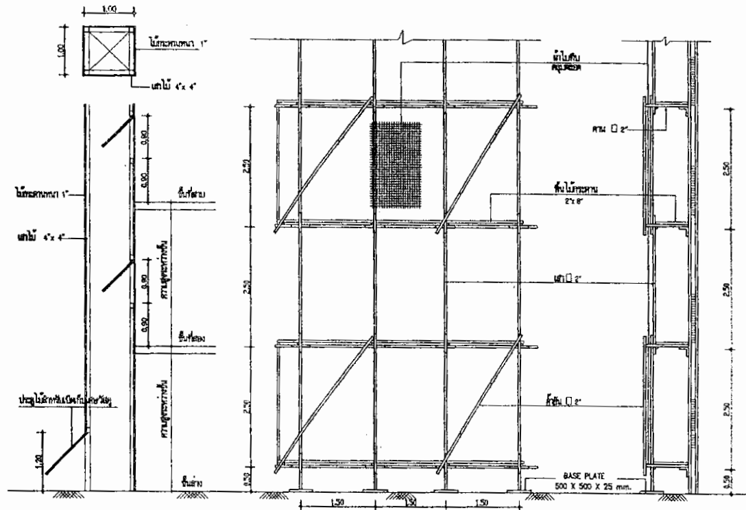
ปล่องรับเศษวัสดุ
