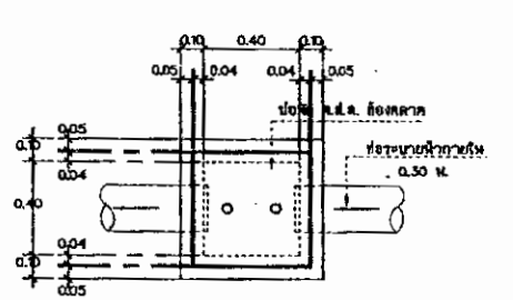
แปลนท่อระบายน้ำ, บ่อพักและวางระบายน้ำ
