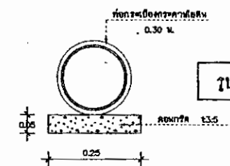
รูปตัดบ่อพัก, วางระบายน้ำ
