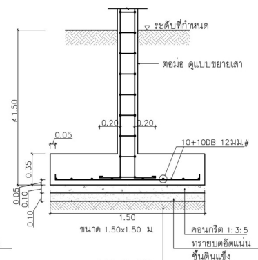
F3 1:25
