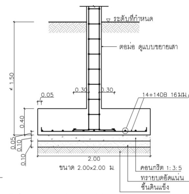
F5 1:25
