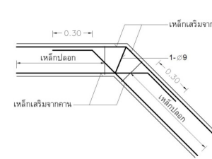
ผังขยายเหล็กในคานหักมุม
