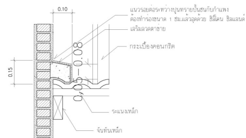
แบบขยายการทำบันลุมบนสันหลัง 1 : 10
