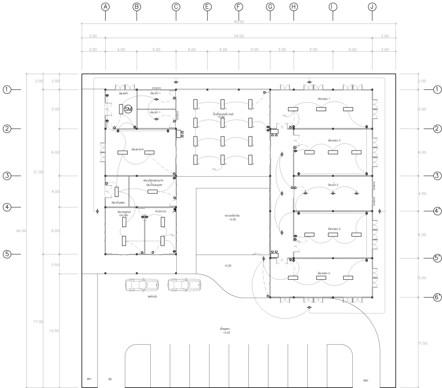
ผังไฟฟ้ากำลังและไฟฟ้าแสงสว่าง มาตราส่วน 1:150
