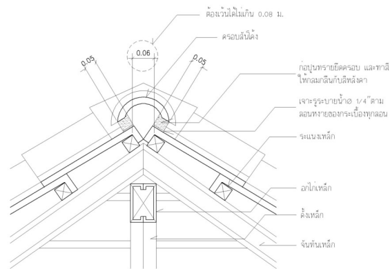
แบบขยายครอบด้าน 1 : 10
