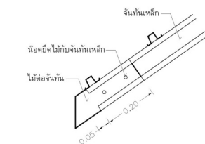
การต่อไม้รับแรงซาย
