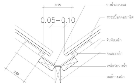
แบบขยายรางน้ำหลังคา 1 : 10
