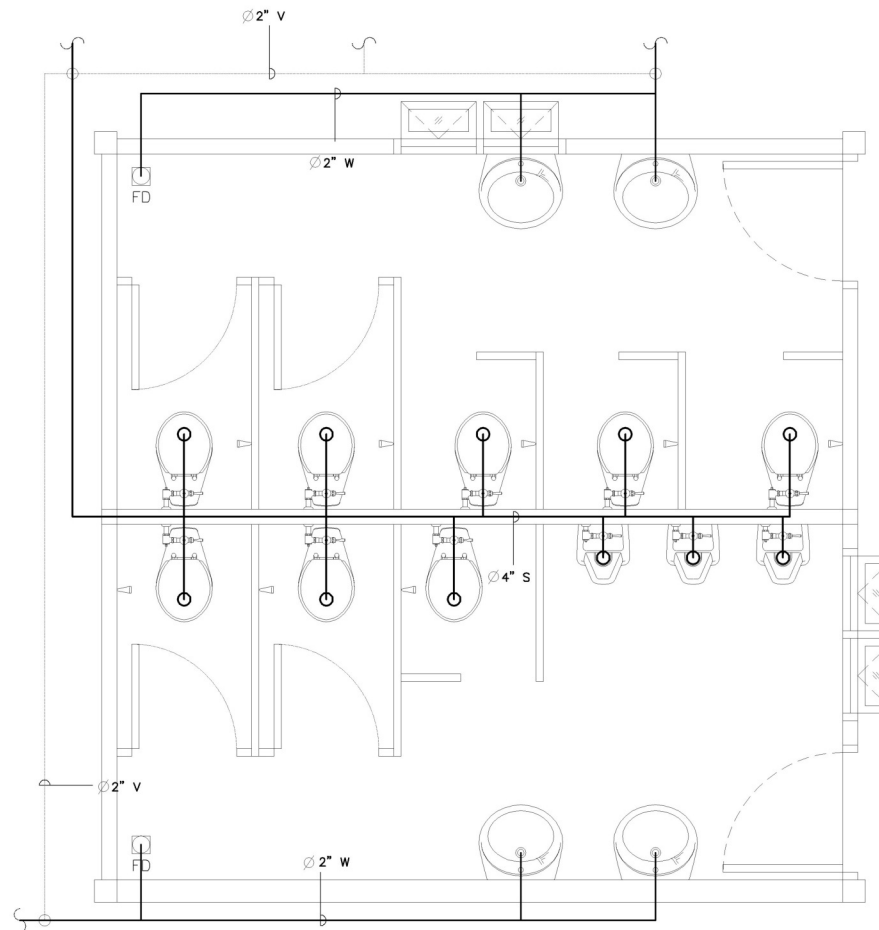
ห้องน้ำ 1 (น้ำเสีย)
