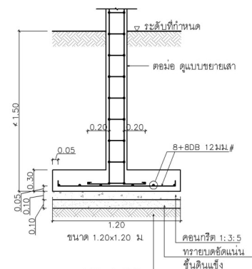
F2 1:25
