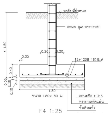
F4 1:25
