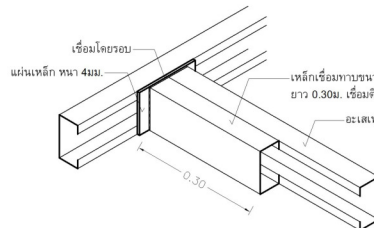
การเชื่อมชนอะเสเหล็ก
