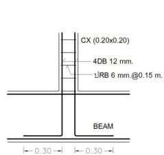
วางบนคาน
