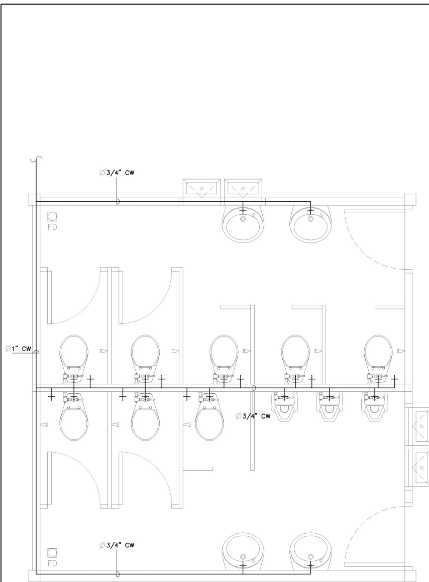
ห้องน้ำ 1 (ประปาเดินบน)
