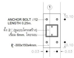
แปลน
