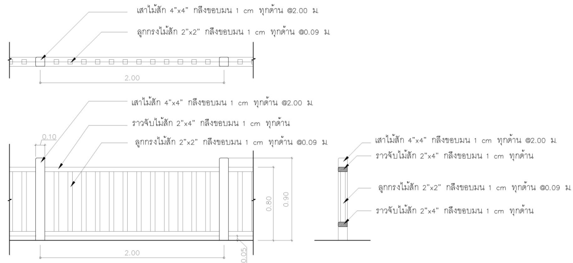
แบบขยายราวกันตก
