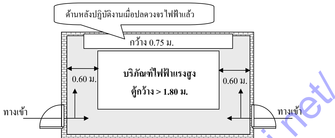
รูปที่ 5 ทางเข้าที่ว่างเพื่อปฏิบัติงาน
