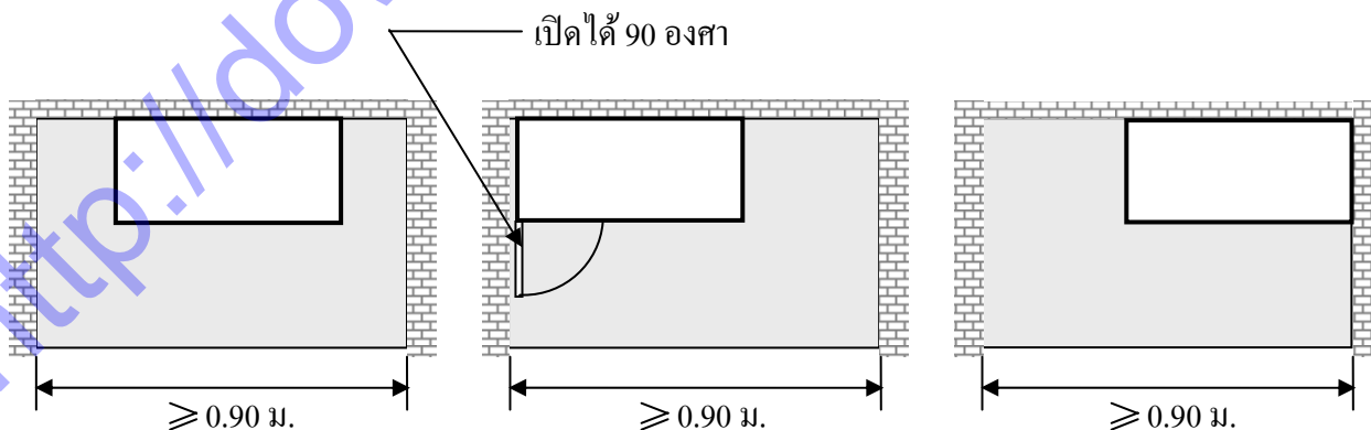
รูปที่ 1 ที่ว่างเพื่อการปฏิบัติงานของระบบแรงสูง
