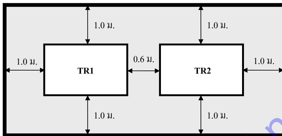
รูปที่ 8 ระยะห่างระหว่างหม้อแปลงกับผนังหรือประตูห้องหม้อแปลง (ข้อ 3.4.3.1.2)
