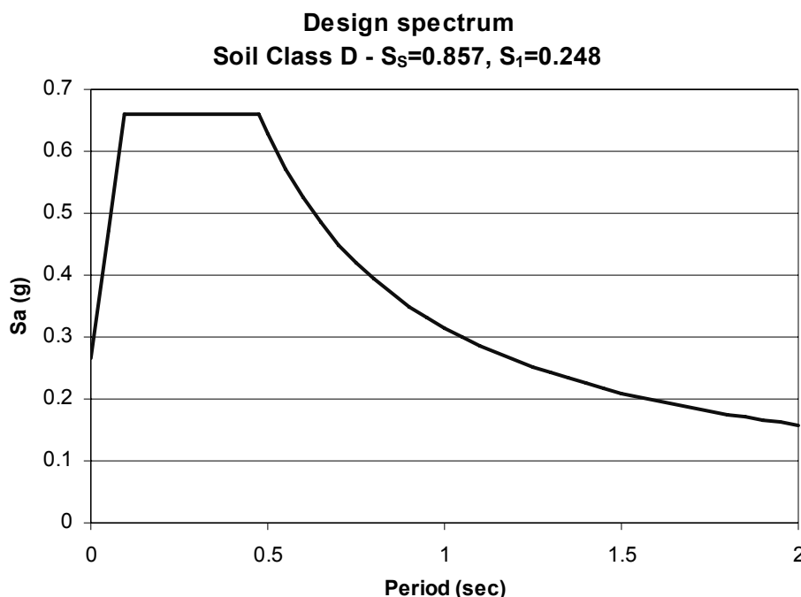
รูปที่ ข.2-1 ตัวอย่างความเร่งตอบสนองเชิงสเปกตรัมเพื่อการออกแบบ สำหรับที่ตั้งบนดินแน่น
