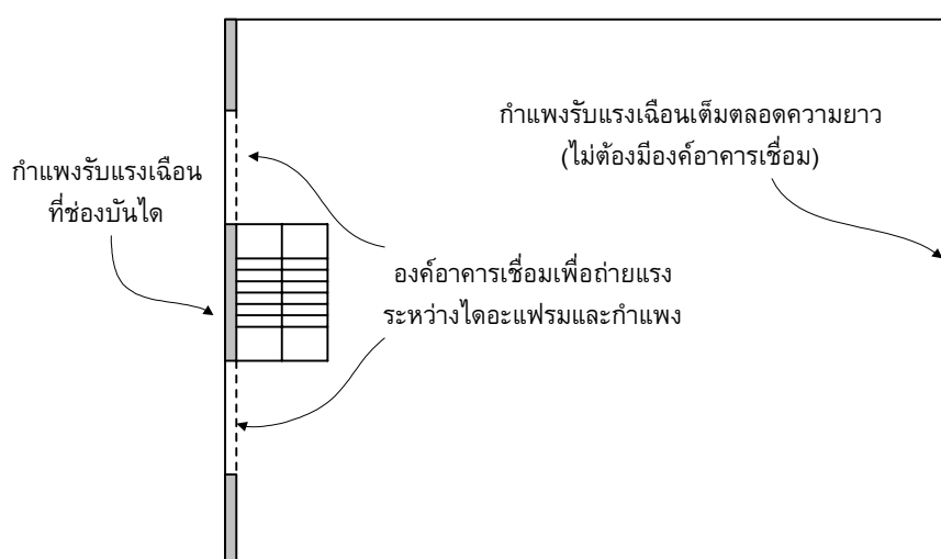
รูปที่ 2.9-1 องค์อาคารเชื่อมระหว่างไดอะแฟรมและกำแพง
