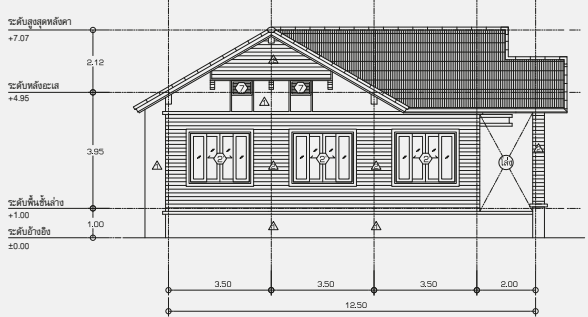
รูปด้าน 4
