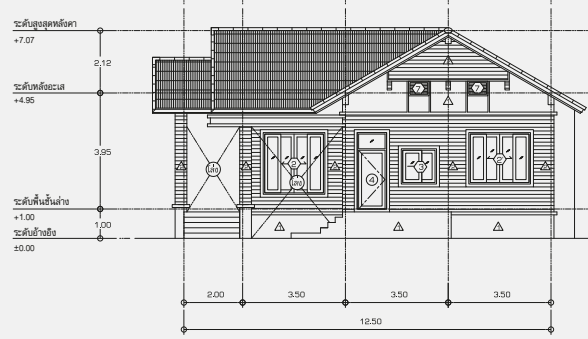
รูปด้าน 2
