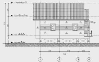
รูปด้าน 4
