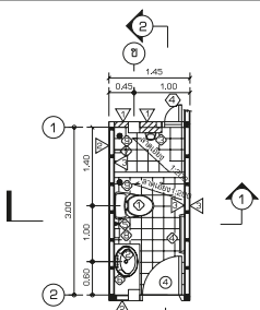
แบบขยายห้องน้ำ 1
