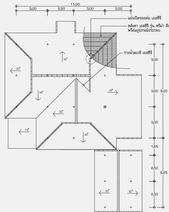
| แปลนหลังคา |
