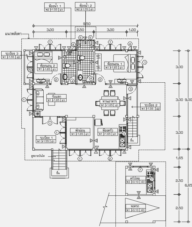
| แปลนพื้น |
