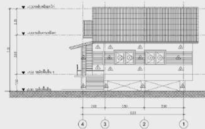
รูปด้าน 2
