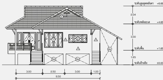
รูปด้าน 1
