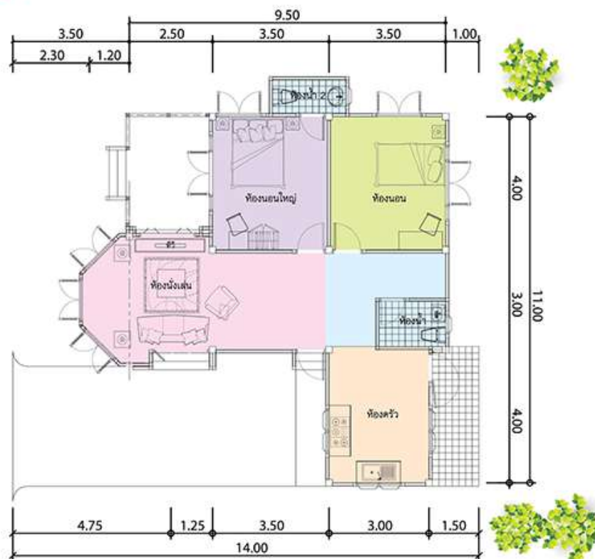
แปลนพื้นที่ส่วน
