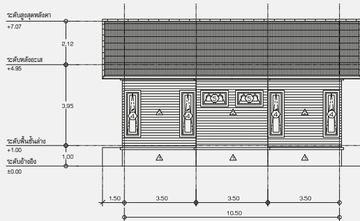
รูปด้าน 3
