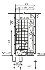
รูปตัด ①
