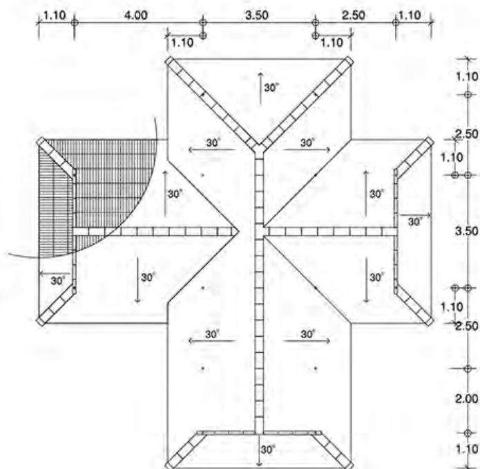
แปลนหลังคา
