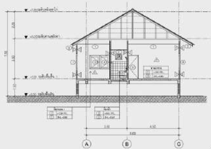
รูปตัด A-A
