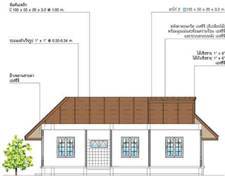
รูปตัด B
