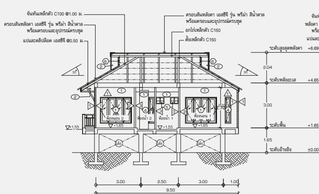
รูปตัด ก
