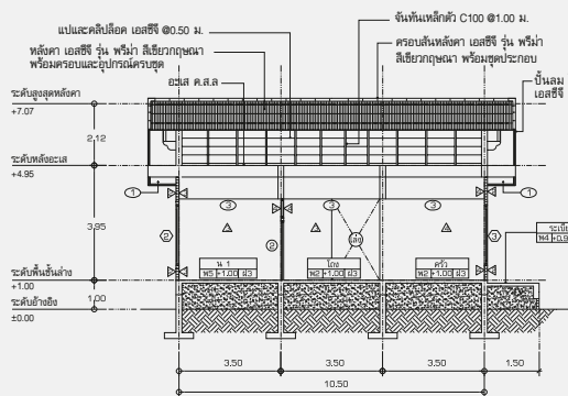
รูปตัด ๑
