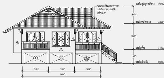
รูปด้าน 4
