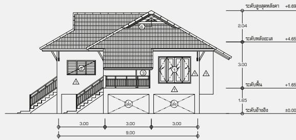
รูปด้าน 2
