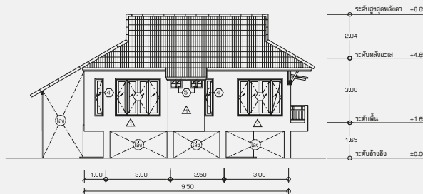
รูปด้าน 3
