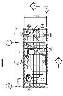
แบบขยายห้องน้ำ 2
