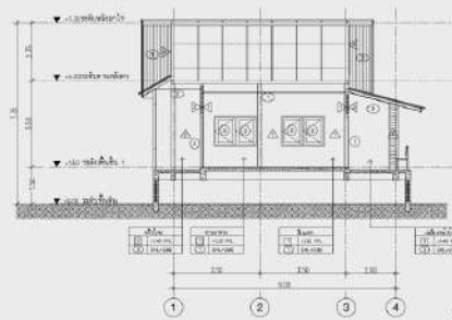
รูปตัด B-B
