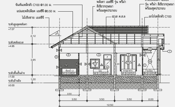
รูปตัด ๒
