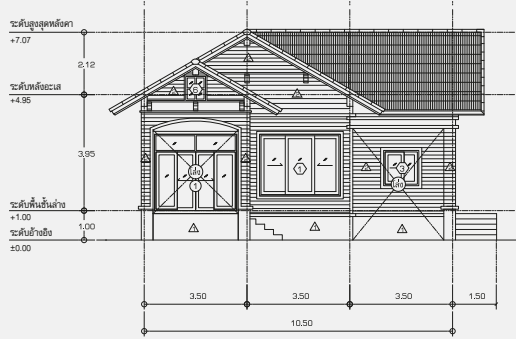
รูปด้าน 1
