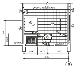
รูปตัด ②
