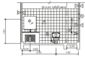
รูปตัด ②
