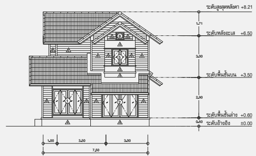
รูปด้าน 2
