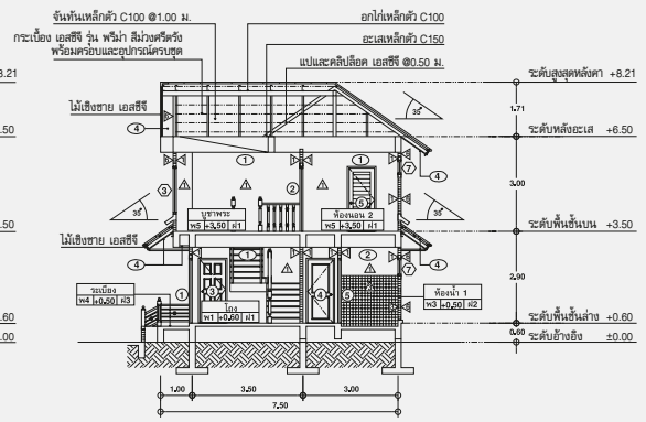
รูปตัด ข
