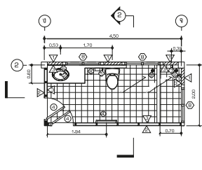
แบบขยายห้องน้ำ 1
