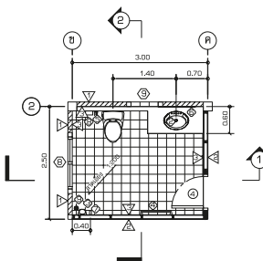
แบบขยายห้องน้ำ 2
