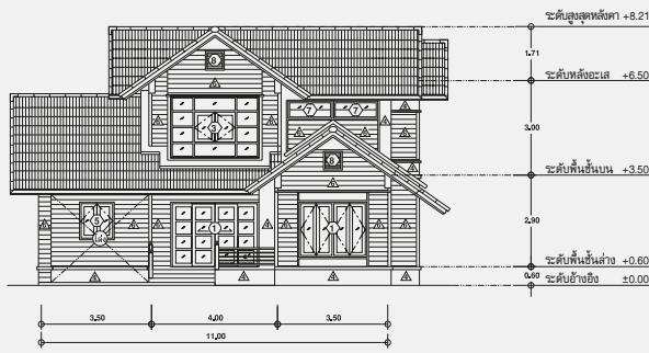
รูปด้าน 1
