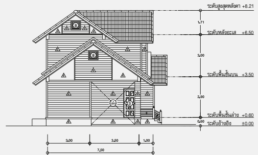
รูปด้าน 4
