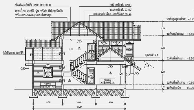
รูปตัด ก
