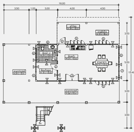
| แผนพื้นชั้นล่าง |
