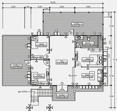
| แผนพื้นชั้นบน |
