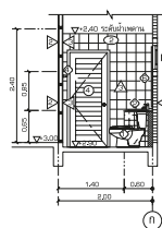
รูปตัด ②
