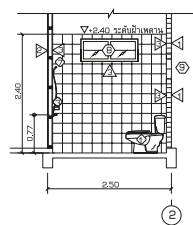
รูปตัด ②
