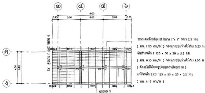
แปลนคานหลังคาและหลังคา 1:125
