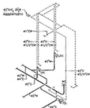
ไอโซเมตริกกระบบสุขาภิบาลห้องน้ำชาย
