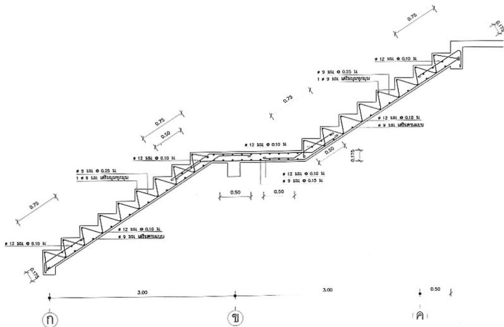
ST1 1:25
