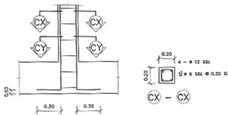
ขยาย ก การตั้งเสาคอนกรีตบนคานคอนกรีต
