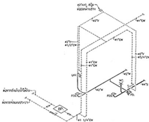
ไอโซเมตริกกระบบสุขาภิบาลห้องน้ำหญิง
