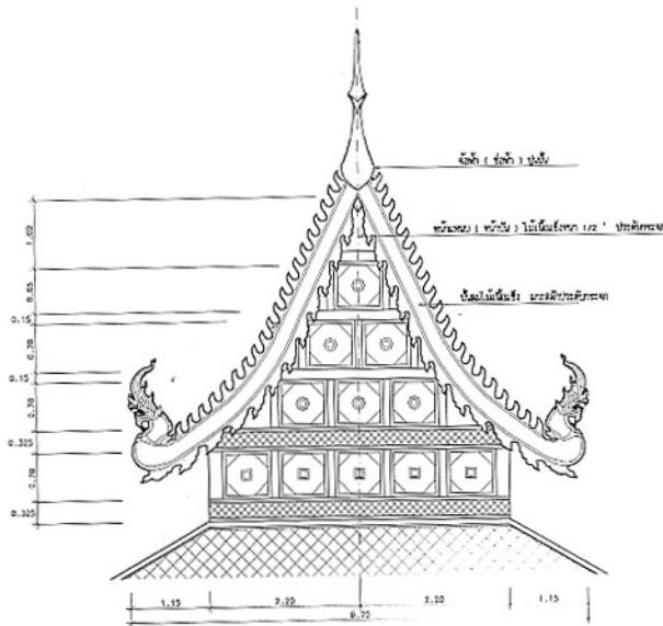
แบบขยายหน้าบัน
