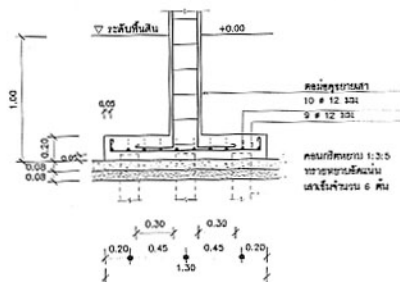
แบบขยายรูปตัด (F2) 1: 25
