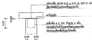
ขยาย ง การติดตั้งคอกไก่เหล็กบนเสาหรือคานคอนกรีต
