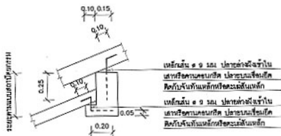
ขยาย ค การตั้งจันทันเหล็กและตะแคงเส้นเหล็กบนเสาหรือคานคอนกรีต RB2
