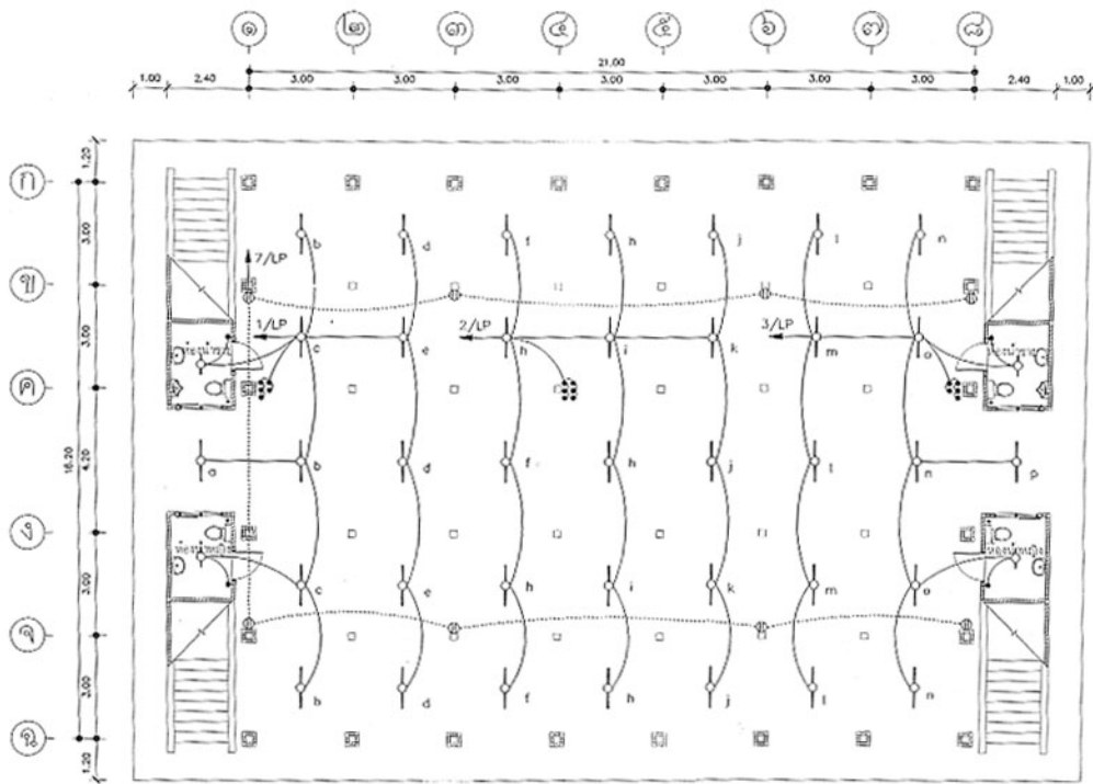
ผังไฟฟ้า ชั้นล่าง 1:100
