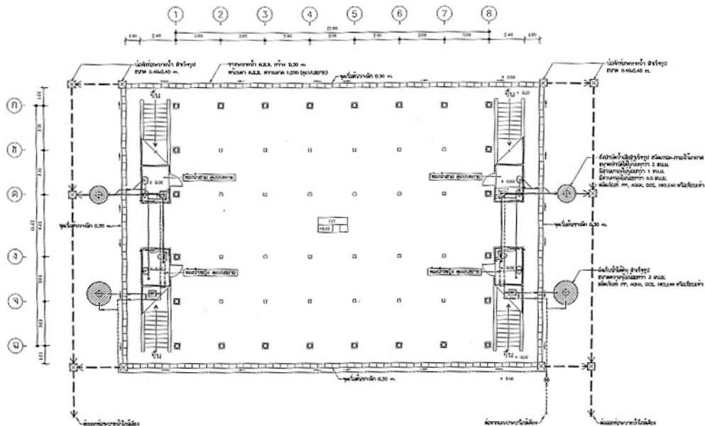
แปลนระบบฐานอาคาร 1 : 150
