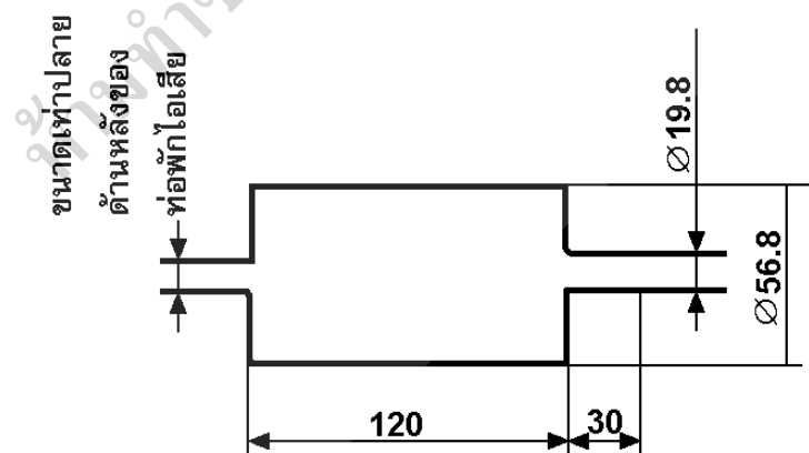
รูปที่ 6 ท่อพักไอเสียซีกบนที่ดึงโยกแล้ว (ข้อ 8.3.1.2(2.3))
