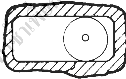
รูปที่ 9 แสดงการหุ้มท่อพักไอเสียด้วยฉนวนความร้อน (ข้อ 8.3.1.2(3))
