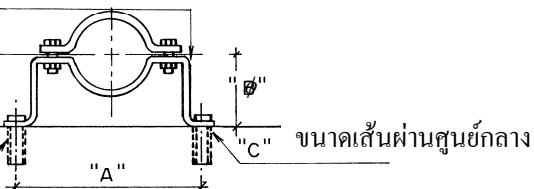
ตาราง ค2 ขนาดแคลมป์สำหรับท่อเดี่ยว
