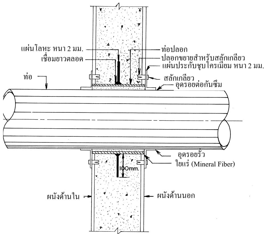
ท่อปลอกผ่านผนังภายนอก
