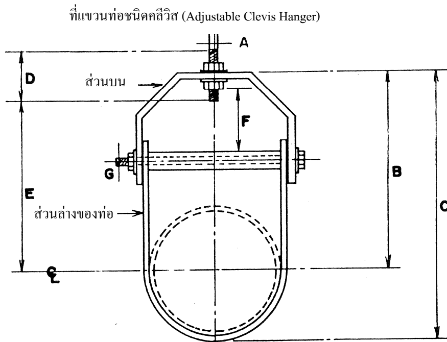
ตาราง ค11 ขนาดของที่แขวนท่อแบบคลีวิส
