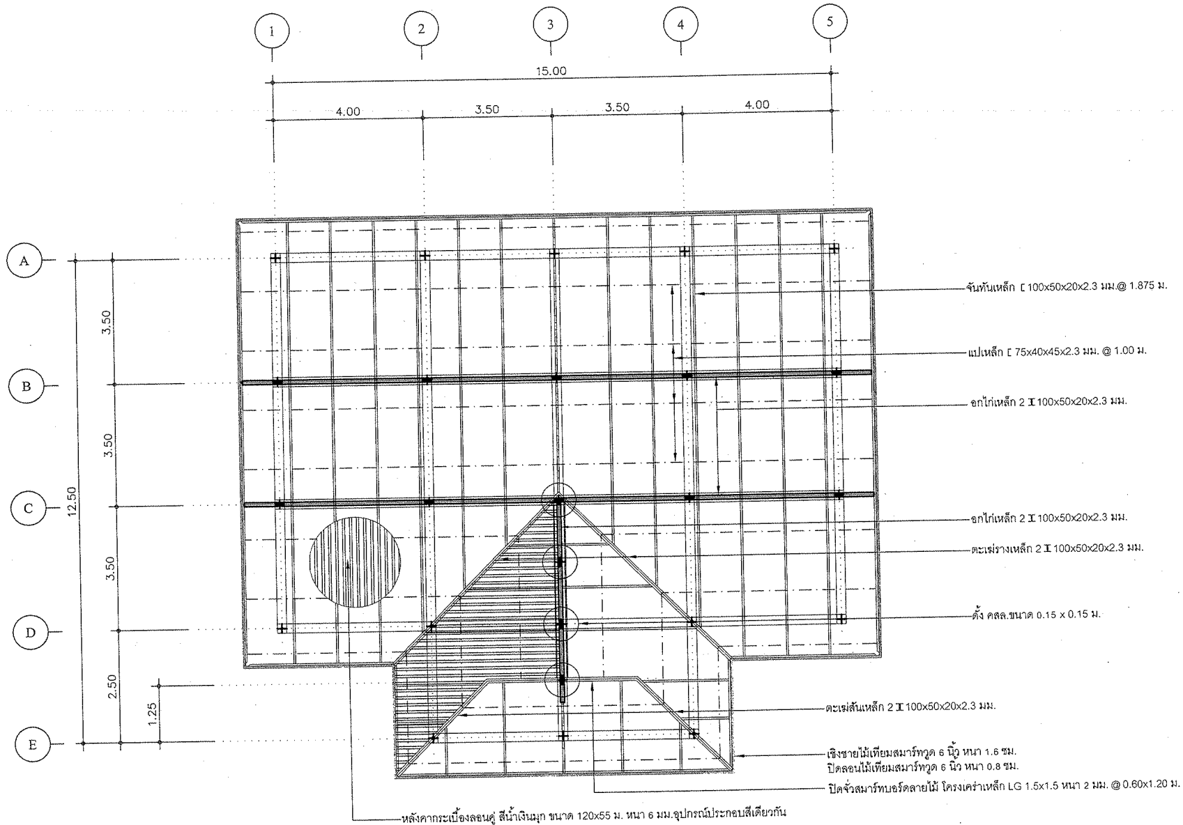
แปลนโครงหลังคา
