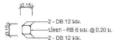
เสาคอนกรีต
