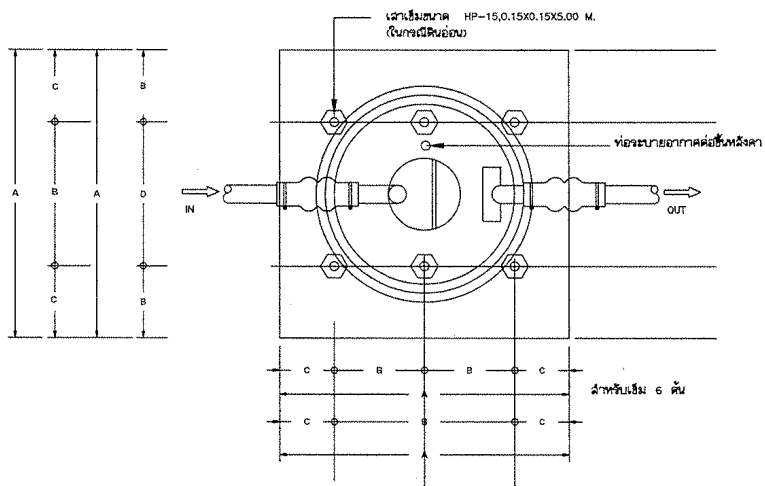
แบบแปลนถังสำเร็จรูปขนาด 3 - 5 คน
