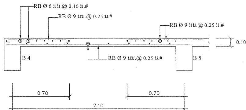
ขยายพื้น S1 ( รูปตัดด้านยาว )
