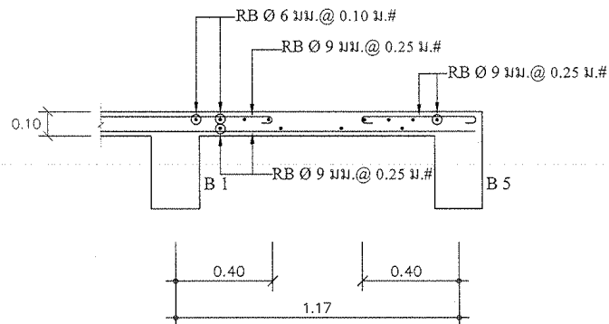
ขยายพื้น S1 ( รูปตัดด้านสั้น )
