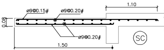
รายละเอียดการเสริมเหล็กพื้น คสล. (รูปตัดทางสั้น)
