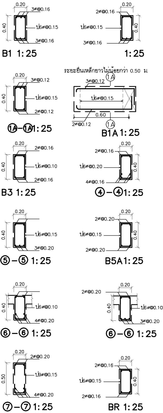
แบบขยายคาน
