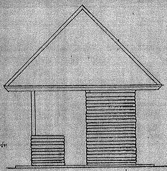
รูปด้านข้าง 1:50
