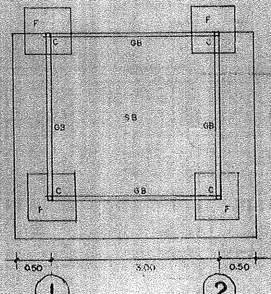
แปลนพื้น 1:50
