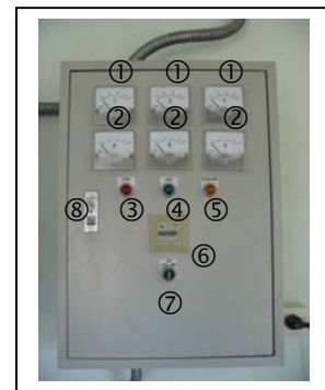
ลักษณะภายนอกตู้ควบคุม เครื่องสูบน้ำดิบ (แบบจมน้ำ)
