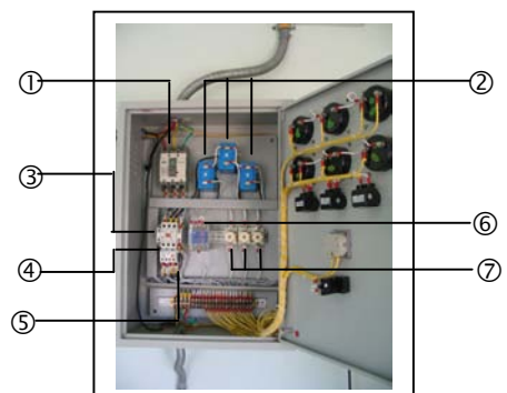
ลักษณะภายในตู้ควบคุม เครื่องสูบน้ำดิบ (แบบจมน้ำ)
