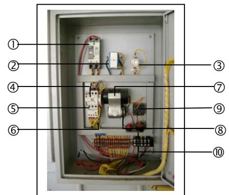
ลักษณะภายในตู้ควบคุม เครื่องสูบน้ำดิบ (แบบจมน้ำ)
