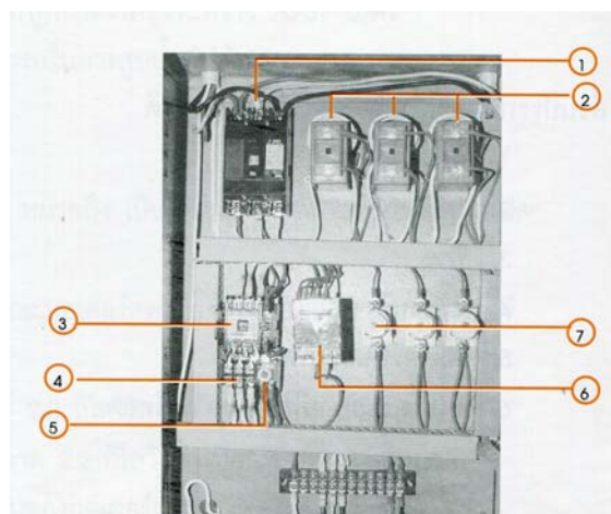
ลักษณะภายในตู้ควบคุมเครื่องสูบน้ำดี
