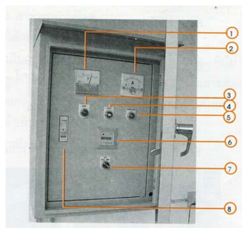
ลักษณะภายนอกตู้ควบคุมเครื่องสูบน้ำดี
