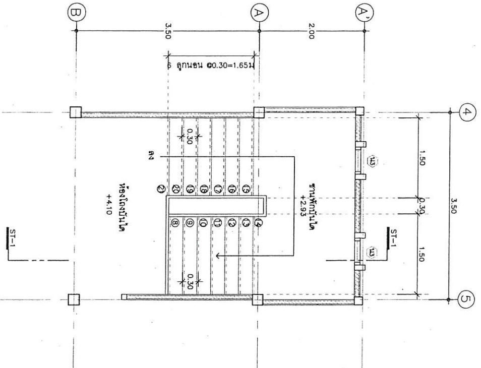
แบบขยายแปลนบันไดขึ้นบน SCALE 1 : 50
