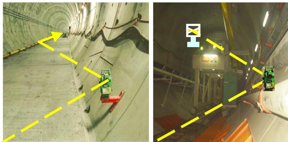
ภาพที่ ๗ วงรอบภายในอุโมงค์โดยเทคนิค Double Zigzag Traverse
