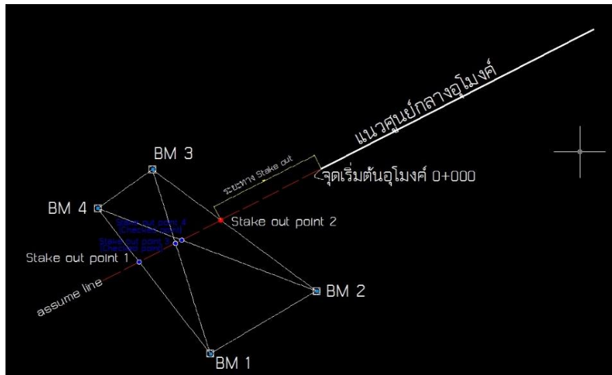
ภาพที่ ๓ การกำหนดตำแหน่ง (Stake Out) จุดในแนวอิมงค์จากหมุดหลักฐานถาวร
