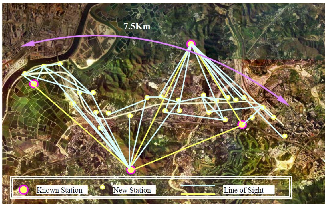
ภาพที่ ๒ ตัวอย่างเส้นวงรอบ เพื่อสร้างหมุดควบคุมทางราบตามแนวอุโมงค์
