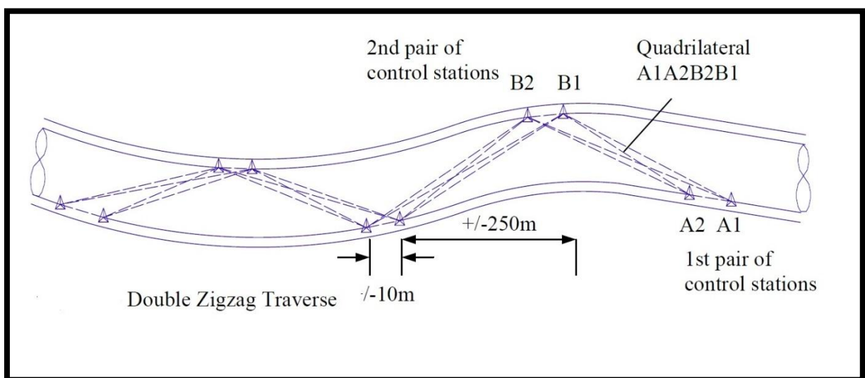
ภาพที่ ๖ ตัวอย่างการกำหนดวงรอบภายในอุโมงค์โดยเทคนิค Double Zigzag Traverse
