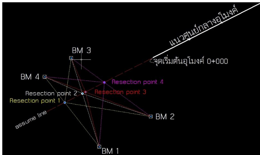
ภาพที่ ๔ การคำนวณค่าพิกัดย้อนกลับ (Resection Computation) ของจุดในแนวอิมงค์จากหมุดหลักฐาน
