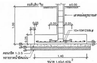
ฐานรากแผ่ F2 1:25
