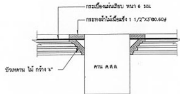
รูปตัด (A) ขยายผ้าเพดาน มาตราส่วน 1:10
