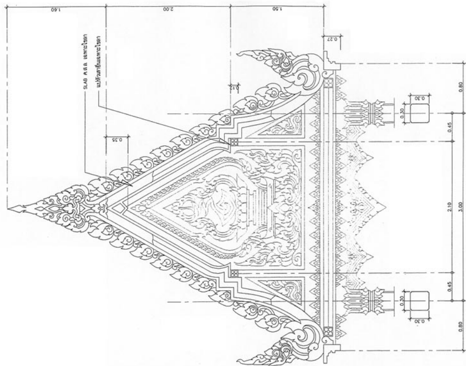
ขยายหน้าบัน ส่วนมุขยื่น 1:25
