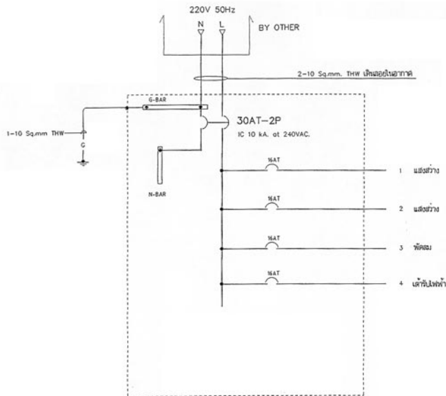
แผงสวิตช์อัตโนมัติ "LP"
