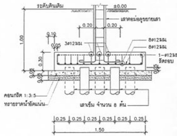
ฐานราก คสล F3 1:25
