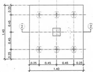
แผนฐานราก F2 1:25
