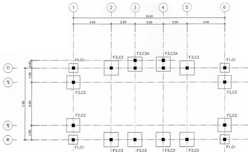
แปลนฐานรากและเสาตอม่อ มาตราส่วน 1:100
