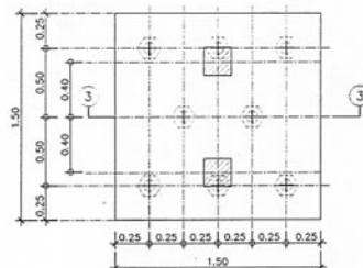
แผนฐานราก F3 1:25
