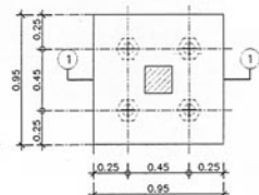
แผนฐานราก F1 1:25
