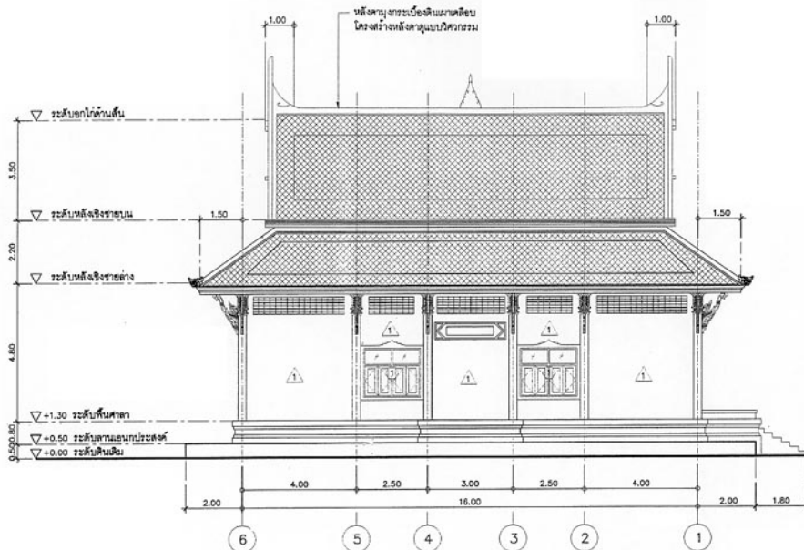
รูปด้าน 3 A-09 1:100
