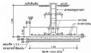
ฐานรากแผ่ F3 1:25
