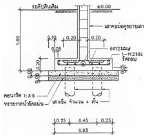
ฐานราก คสล F1 1:25
