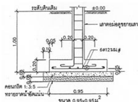
ฐานรากแผ่ F1 1:25
