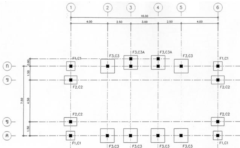
แปลนฐานรากเสาเข็มและเสาตอม่อ มาตราส่วน 1:100
