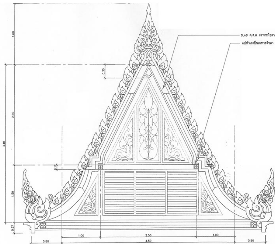
ขยายหน้าบรรณ 1:25
