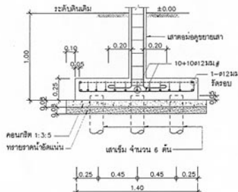
ฐานราก คสล F2 1:25
