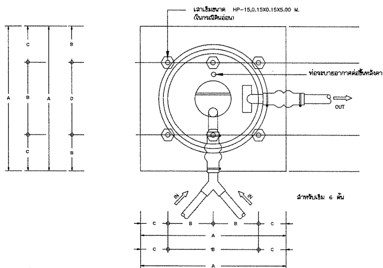
แบบแปลนถึงสำเร็จรูป
