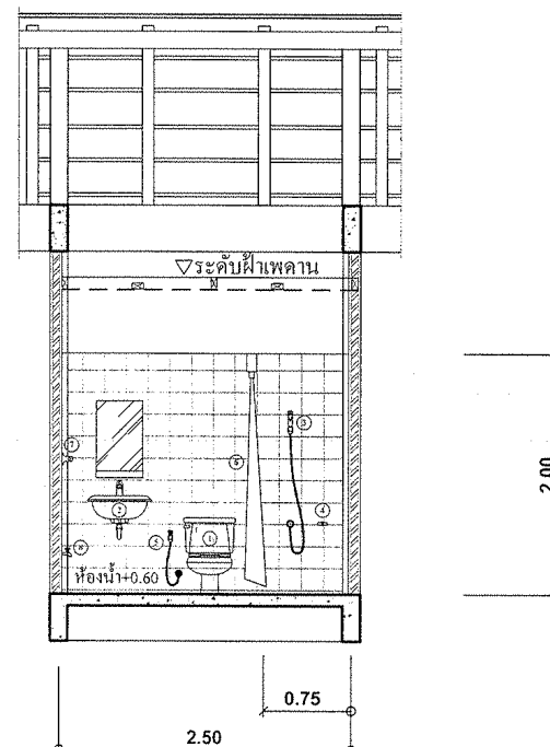
รูปตัดห้องน้ำ (B)
