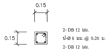
เสาดิ่ง
