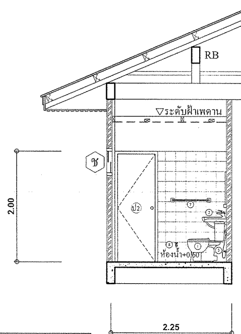
รูปตัดห้องน้ำ (A) มาตราส่วน 1 : 50
