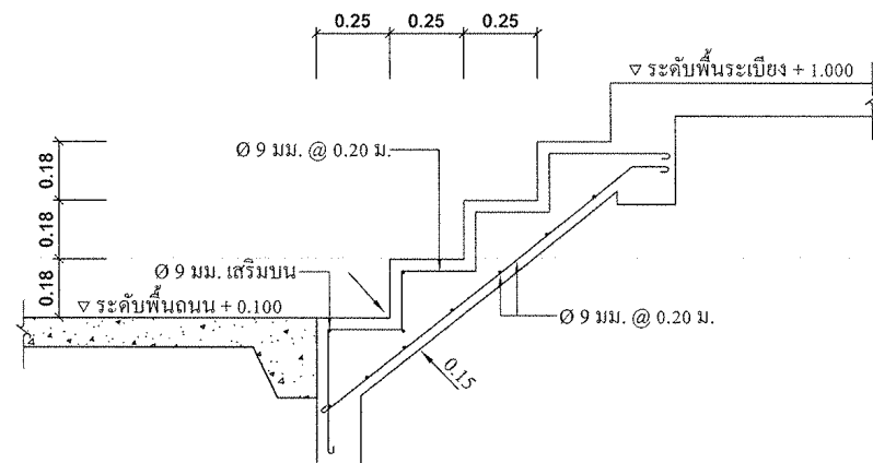
ขยายบันได ST1 มาตราส่วน 1 : 20
