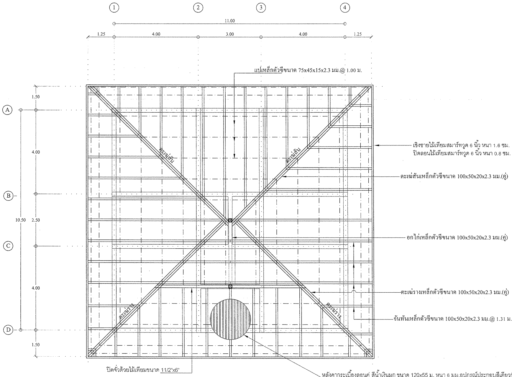
แปลนโครงสร้างหลังคา มาตราส่วน 1 : 75
