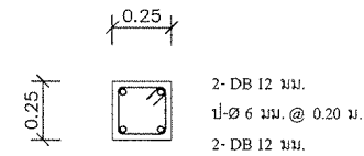
C1 (ต่อม่อ)
