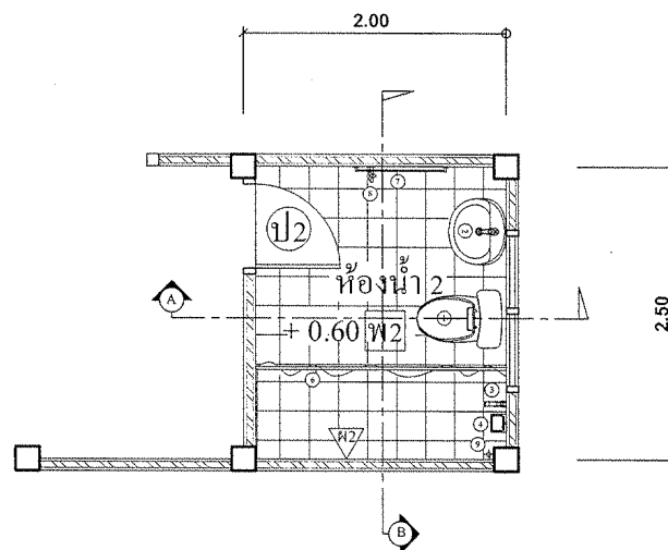
แปลนห้องน้ำ 2
