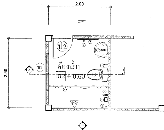
แปลนห้องน้ำ 1 มาตราส่วน 1 : 50
