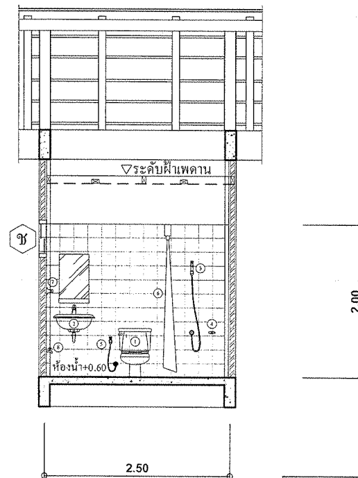
รูปตัดห้องน้ำ (B) มาตราส่วน 1 : 50
