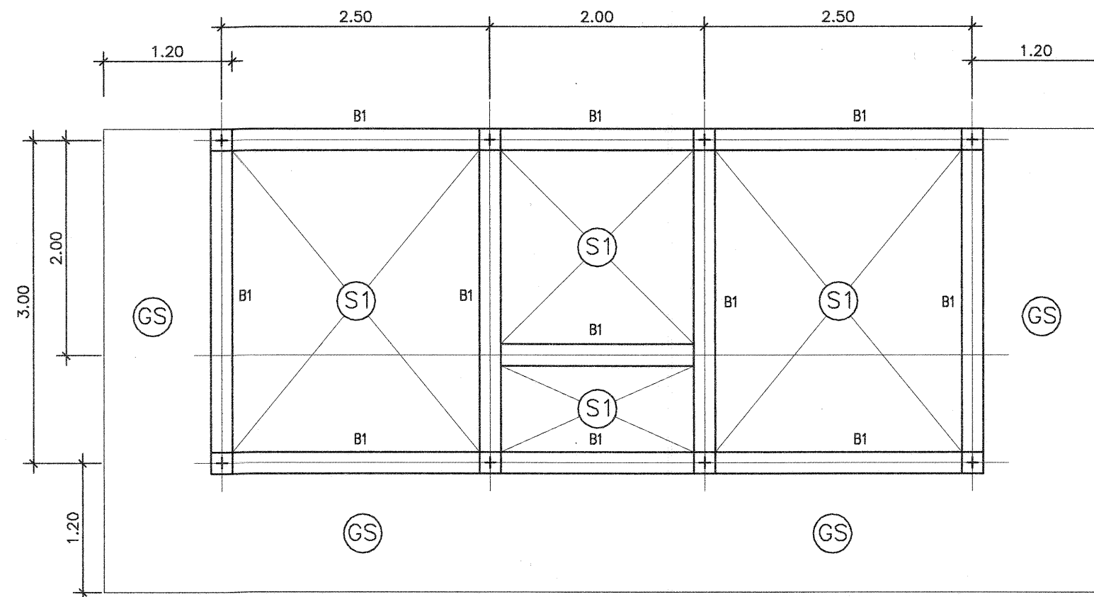
แปลน เสา คาน พื้น มาตราส่วน 1:50
