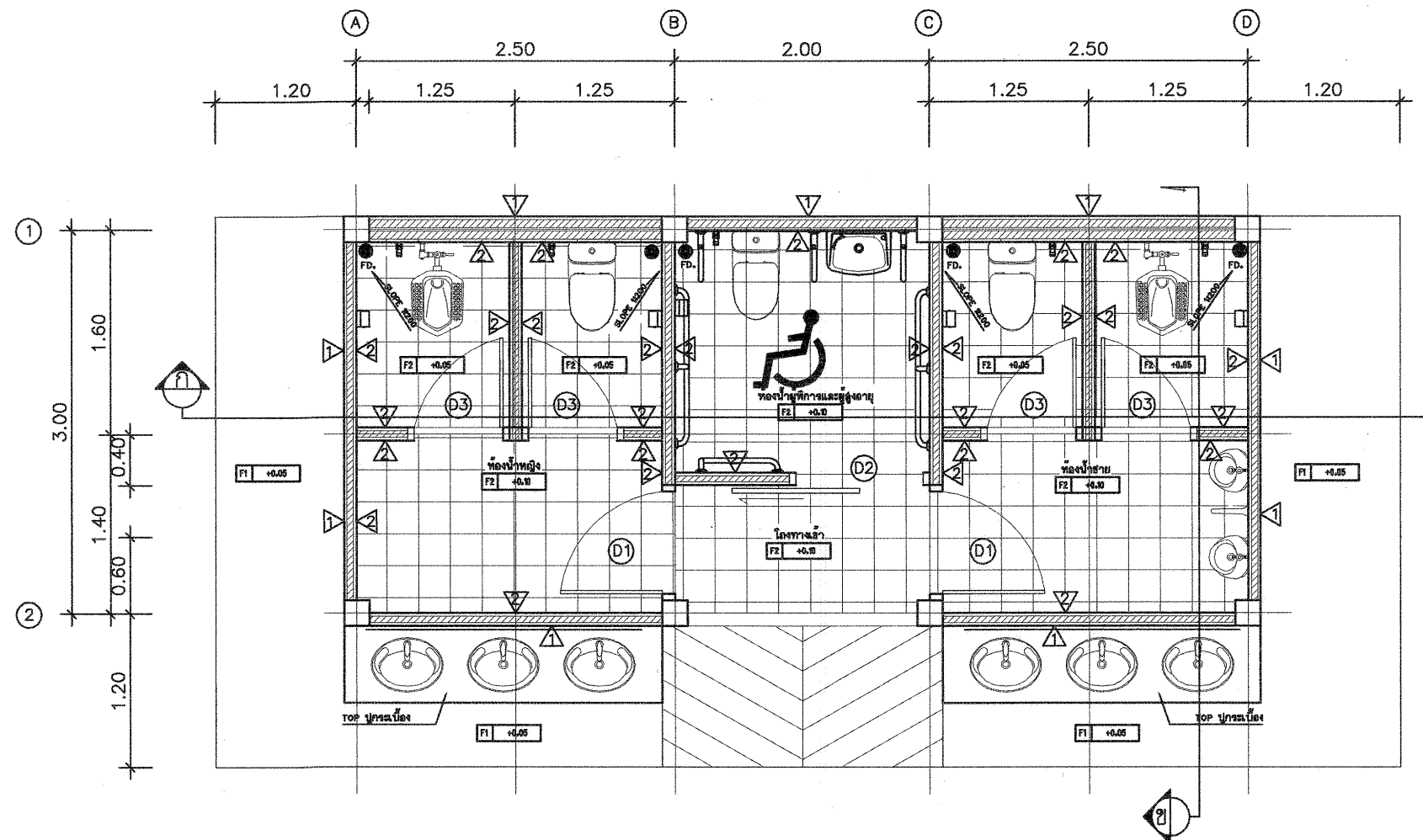
แปลนพื้น มาตราส่วน 1:50
