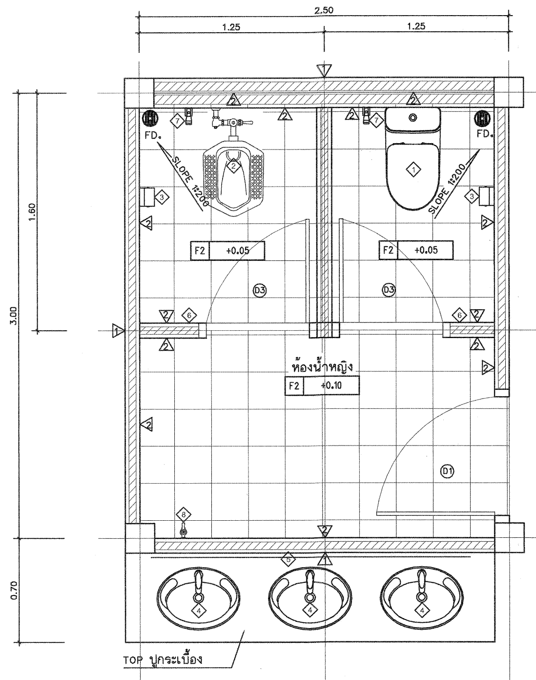
แบบขยายห้องน้ำหญิง มาตราส่วน 1:25
