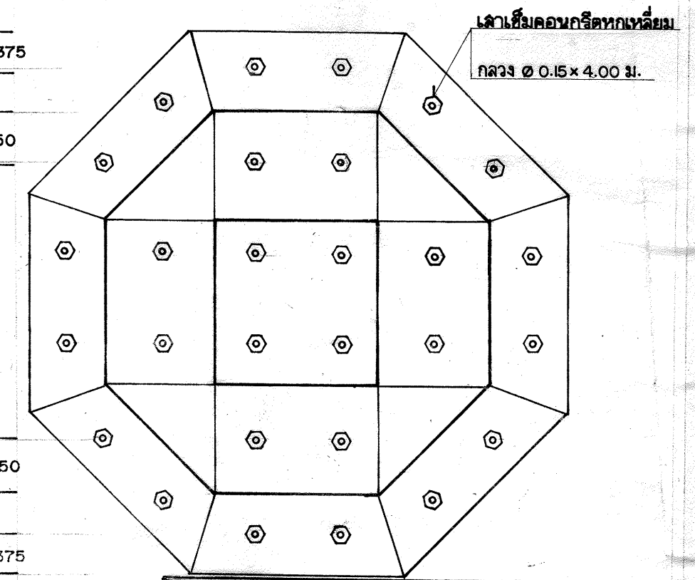
แปลนแสดงตำแหน่งเสาเข็ม มาตราส่วน 1:50
