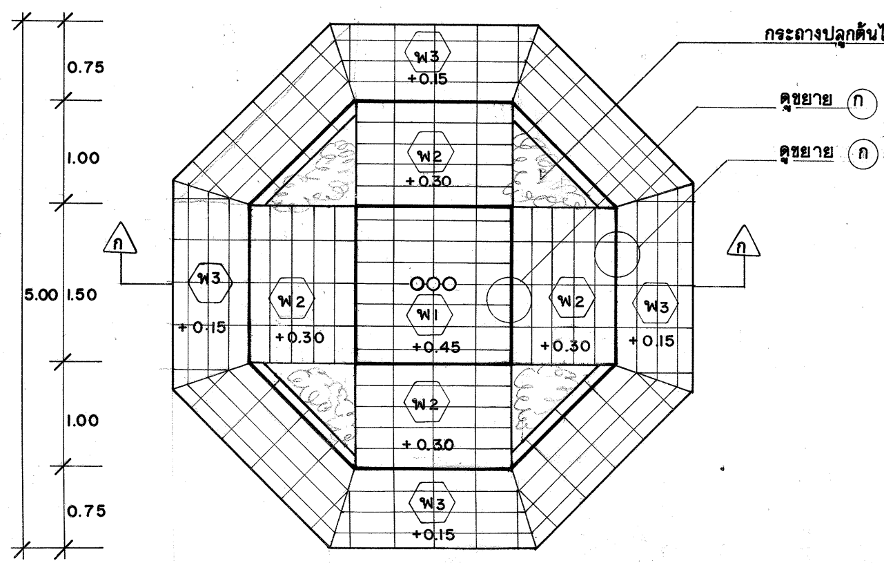
แปลนเสาเข็ม มาตราส่วน 1:50
