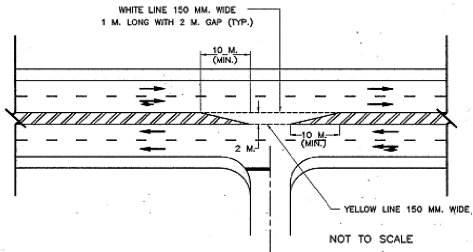
รูปที่ 8(d) การเปิดเกาะกลางของเกาะสี่บริเวณทางเชื่อมตามมาตรฐานของกรมทางหลวง
