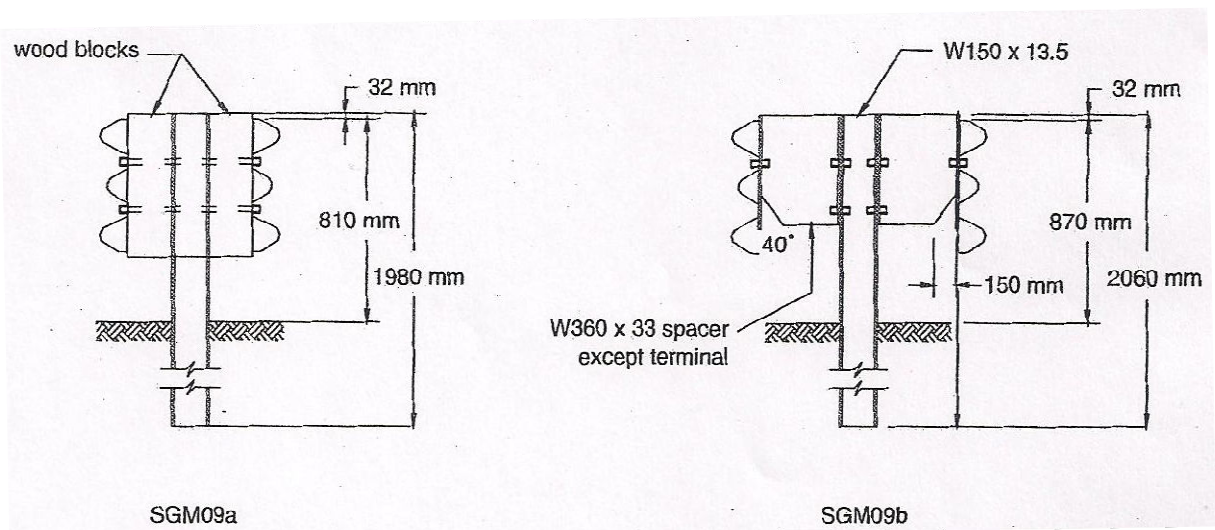
รูปที่ 25(a) Strong-post three-beam median barrier (Semi-Flexible Type)
