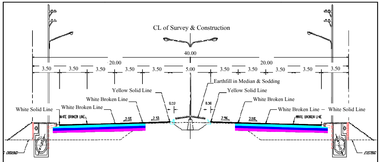
รูปที่ 37 รูปตัดที่ 2.4 ขยายคันทางเดิมแบบ Raised Median เต็มเขตทาง 40 ม.และ Overlay คันทางเดิม
