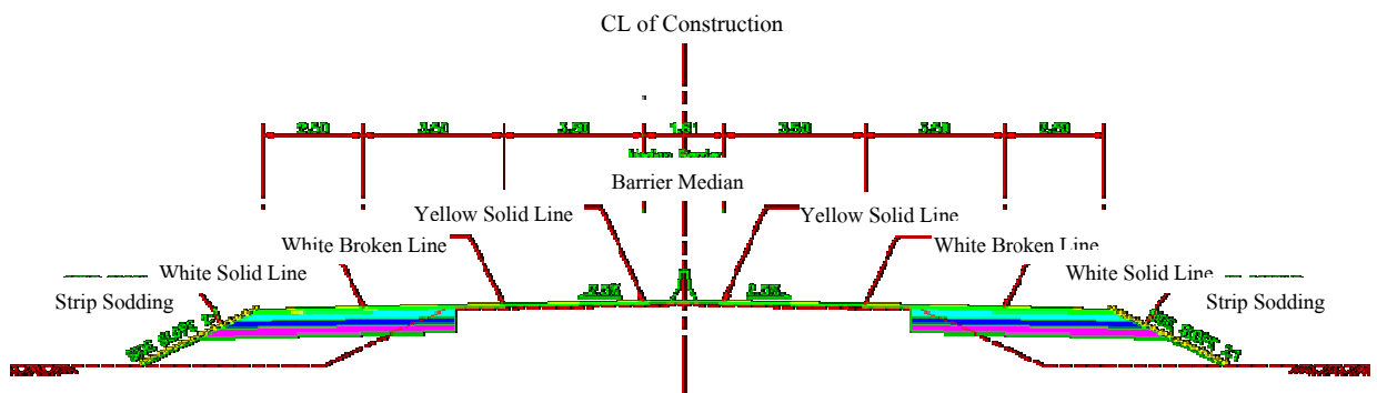
รูปที่ 42 รูปตัดที่ 4.1 ขยายคันทางเดิมแบบ Barrier Median (ขึ้นกลางคันทางเดิม)
