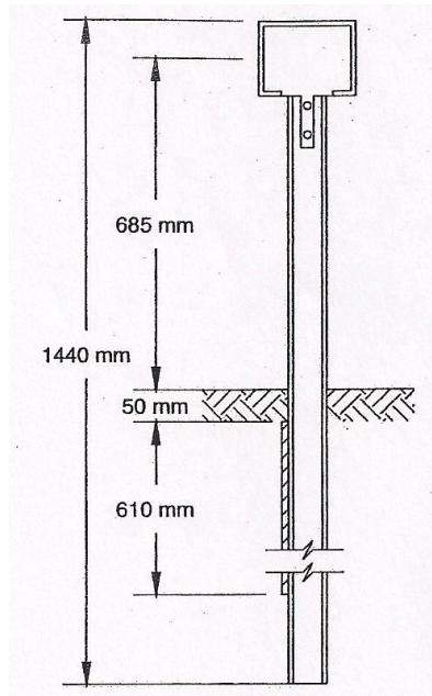
รูปที่ 23(a) Weak-post W-beam median barrier (Semi-Flexible Type)
