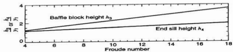
(ค) กราฟสำหรับหาความสูงของ baffle blocks และ end sill
