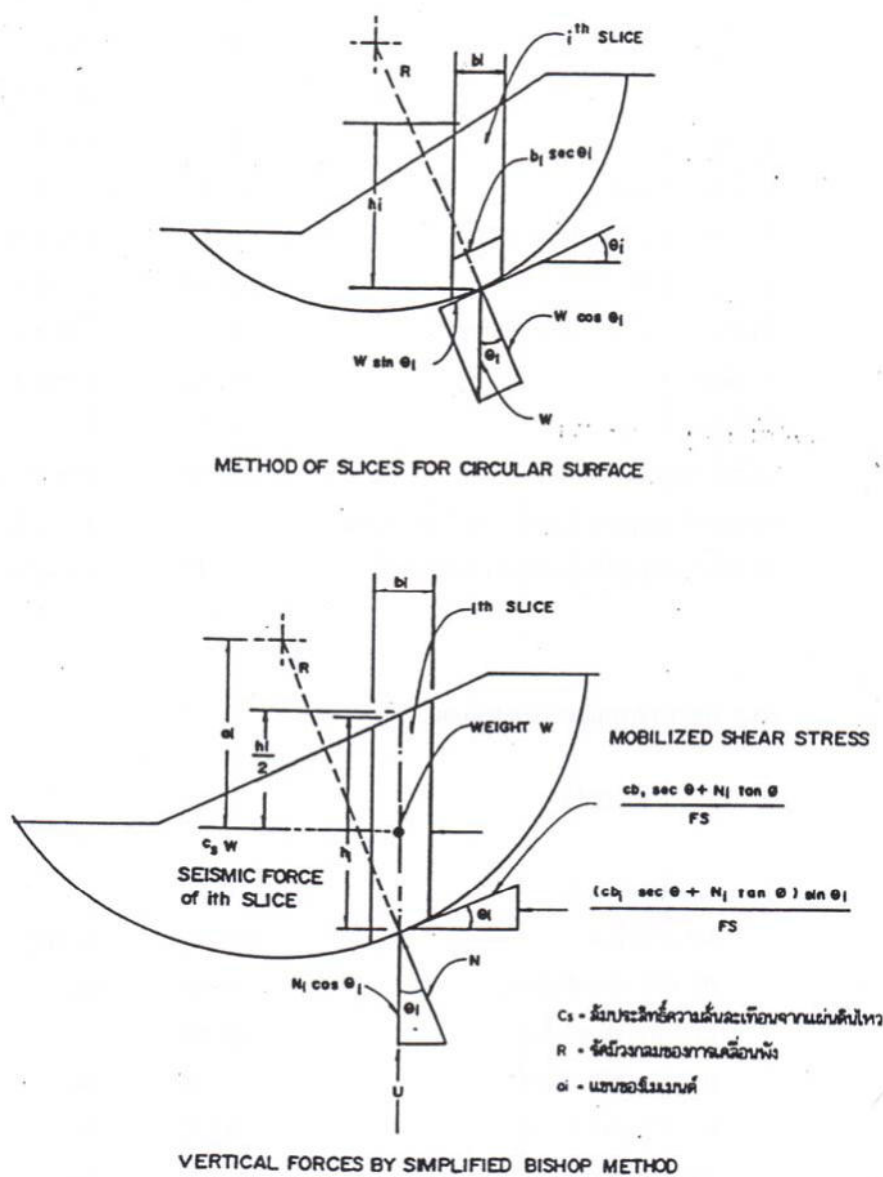
รูปที่ 3-3 แสดงการวิเคราะห์ความมั่นคงของลาดเขื่อนโดยวิธี Simplified Bishop Method ที่มา : เอกสารประกอบการบรรยาย เรื่อง “เกณฑ์กำหนดค่าในการออกแบบเขื่อน” gtz, 2544
