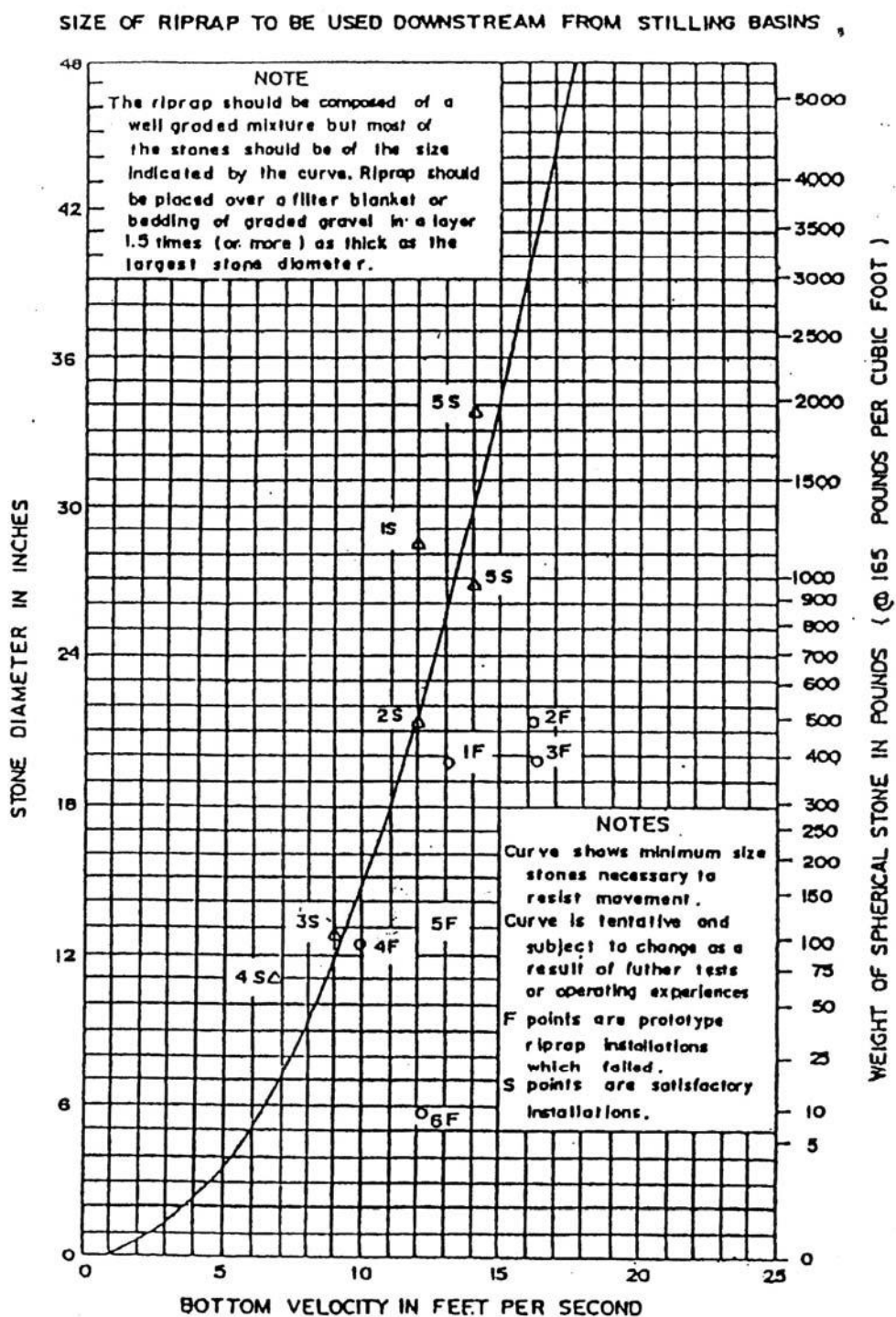
รูปที่ 4-17 โฉมออกแบบขนาดหินที่ต้านทานการกัดเซาะในบริเวณท้องน้ำ ที่มา U.S.B.R.(1963), "Hydraulic of Stilling Basins and Energy Dissipators", Denver
