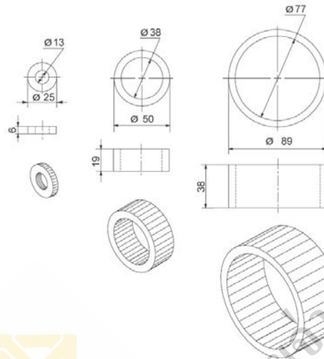
รูปที่ 11 เกจทดสอบขนาดต่างกัน 3 แบบ (ข้อ 9.2.1.1)
