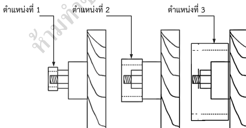
รูปที่ 12 ตำแหน่งการทดสอบปลายที่ยื่นล้าของสลักเกลียวและแป้นเกลียว (ข้อ 9.2.2)
