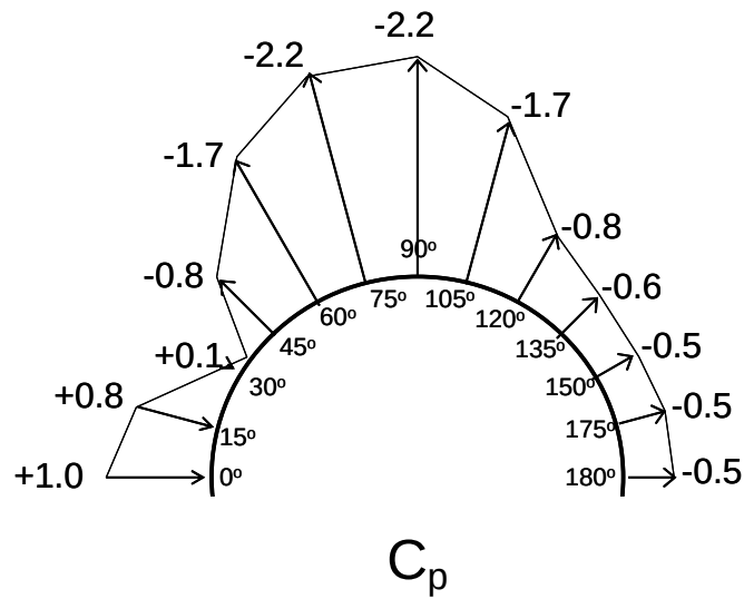
รูปที่ ๓.๖.๒ สัมประสิทธิ์ของหน่วยแรงลม ( C_p ) สำหรับโครงสร้างของปล่องควันตัวอย่าง
