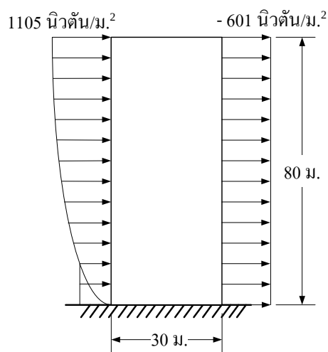
รูปที่ ต.2.2 หน่วยแรงลมสถิตเทียบเท่าด้านด้นลมและท้ายลม
