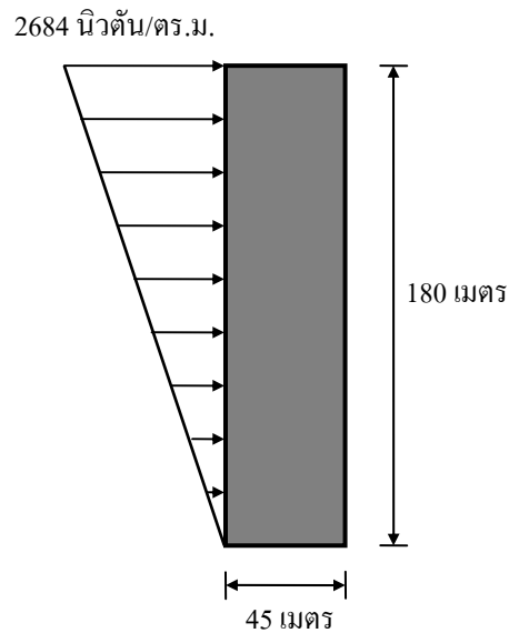
รูปที่ ค.3.5 แรงลมสถิตเทียบเท่าในทิศตั้งฉากกับแนวลม เมื่อลมกระทำในทิศทาง xx
