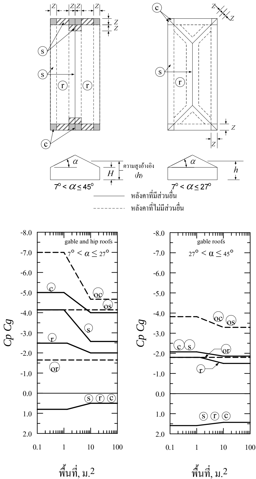
รูปที่ ข.5 ค่าสัมประสิทธิ์ของหน่วยแรงลมสูงสุดที่กระทำภายนอกอาคาร ( C_p C_g ) ที่กระทำกับหลังคาที่มีความชันมากกว่า 7^\circ สำหรับการออกแบบหลังคาและชิ้นส่วนของโครงสร้างรอง (secondary structural members)
