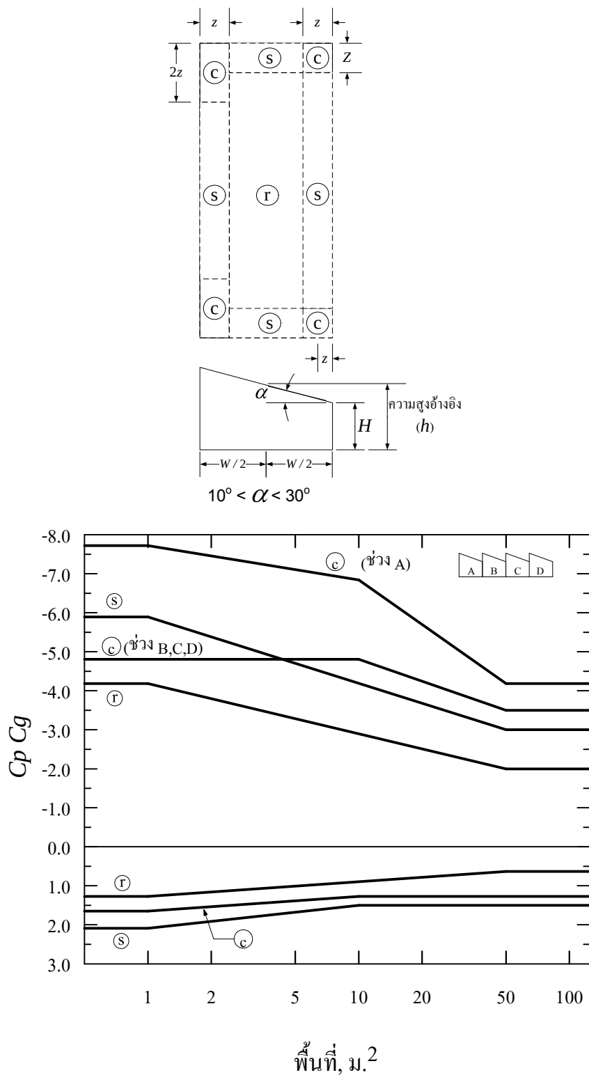
รูปที่ ข.8 ค่าสัมประสิทธิ์ของหน่วยแรงลมสูงสุดที่กระทำภายนอกอาคาร ( C_p C_g ) ที่กระทำกับหลังคาลักษณะพื้นเอียง (มีความลาดชันเพียงด้านเดียว และมีความต่อเนื่องมากกว่า 1 ช่วง) ที่มีความชันมากกว่า 10^\circ สำหรับการออกแบบหลังคาและชิ้นส่วนของโครงสร้างรอง (secondary structural members)
