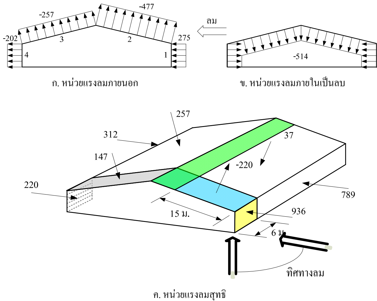
รูปที่ ต.1.4 ค่าหน่วยแรงลมสุทธิ (นิวตัน/ม. 2 ) ที่กระทำกับพื้นผิวโซนต่างๆ ของอาคารตัวอย่าง เมื่อ ทิศทางลมโดยทั่วไปอยู่ในแนวตั้งฉากกับสันหลังคา และหน่วยแรงลมภายในมีค่าเป็นลบ
