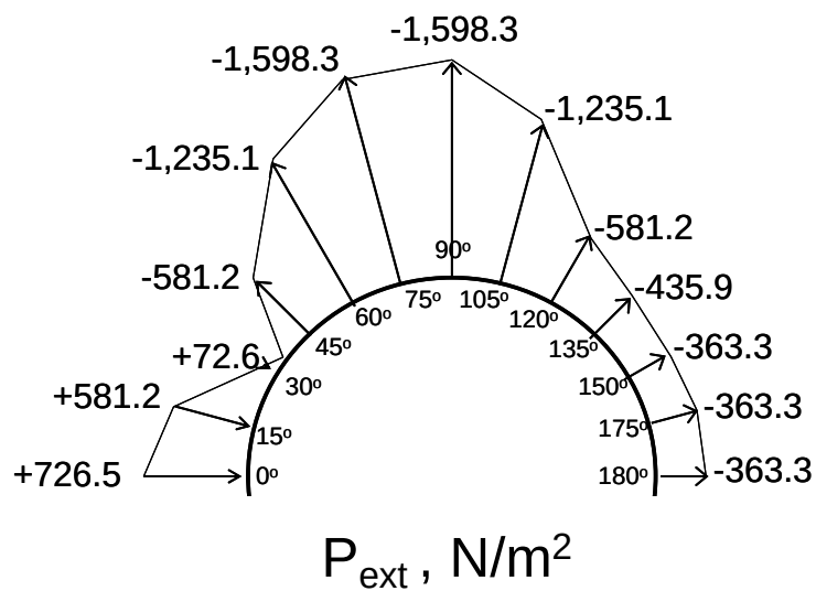
รูปที่ ๓.๖.๓ หน่วยแรงลมภายนอกที่กระทำกับผนังของปล่องควัน ณ ตำแหน่งต่างๆ
