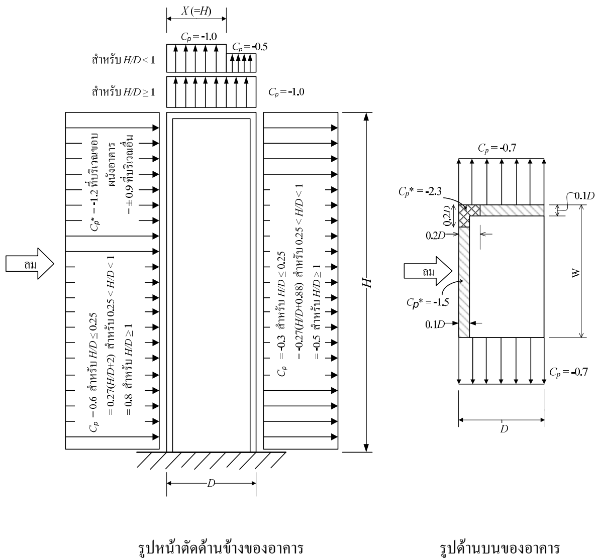
รูปที่ ข.9 ค่าสัมประสิทธิ์ของหน่วยแรงลม ( C_p และ C_p^* ) สำหรับอาคารที่มีความสูงมากกว่าความกว้าง และมีหลังคาอยู่ในแนวราบ
