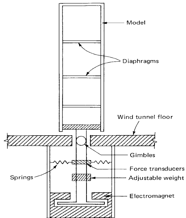
รูปที่ อ.5.4 แบบจำลองยึดหยุ่นของอาคาร
