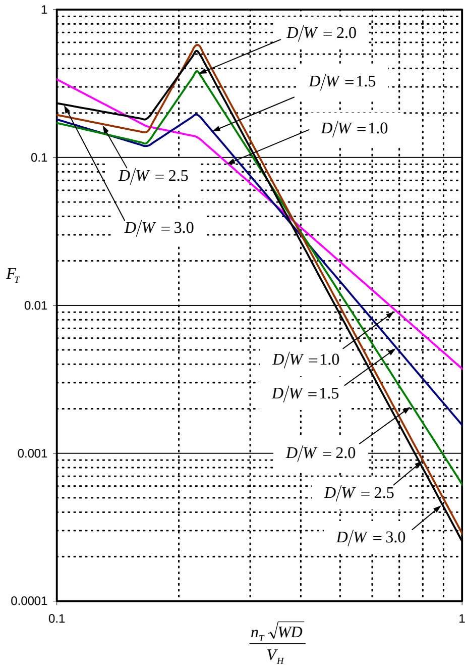
รูปที่ 4.7 สเปกตรัมของแรงลมในแนวนิดของอาคาร สำหรับ D/W = 1.0, 1.5, 2.0, 2.5 และ 3.0
