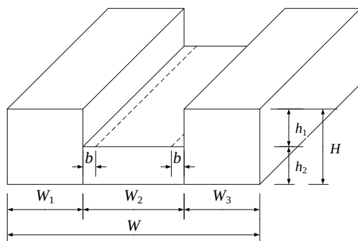
รูปที่ ข.4 ค่าสัมประสิทธิ์ของหน่วยแรงลมสูงสุดที่กระทำภายนอกอาคาร ( C_p C_g ) ที่กระทำบนหลังคาลดระดับ (stepped roof) โดยใช้ประกอบกับรูปที่ ข.3 สำหรับการออกแบบหลังคาและชิ้นส่วนของโครงสร้างรอง (secondary structural members)
