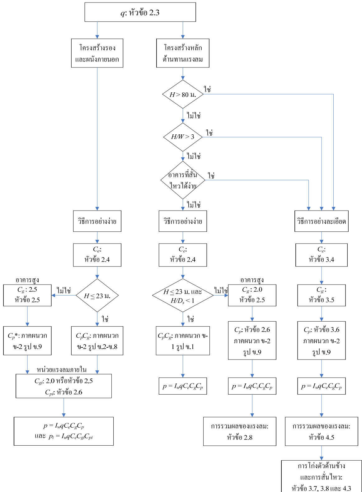
รูปที่ อ.2.1 แผนภาพขั้นตอนการคำนวณแรงลมและการตอบสนองโดยวิธีการอย่างง่ายและวิธีการอย่างละเอียด
