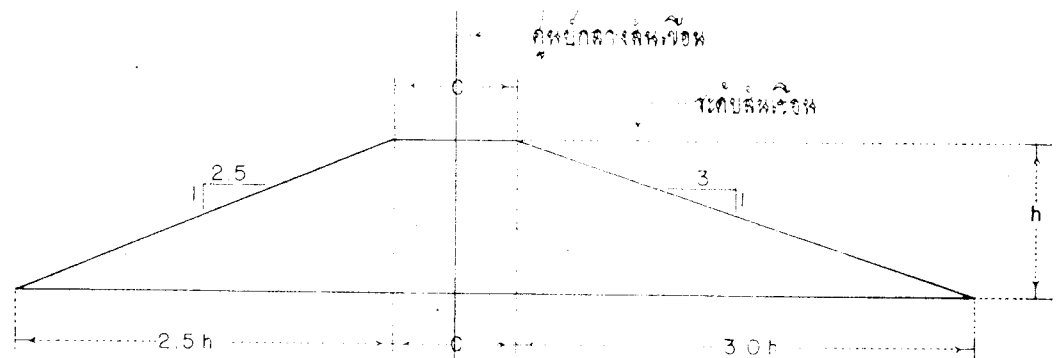
(ข) รูปทศมาทรราชของตัวเขื่อน
