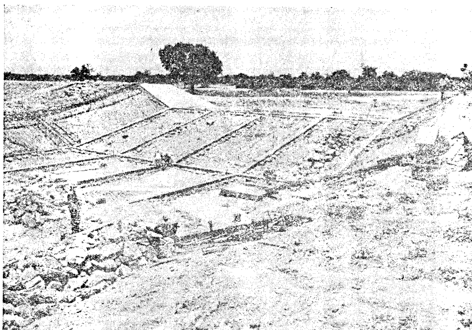
รูปที่ 10.2 งานก่อสร้างทางระบายน้ำดินแบบรางเท
