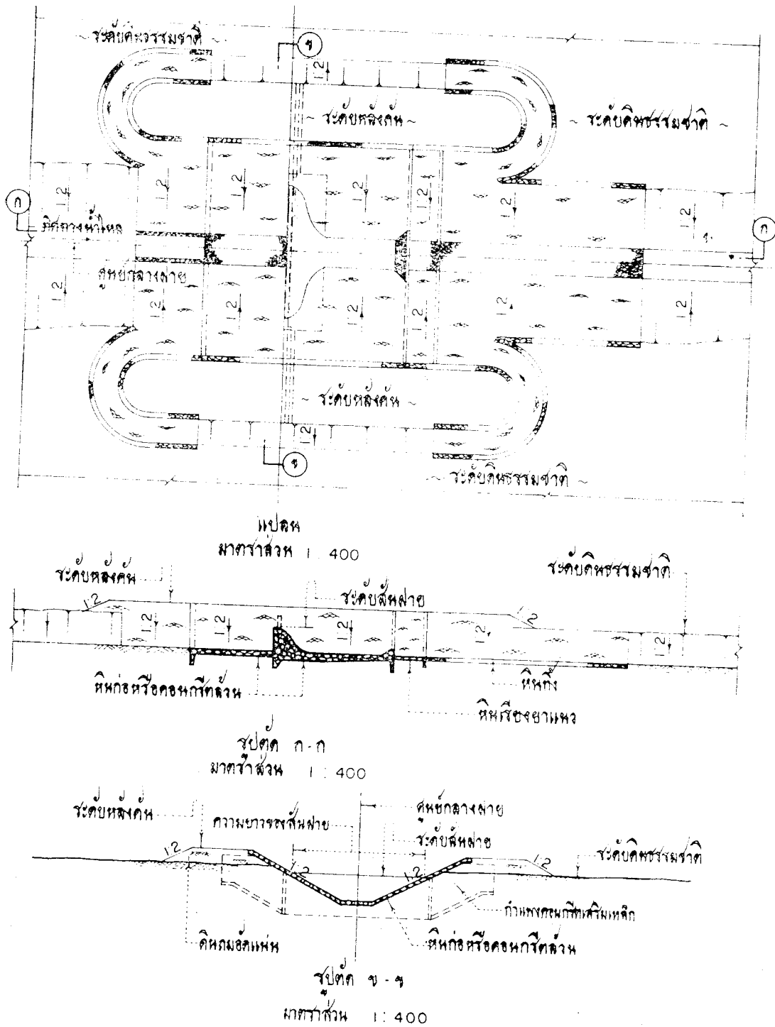
รูปที่ 8.10 แบบมาตรฐานของฝ่ายคอนกรีต
