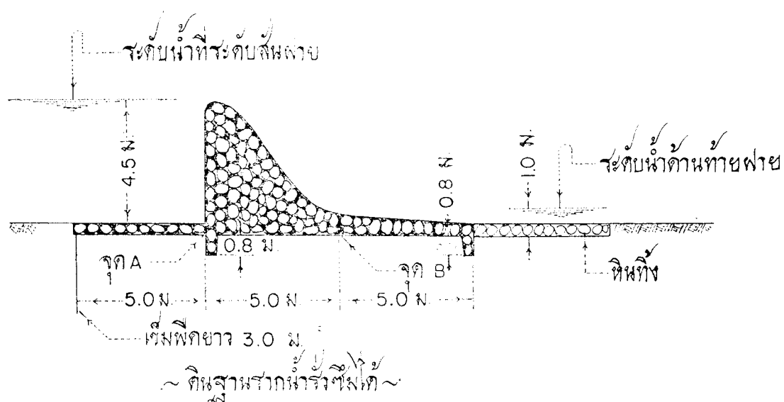
รูปที่ 8.7 รูปแสดงการคำนวณหาความเหมาะสมของฝายที่สร้างบนดินฐานรากตามทฤษฎีของ Lane
