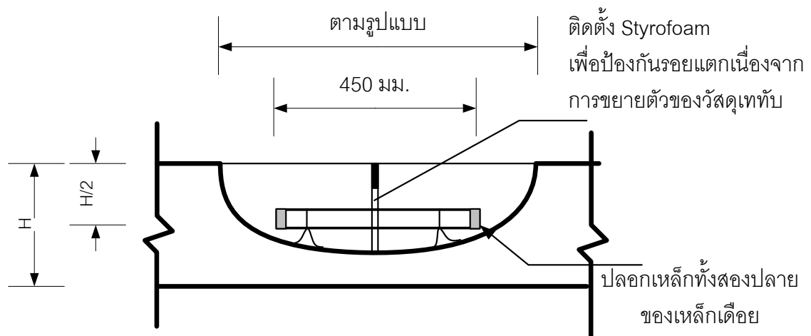
รูปที่ 3.4.4 รูปแบบติดตั้งเหล็กเดือย เพื่อเพิ่มการถ่ายน้ำหนัก
