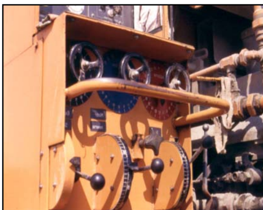
รูปที่ 2.4.2 อุปกรณ์วัดของเครื่องจักร Slurry Seal Machine
