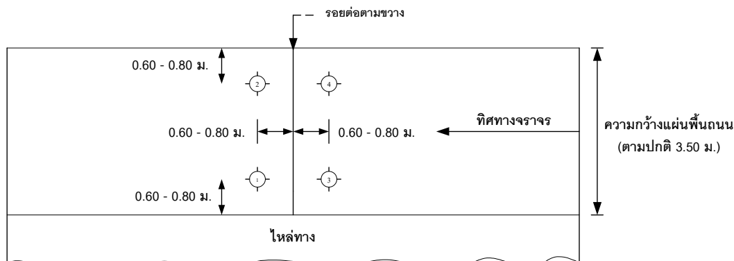
รูปที่ 3.6.2 กรณีที่เสียหายทั้งสองด้าน ให้เจาะ 4 รู บริเวณรอยต่อตามขวาง โดยเจาะทั้งสองข้างๆ ละ 2 รู
