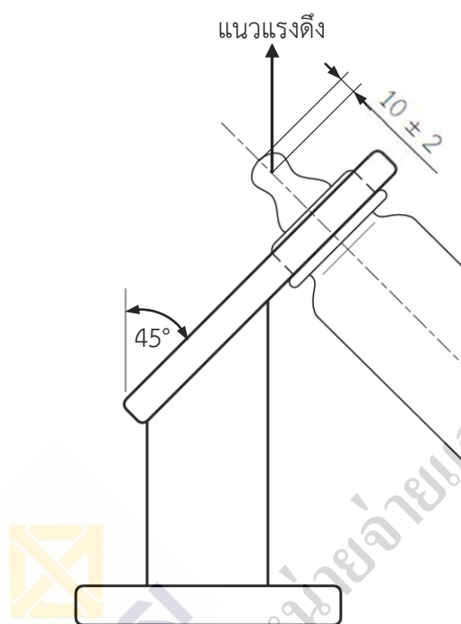
รูปที่ 4 การทดสอบการยึดแน่นกับขวตนม (ข้อ 8.3.3)
