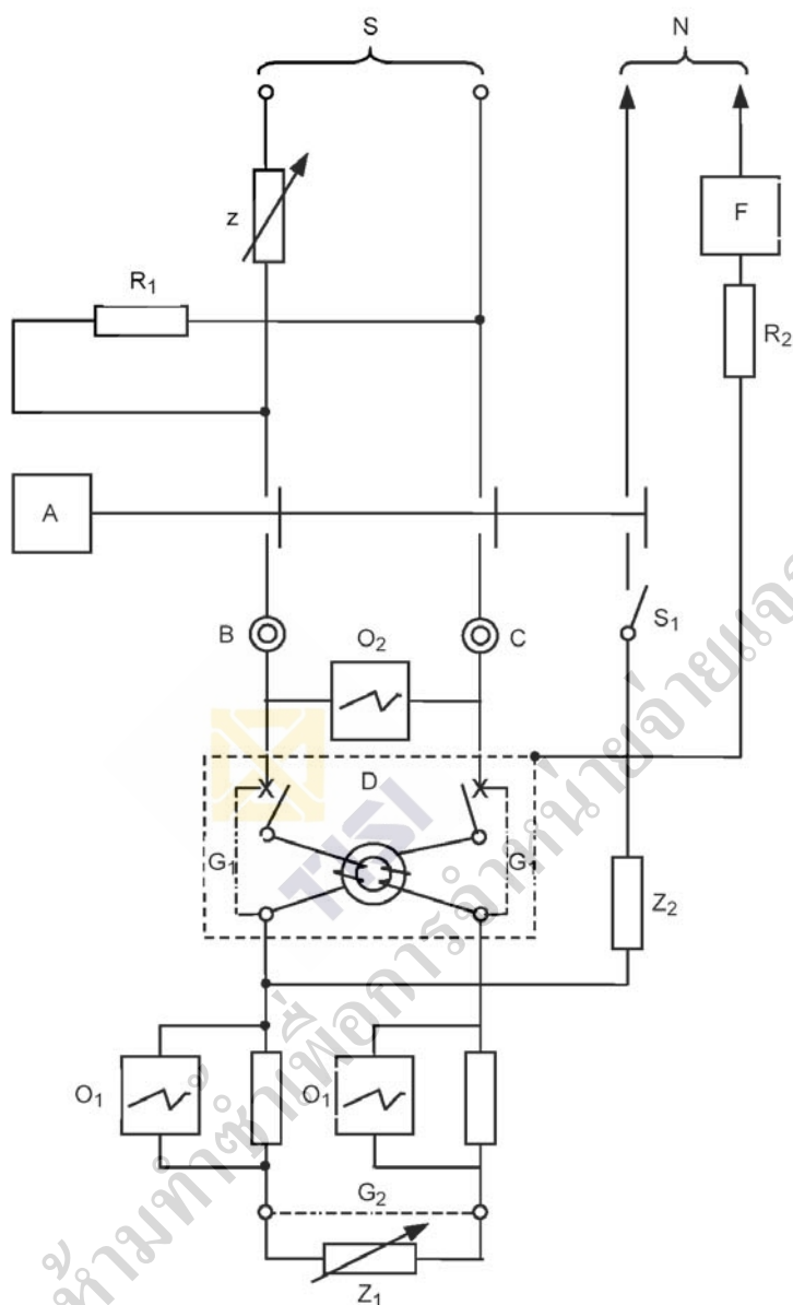
รูปที่ 6 วงจรทดสอบการทวนสอบความทนกระแสไฟฟ้าลัดวงจรที่กำหนด ของ RCBO แบบ 2 ขั้ว ในกรณีของวงจรเฟสเดียว (ข้อ 9.12)
