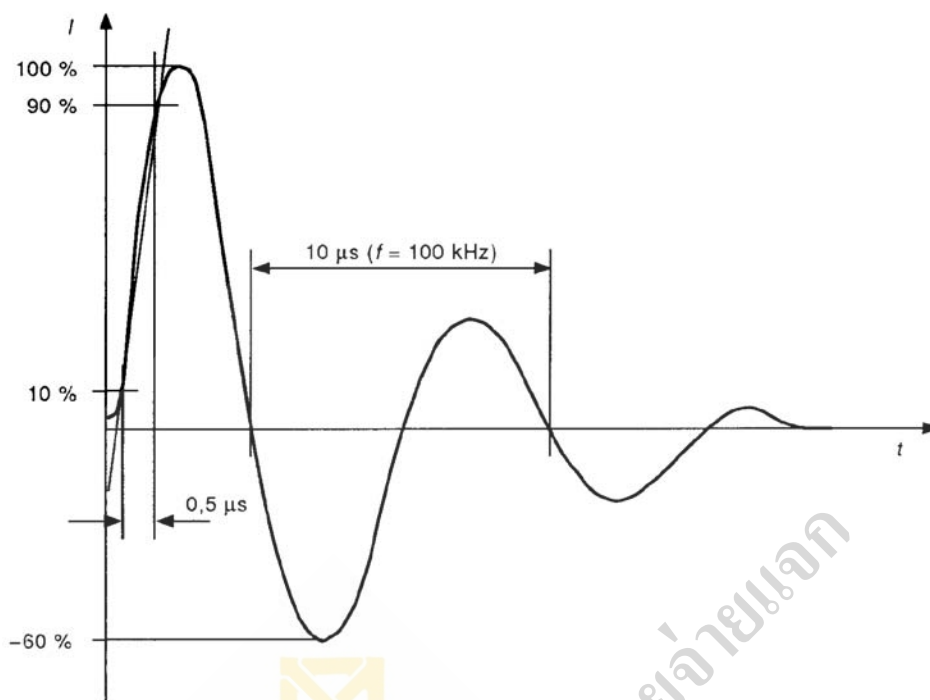
รูปที่ 23 คลื่นกระแสไฟฟ้าแกว่งหน่วง 0.5 ไมโครวินาที/100 กิโลเฮิร์ตซ์ (ข้อ 9.19.1)
