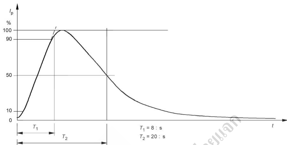
รูปที่ 25 อิมพัลส์กระแสเล็กร 8/20 ไมโครวินาที (ข้อ 9.19.2.1)
