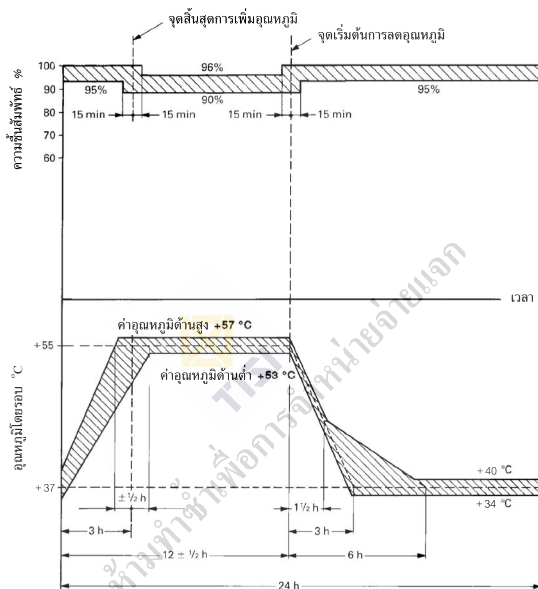
รูปที่ 21 วัฏจักรการทดสอบความชื้นได้ (ข้อ 9.22.1.3)
