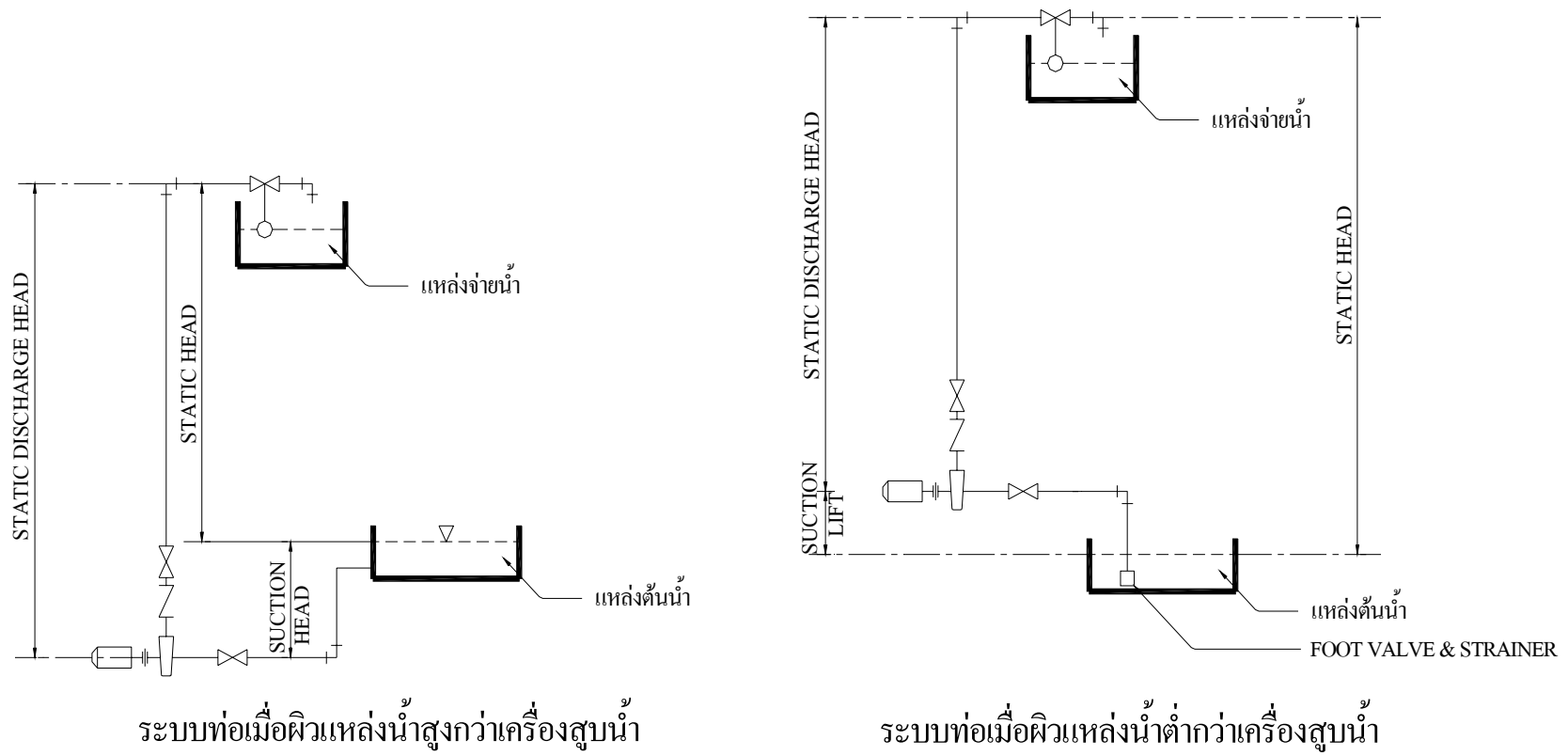
รูปที่ 2.3 แสดงรูปแบบอย่างง่ายของเครื่องสูบน้ำ และแรงดัน (Head) ต่าง ๆ
