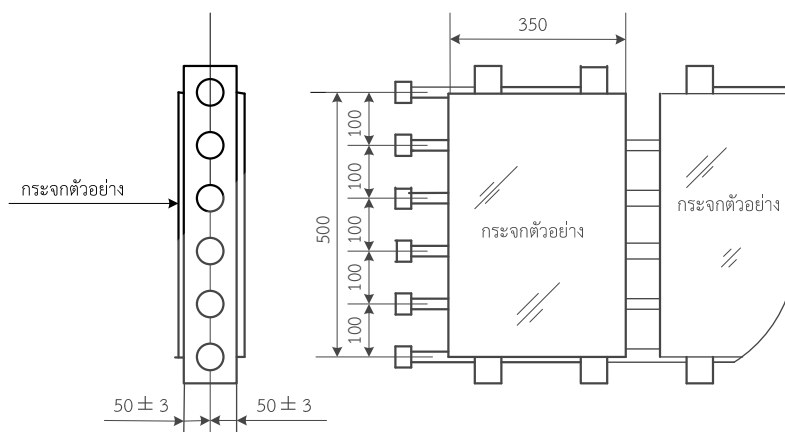
รูปที่ 7 ตัวอย่างแผงหลอดอัลตราไวโอเล็ตและการติดตั้งตัวอย่าง
