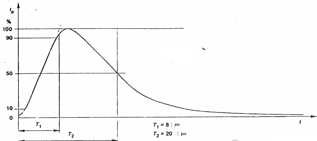
รูปที่ 23 อิมพัลส์ของกระแสเสิร์จ 8/20 ไมโครวินาที
