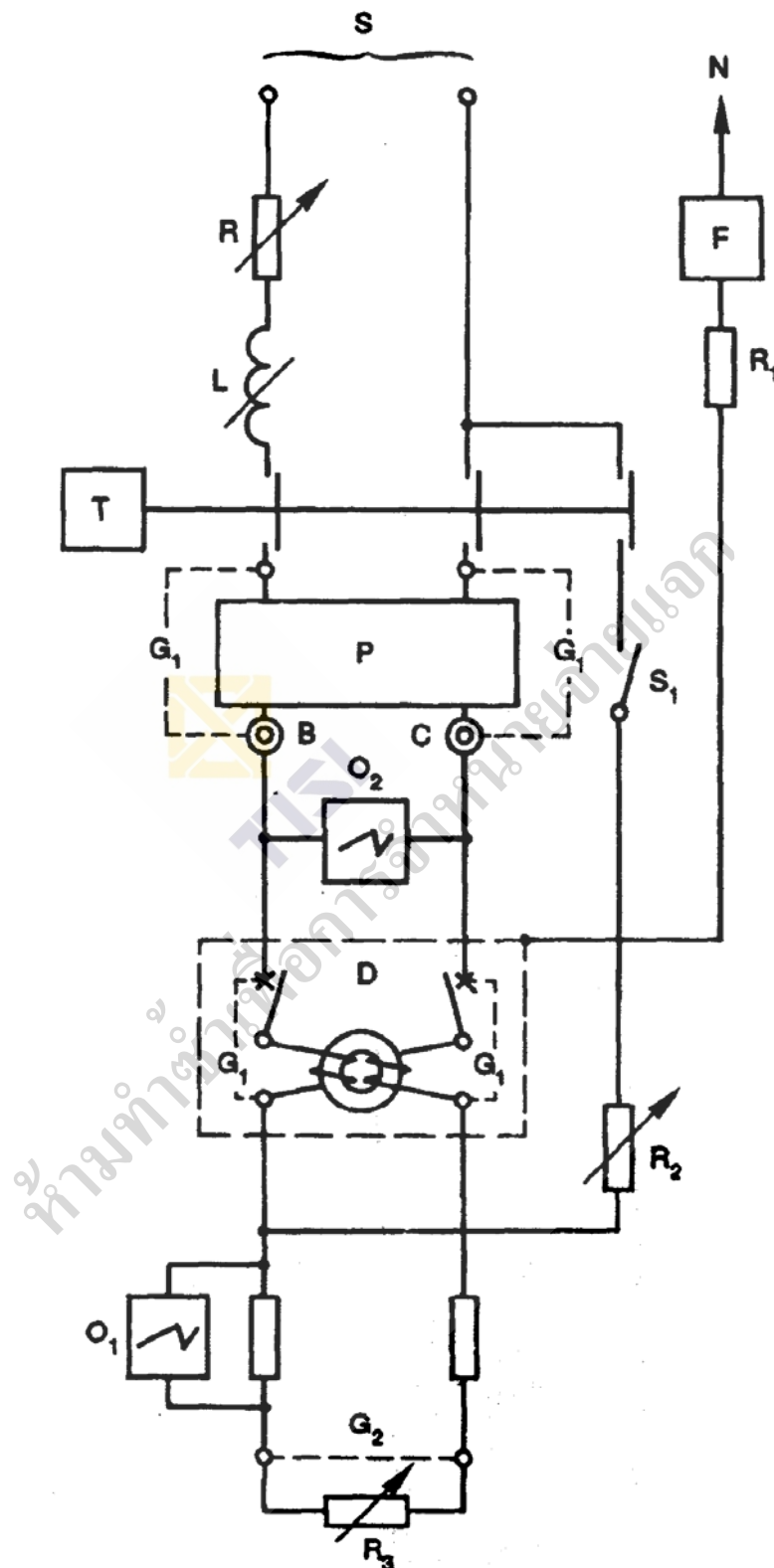
รูปที่ 6 วงจรทดสอบการทวนสอบวิสัยความสามารถต่อการตัดวงจรที่กำหนด และการประสาน SCPD ของ RCCB แบบ 2 ขั้ว กับวงจร 1 เฟส (ข้อ 9.11)
