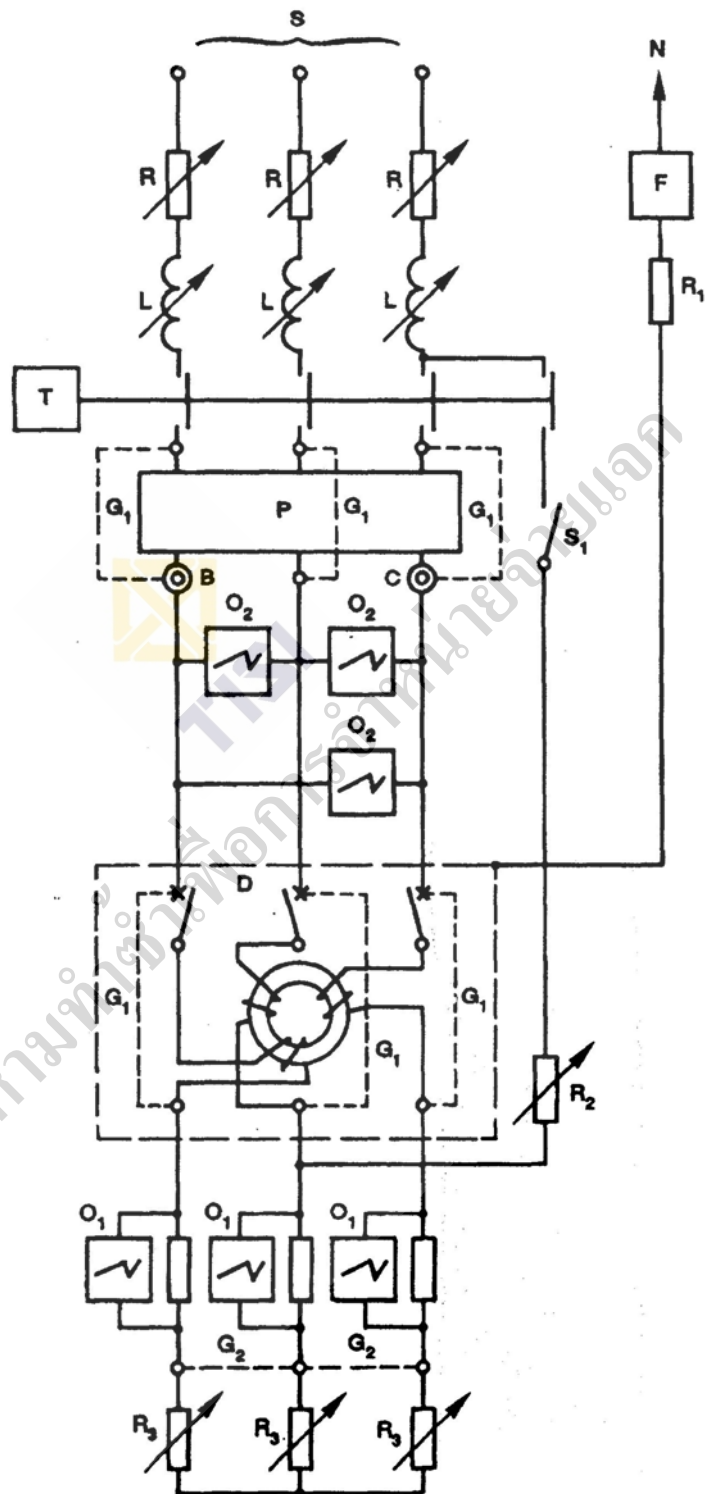
รูปที่ 7 วงจรทดสอบการทนสอบวิธีความสามารถต่อการตัดวงจรที่กำหนด และการประสาน SCPD ของ RCCB แบบ 3 ขั้ว กับวงจร 3 เฟส (ข้อ 9.11)
