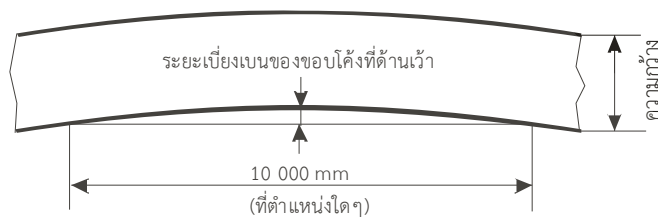
รูปที่ 2 การวัดระยะเบี่ยงเบนของขอบโค้งที่ด้านเว้าของเหล็กแผ่นหนา/แผ่นบางขอบตัด (ข้อ 7.6)
