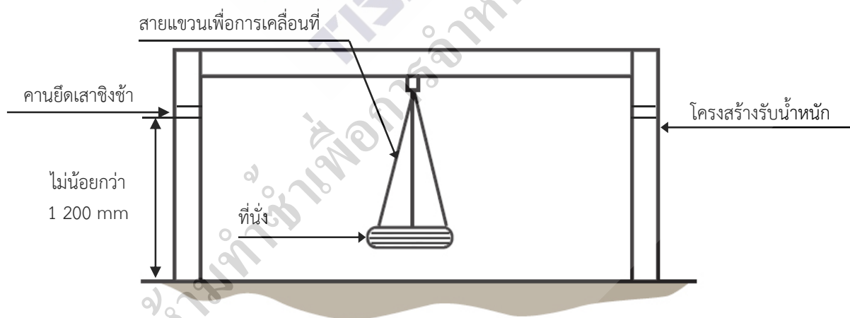
รูปที่ 2 ตัวอย่างชิงช้าหมุนรอบ (ข้อ 2.4)
