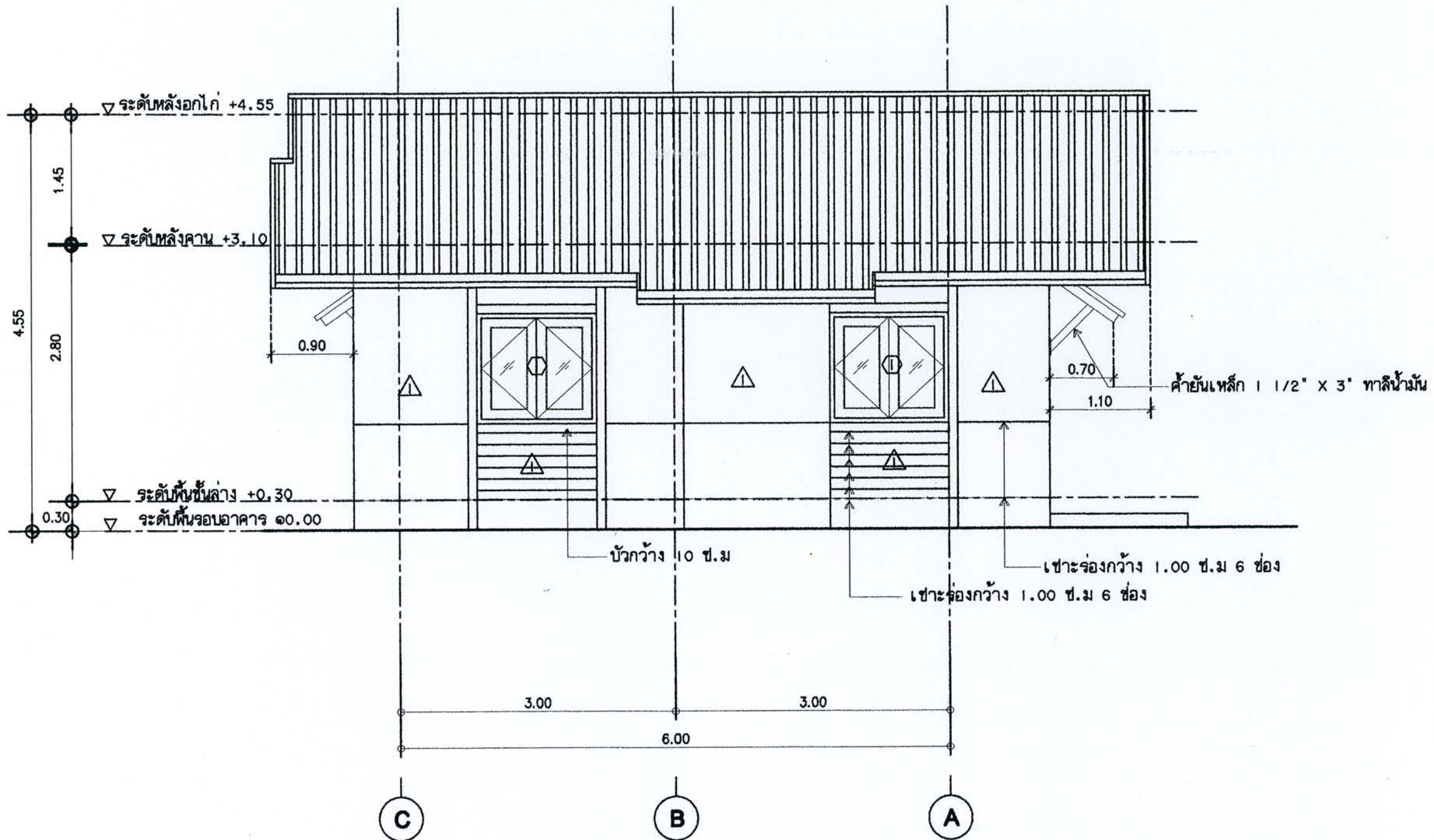
รูปด้าน 2 SCALE 1:50
