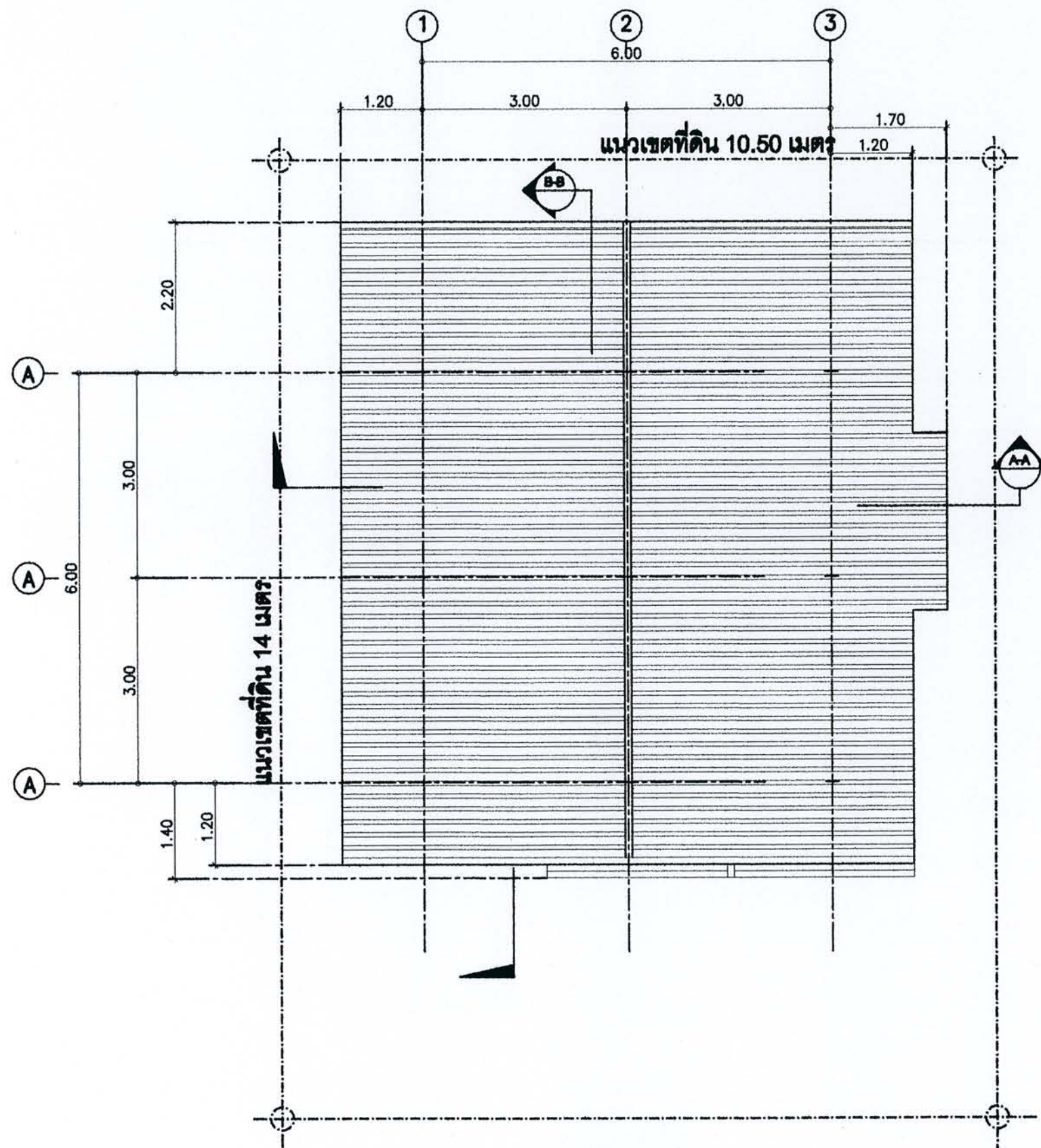
แปลนหลังคา SCALE 1:75
