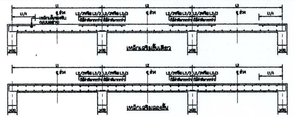
แบบมาตรฐานแสดงการเสริมเหล็กตามยาวในคานที่มีจุดรองรับโดยเสา
