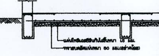
แบบมาตรฐานแบบขยาย
