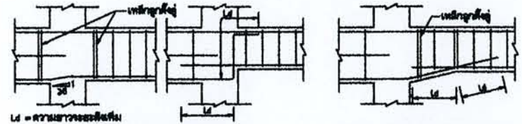
การวางเหล็กเสริมคานให้ต่อเนื่อง
