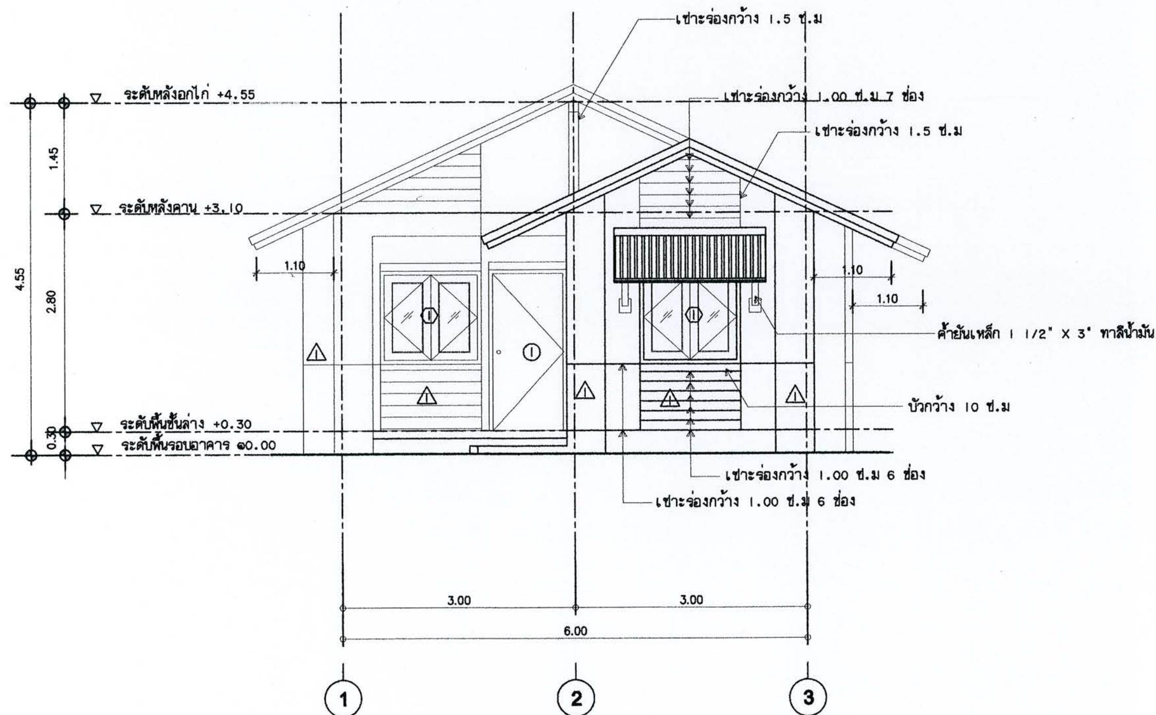
รูปด้าน 1 SCALE 1:50
