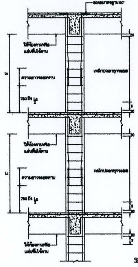
แบบมาตรฐานแบบขยาย
