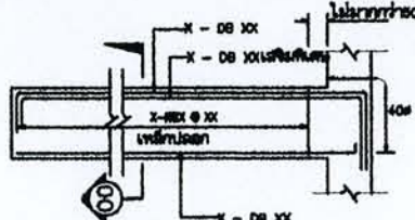
แบบมาตรฐานแสดงการเสริมเหล็กในคานยื่น แบบที่ (1)
