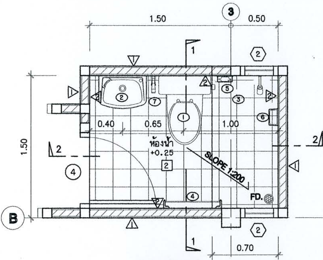
แปลนห้องน้ำ มาตราส่วน 1:25
