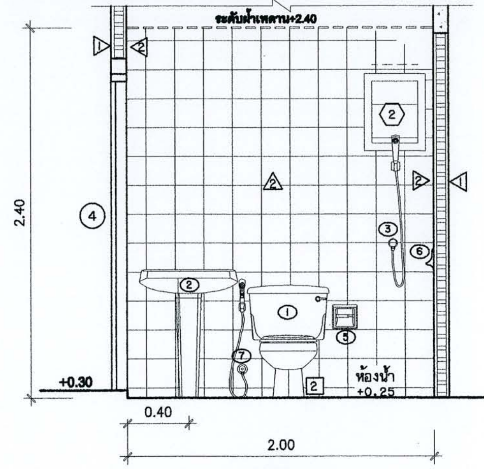
รูปตัด 2-2 มาตราส่วน 1:25
