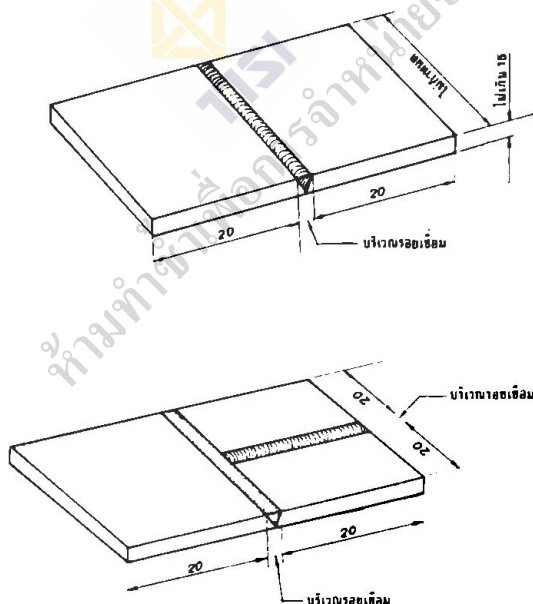
รูปที่ ก.1 ลักษณะของรอยเชื่อม (ข้อ ก.1.2)
