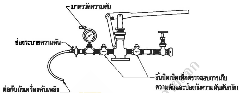
รูปที่ ก.1 เครื่องอัดไฮดรอลิก (ข้อ ก.1.1)
