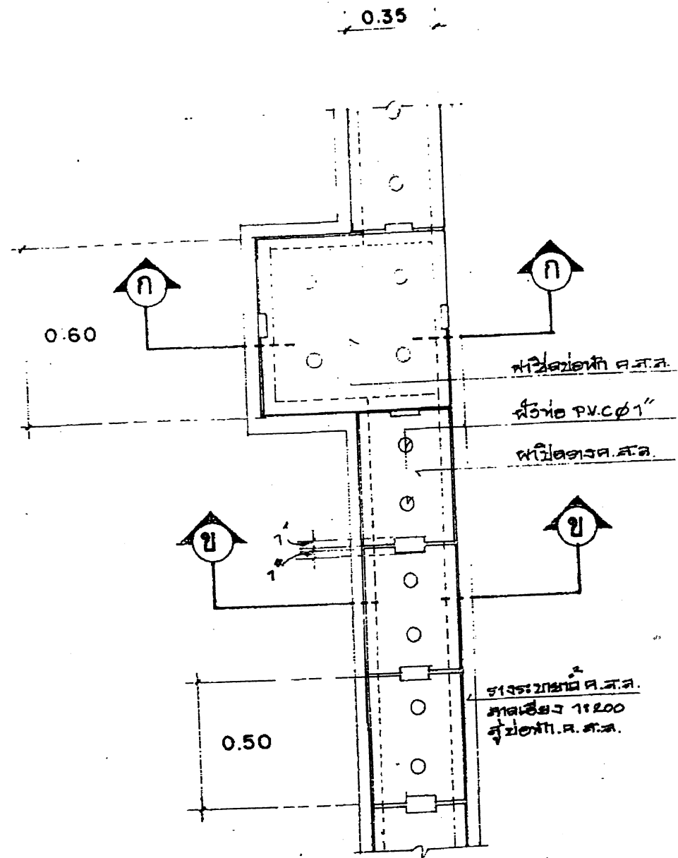
แปลนร่างระบายน้ำเปิด 1:20
