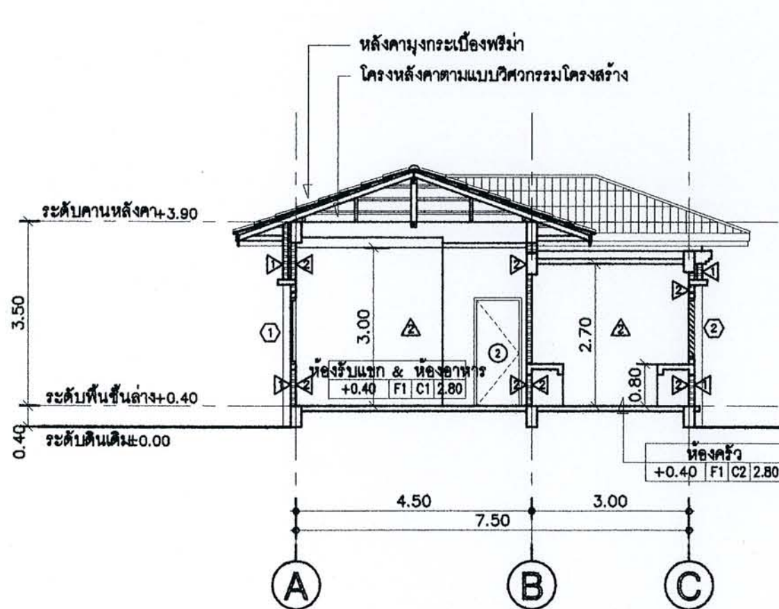
รูปตัด A ขนาด 1:100
