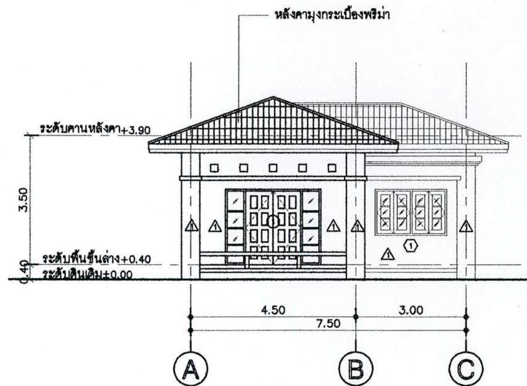
รูปด้าน 1 ขนาด 1:100
