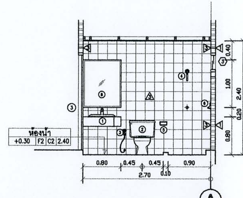
รูปตัด 2 มาตราส่วน 1:50
