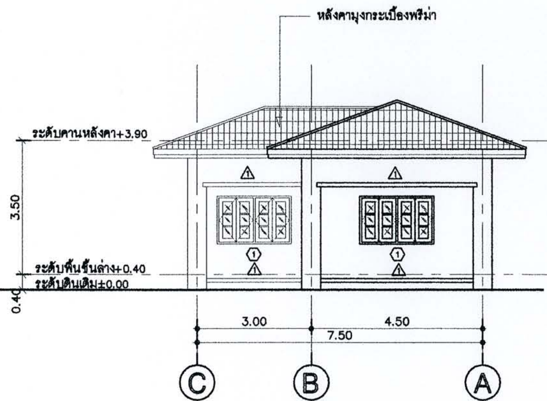
รูปด้าน 3 ขนาดย่อ 1:100
