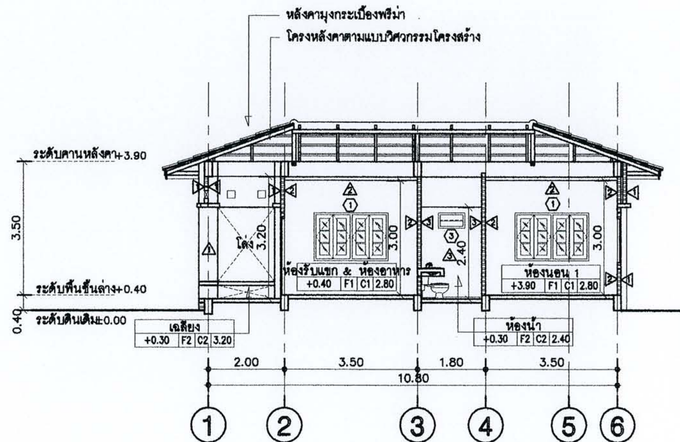
รูปตัด B ขนาด 1:100
