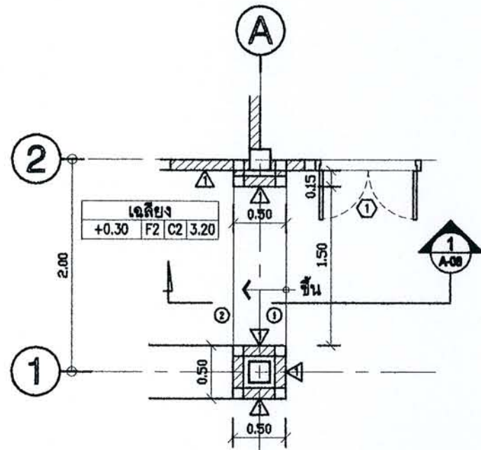
แปลนขยาย ST-1 มาตราส่วน 1:50
