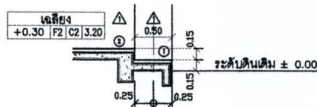
รูปตัด 1 มาตราส่วน 1:50
