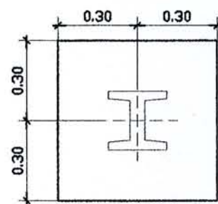
PLAN F1 scale 1:20
