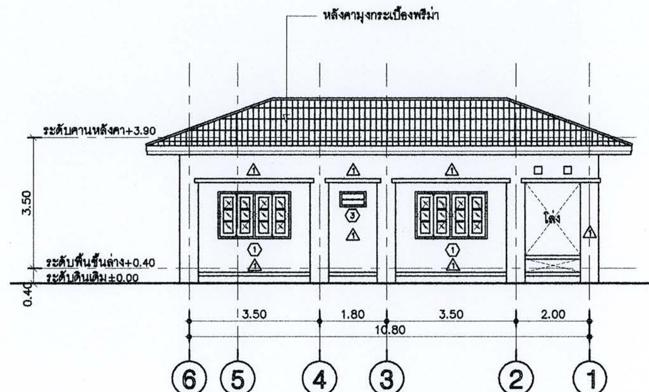
รูปด้าน 4 ขนาดย่อ 1:100
