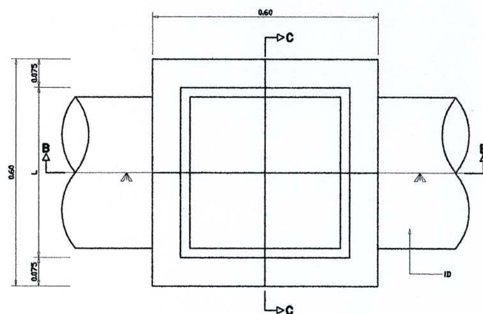
แบบขยายบ่อพักสำเร็จรูปมาตรฐาน มาตราส่วน 1:10
