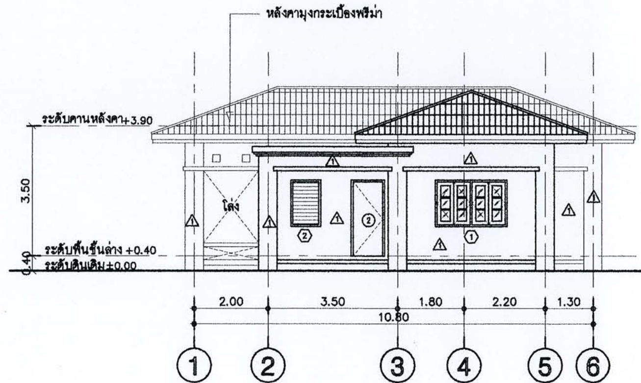
รูปด้าน 2 ขนาด 1:100
