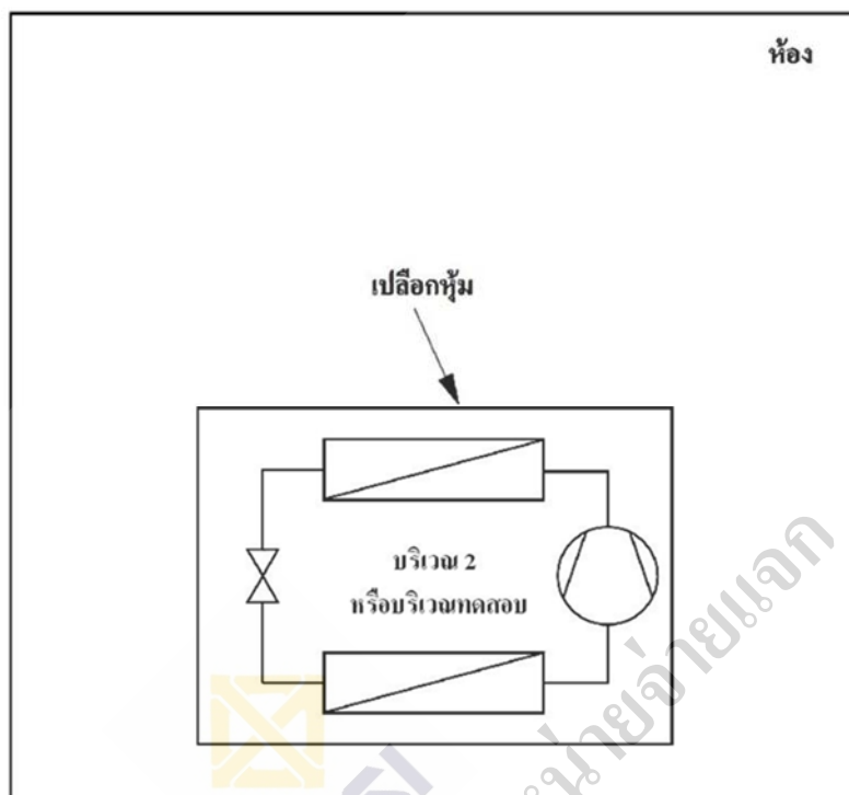
รูปที่ ชช. 1 พื้นที่ไม่มีภาระระบายอากาศ
