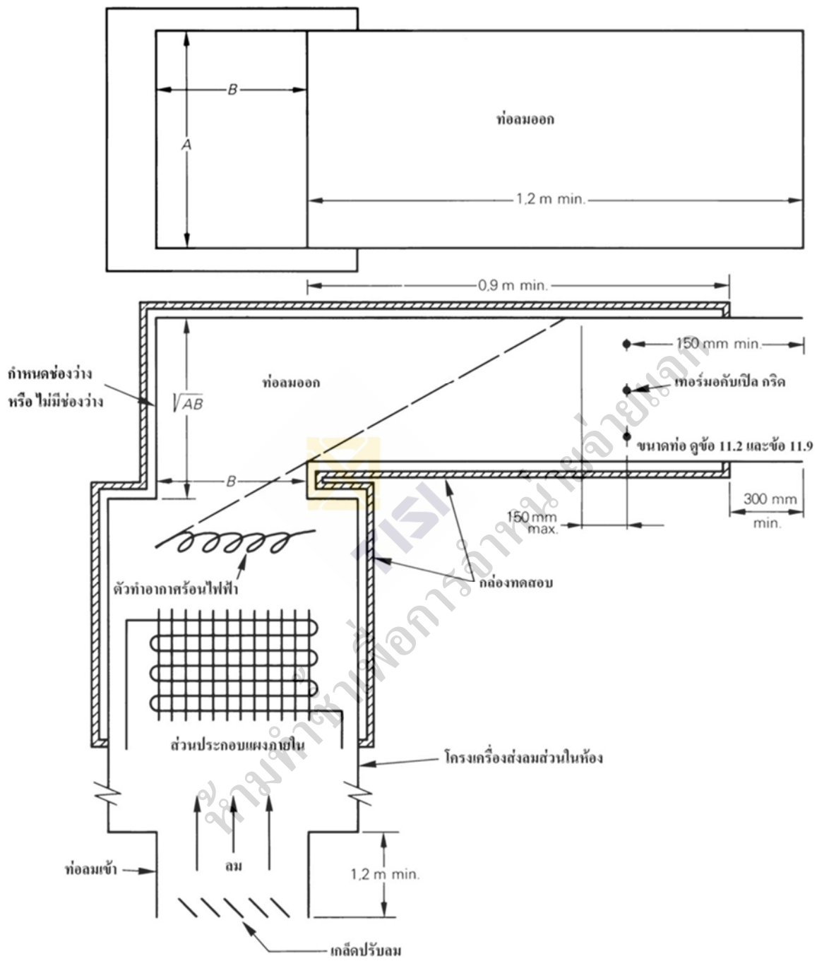
รูปที่ 101 ก) การประยุกต์ใช้ กรณีลมไหลขึ้น (upflow)
