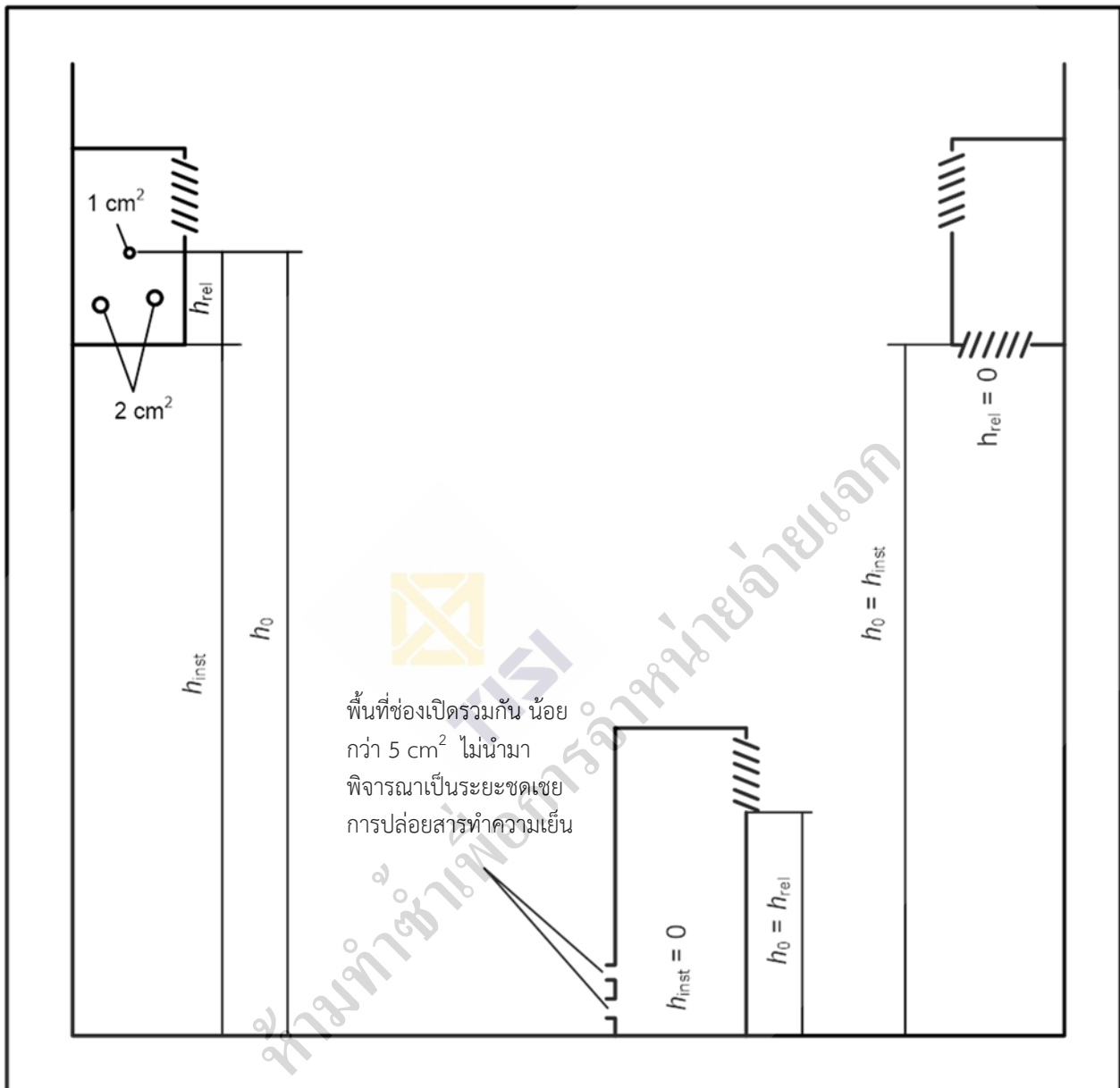
รูปที่ ขช.3 ค่าความสูงของ h_{\text{inst}} , h_0 และ h_{\text{rel}} สำหรับใช้ในการคำนวณค่า A_{\text{min}} และ m_{\text{max}}
