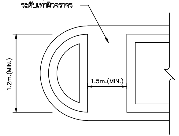
แปลนลาดทางเท้า (TYPE D)
