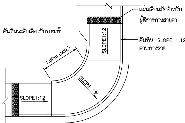
แปลนลาดทางเท้า (TYPE G)
