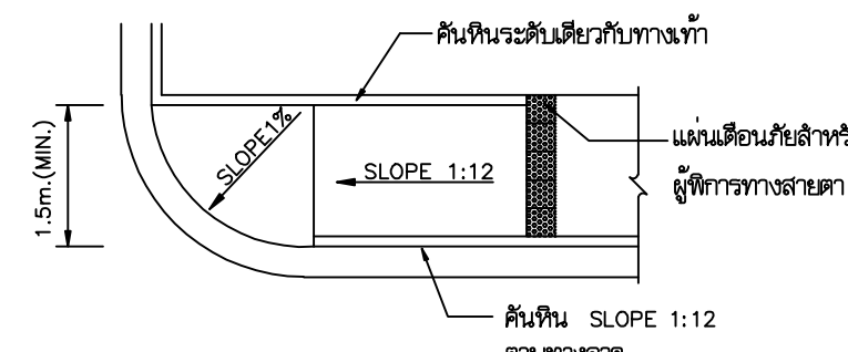
แปลนลาดทางเท้า (TYPE C)
