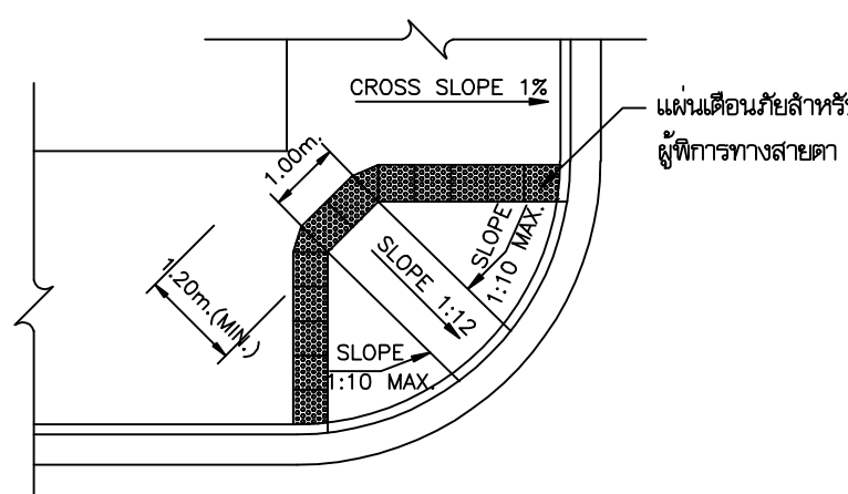
แปลนลาดทางเท้า (TYPE F)
