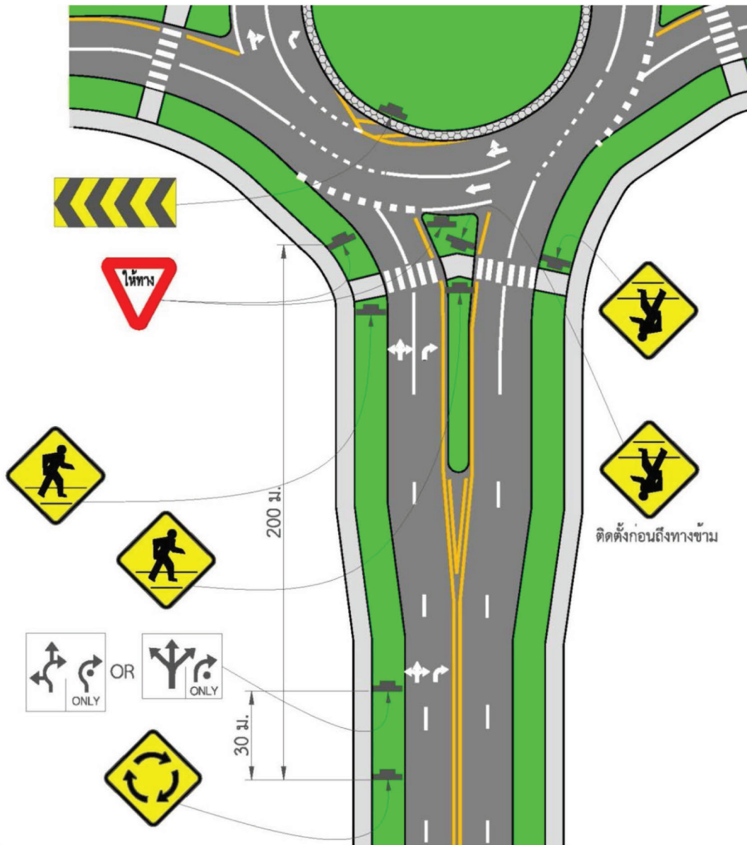
รูปที่ M7b-3 การติดตั้งป้ายจราจรสำหรับวงเวียนขนาดใหญ่
