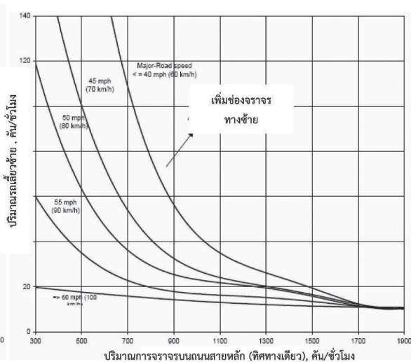
ข) แนวทางการจัดทำช่องเฉพาะสำหรับรถเลี้ยวซ้าย บริเวณทางแยก ถนน 4 ช่องจราจร
