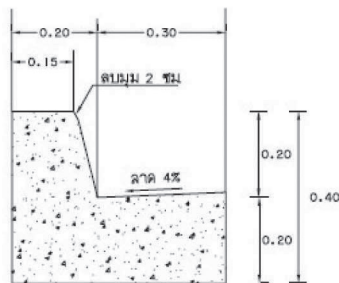
รูปที่ M2b-4 คันหินรูปแบบที่ 1 คันหินทั่วไปและรางต้น
