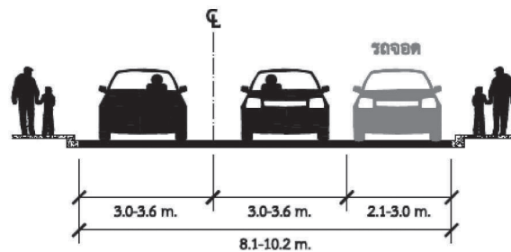
รูปที่ P1b - 9 ความกว้างของถนนสายรองแบบมีช่องจราจรจอด 1 ข้าง
