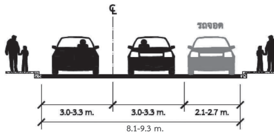
รูปที่ P1b - 12 ความกว้างของถนนท้องถิ่นแบบมีช่องจราจรจอด 1 ข้าง
