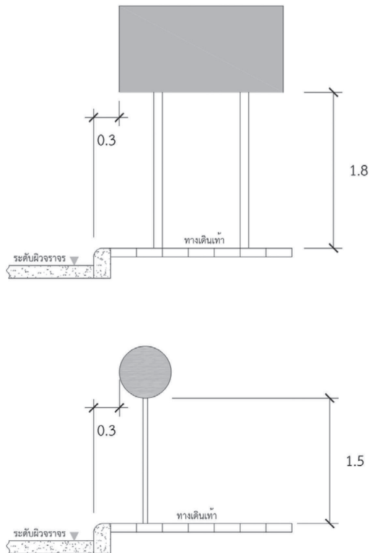
รูปที่ M1a-3 การติดตั้งป้ายจราจรและป้ายแนะนำบนทางเท้า
