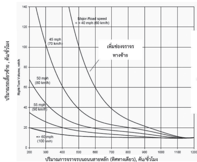
ก) แนวทางการจัดทำช่องเฉพาะสำหรับรถเลี้ยวซ้าย บริเวณทางแยก ถนน 2 ช่องจราจร
