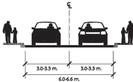
รูปที่ P1b - 11 ความกว้างของถนนท้องถิ่นแบบไม่มีช่องจราจรจอด
