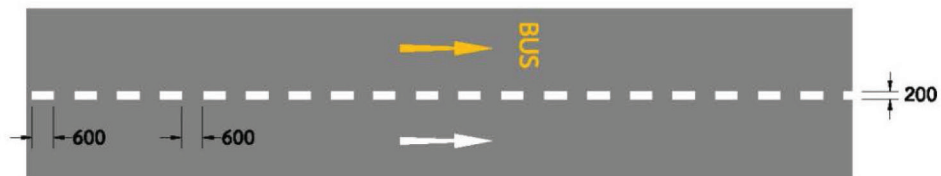
รูปที่ S2c-4 มาตรฐานเส้นแบ่งช่องจราจร
