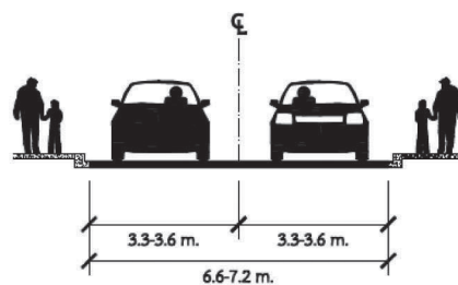
รูปที่ S2e-4 ความกว้างของถนนสายหลักแบบไม่มีช่องจราจรจอด
