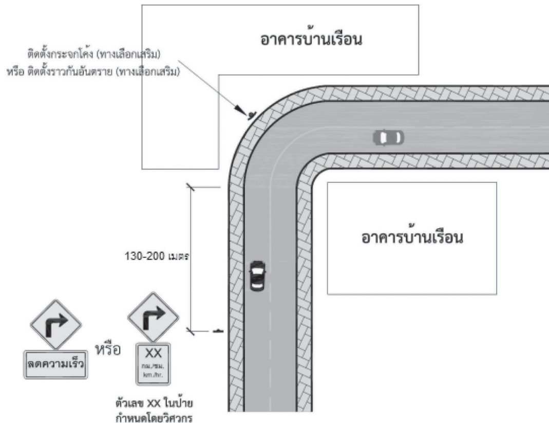
รูปที่ P3a - 3 ตัวอย่างการติดตั้งกระຈกโค้ง
