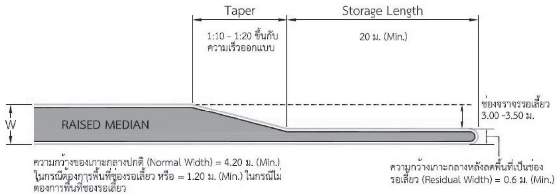
รูปที่ P7a - 4 แผนแสดงเกาะกลางแบบยก
