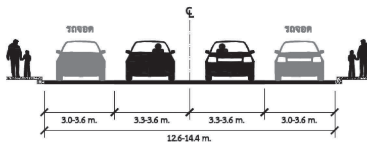
รูปที่ P1b - 7 ความกว้างของถนนสายหลักแบบมีช่องจราจรจอด 2 ข้าง
