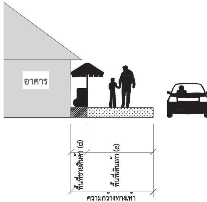
รูปที่ S2d-3 การออกแบบพื้นที่ทางเท้า : พื้นที่ขายสินค้าจัดขอบอาคาร
