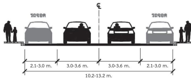
รูปที่ P1b - 10 ความกว้างของถนนสายหลักแบบมีช่องจราจรจอด 2 ข้าง
