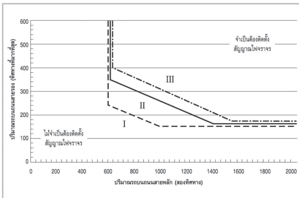
รูปที่ M5a-6 แสดงปริมาณจราจรบนถนนสายหลักและถนนสายรอง
