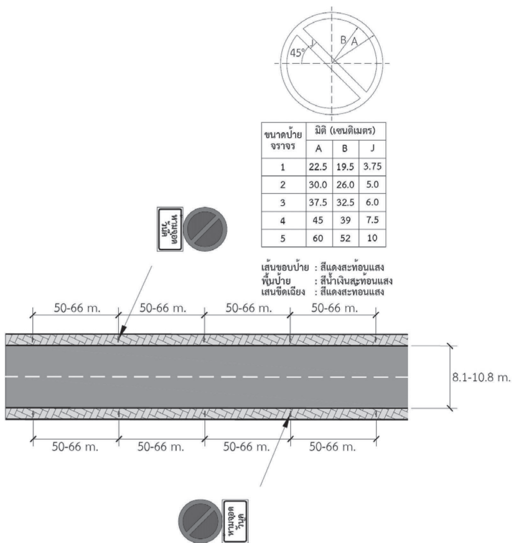
รูปที่ S2e-13 ขนาดของป้ายและระยะการติดตั้งป้ายวันคู่ วันคี่
