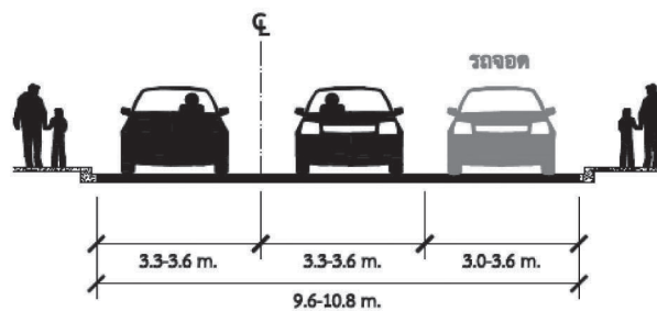
รูปที่ P1b - 6 ความกว้างของถนนสายหลักแบบมีช่องจราจรจอด 1 ข้าง
