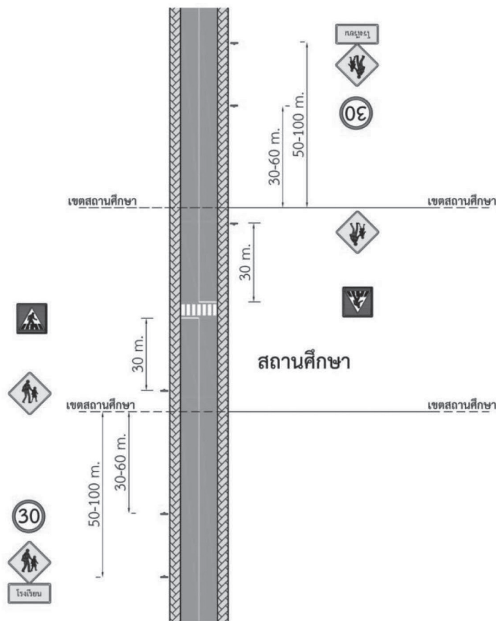
รูปที่ S1a-5 การติดตั้งป้ายและเครื่องหมายจราจรบริเวณทางเดินข้ามบริเวณด้านหน้าโรงเรียน บนซอยขนาดเล็ก
