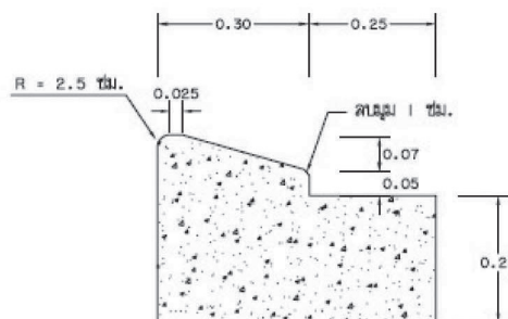
รูปที่ M2b-5 คันหินรูปแบบที่ 2 คันหินเตี้ยและรางต้น
