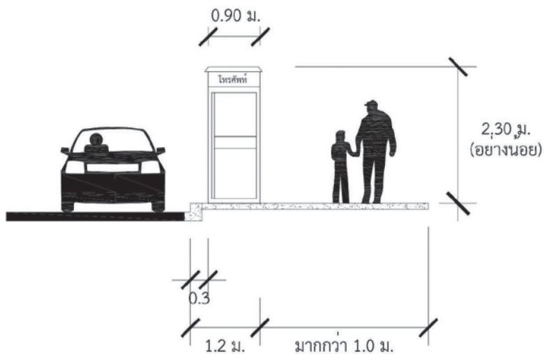
รูปที่ P4a - 5 การติดตั้งอุปกรณ์บนทางเท้า
