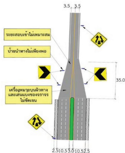
รูปที่ P1a - 1 ปัญหาการลดช่องจราจรอย่างกะทันหัน
