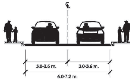
รูปที่ P1b - 8 ความกว้างของถนนสายรองแบบไม่มีช่องจราจรจอด
