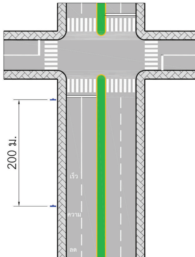
รูปที่ P4c - 5 การออกแบบทางม้าลายบริเวณทางแยก มีสัญญาณไฟจราจร
