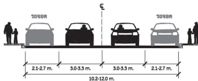
รูปที่ P1b - 13 ความกว้างของถนนท้องถิ่นแบบมีช่องจราจรจอด 2 ข้าง
