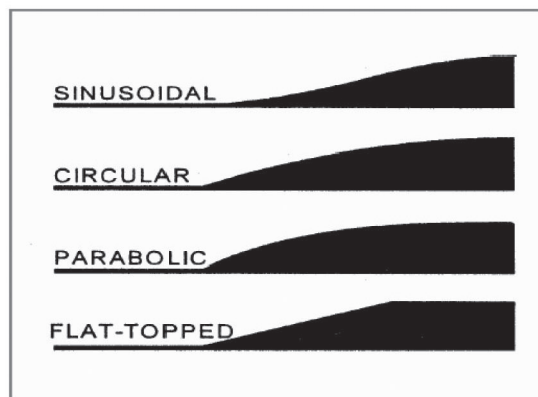
รูปที่ P3b - 5 แสดงภาพหน้าตัดแบบต่างๆของเส้นลดความเร็วของเส้นอุปกรณ์ speed hump
