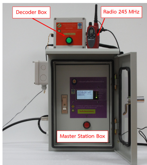
รูปที่ 5-4 กล่องถอดรหัสสัญญาณ (decoder box) ที่เชื่อมต่อกับเครื่องประมวลผลแม่ข่าย
