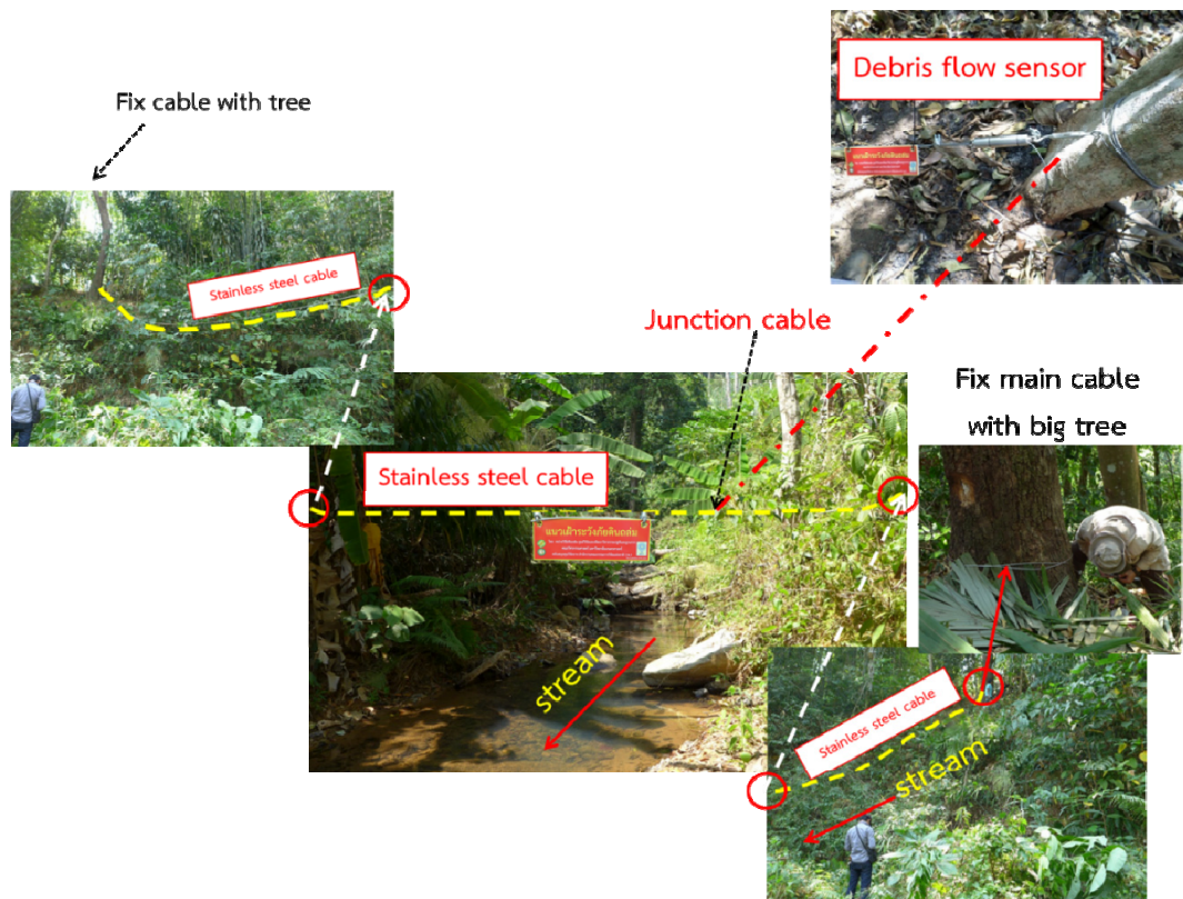
รูปที่ 5-6 ตัวอย่างขั้นตอนการติดตั้งเครื่องมือตรวจวัดการไหล (debris flow sensor) ในพื้นที่เสี่ยงภัยดินถล่มและน้ำป่าไหลหลาก
