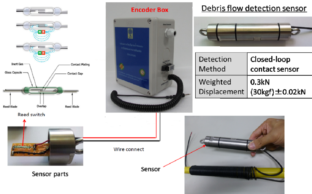
รูปที่ 3-3 อุปกรณ์ตรวจวัดการไหลดินถล่ม debris flow detector sensor
